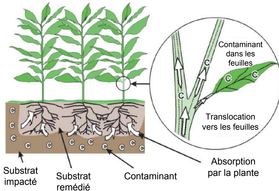
Figure I-4 : Principe de la phytoextraction. Ce schéma illustre l'assimilation des contaminants (C) contenus dans un substrat par les racines de la plante et le mouvement des contaminants des racines vers les parties aériennes de la plante.
