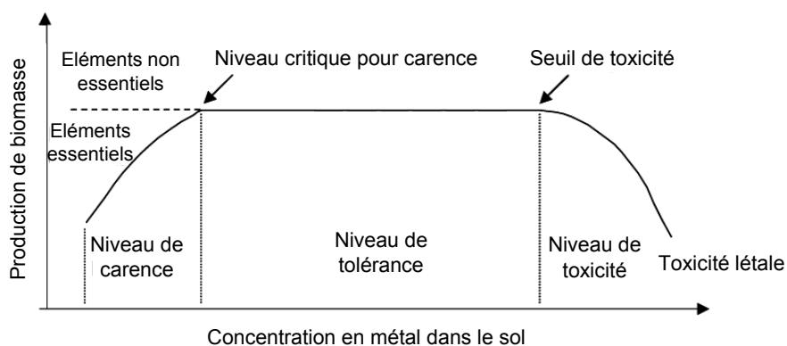
Figure I-14: Effets de la concentration en polluant métallique présent dans le sol sur la biomasse produite par les plantes (adapté de Baker & Brooks, 1989).
