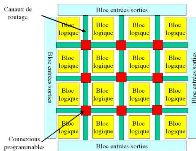
FIGURE 2.3 – Bloc diagramme d'un FPGA
