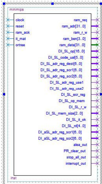
FIGURE 4.6 – Schéma bloc de l'ACU
