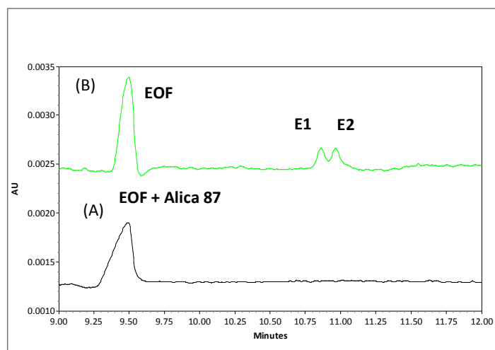
Figure 36 : Electrophérogramme de l'Alica 76, (A) en absence de NH 2 -β-CD, (B) en présence de 20 mM de NH 2 -β-CD, BGE 2, pH 7,4
