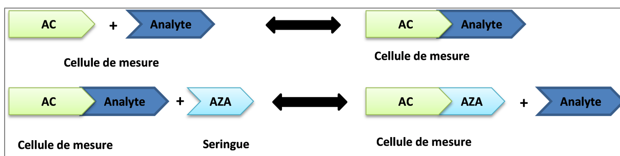
Figure 56 : Représentation schématique de la titration par compétition.
