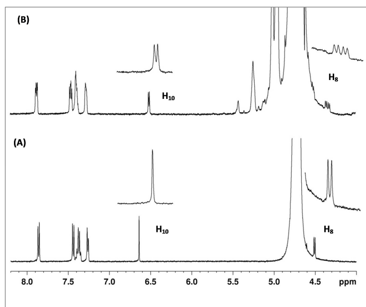
Figure 27 : Extrait des spectres ^1\text{H} de (A) l'Alica 87 seul (0,5 mM en Alica 87) et du (B) complexe \text{NH}_2 - \beta -CD/ Alica 87 (0,5 mM en Alica 87 et 3 mM \text{NH}_2 - \beta -CD), tampon phosphate deutéré pH 7,4 (67 mM) contenant 30% en DMSO d_6 .
