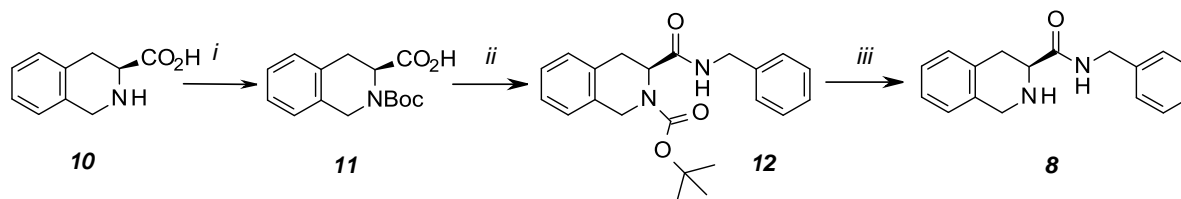
Schéma 3 : i) \text{Boc}_2\text{O} , \text{NaOH} , \text{THF} , \text{H}_2\text{O} ; 97%; ii) \text{Bn-NH}_2 , \text{HOBt} , \text{HBTU} , \text{DIEA} , \text{DCM} ; 90%; iii) \text{TFA} , \text{DCM} puis \text{Na}_2\text{CO}_3 aq., 94%.
