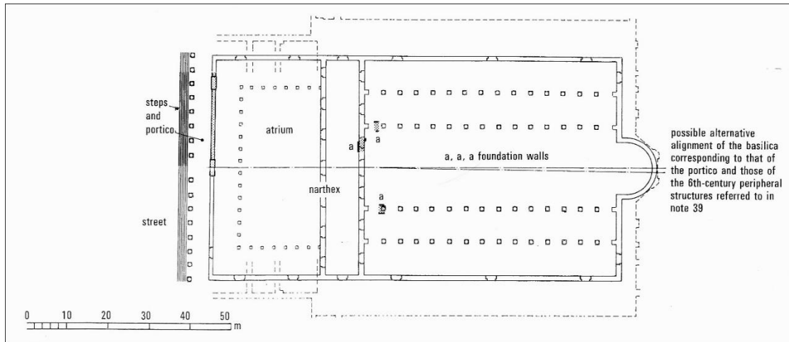
Fig. 66 : plan hypothétique de la Grande Église théodosienne, dans Mainstone, Hagia Sophia , p. 141 (fig. 165)
