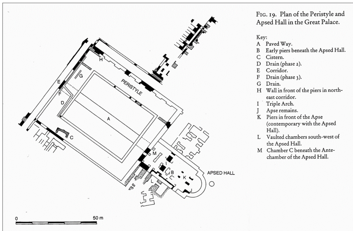
Fig. 40 : salle absidiée et péristyle, dans Bardill, Brickstamps , p. 137 (fig. 19)
