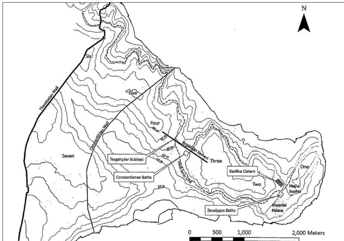
Fig. 157 : en pointillé, parcours hypothétique de l'aqueduc d'Hadrien, dans Ward-Crow-Crappier, Water-Supply Infrastructure , p. 184 (fig. 4)
