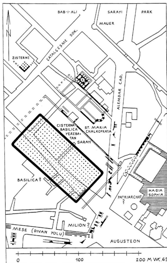
Fig. 148 : plan de la Citerne Basilique, avec les vestiges de la Basilique, dans Kleiss, Chalkopratenkirche , p. 150 (fig. 1)
