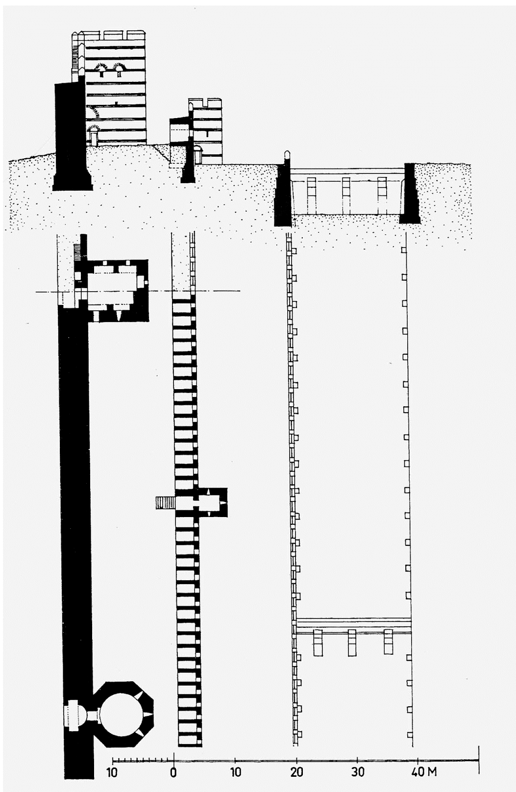
Fig. 109 : le système de défense d'est en ouest, dans Müller-Wiener, Bildlexicon , p. 287 (fig. 326)
