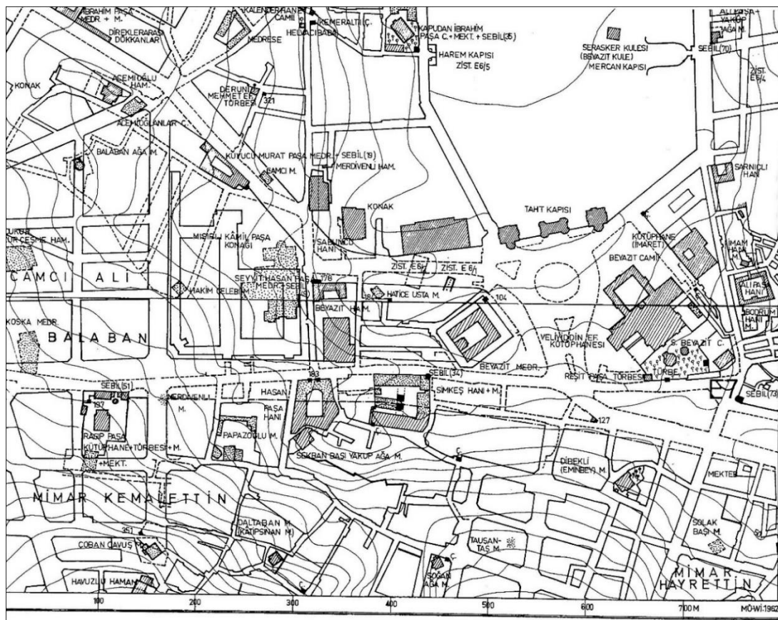
Fig. 78 : plan du secteur de Beyazıt, dans Müller-Wiener, Bildlexicon , p. 258 (fig. 290)
