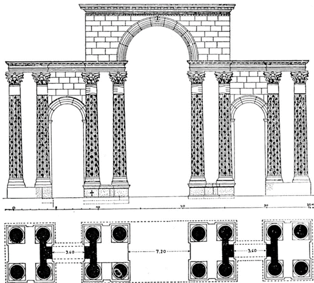
Fig. 83 : forum de Théodose I er : reconstitution hypothétique de l'arc, dans Naumann, Neue Beobachtungen , p. 128 (fig. 6)
