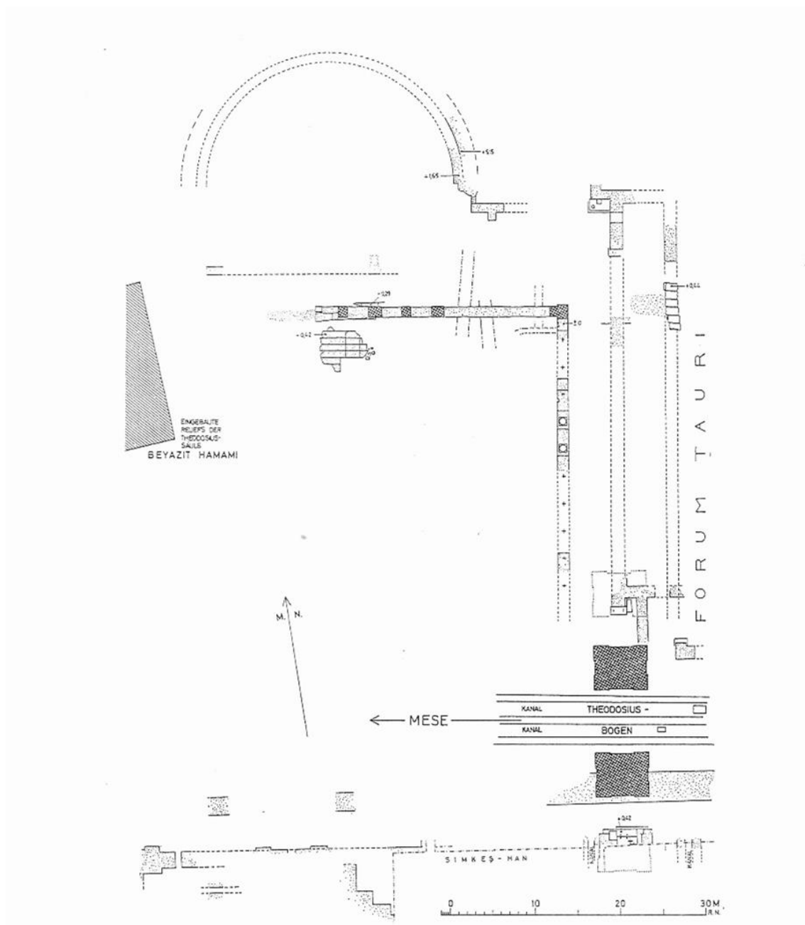
Fig. 84 : forum de Théodose I er : plan avec stylobate, dans Naumann, Neue Beobachtungen , p. 122 (fig. 5)
