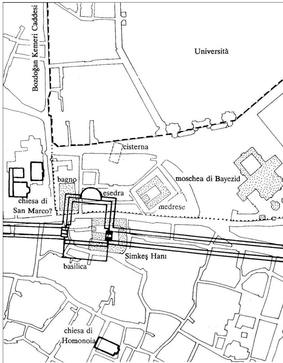
Fig. 85 : reconstitution hypothétique du forum de Théodose I er dans Berger, Tauros , p. 28 (fig. 1)
