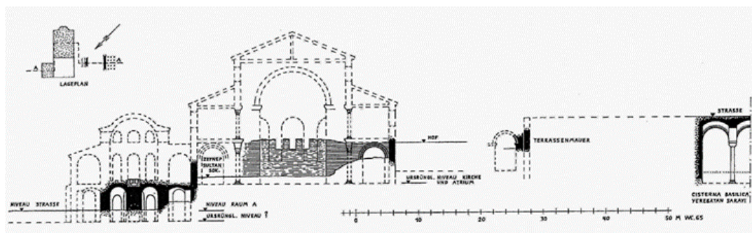
Fig. 71 : à gauche, la Théotokos des Chalkoprateia ; à droite, la Citerne Basilique, dans Kleiss, Chalkopratenkirche , 156 (fig. 4)
