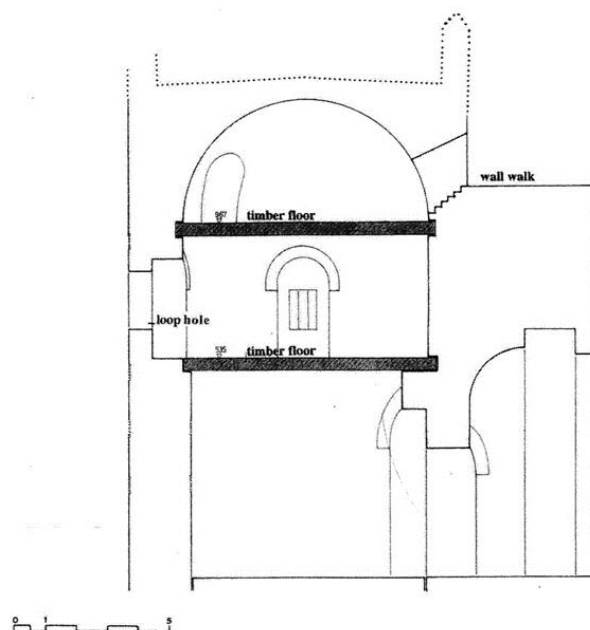
Fig. 111 : tour 2, dans Ahunbay-Ahunbay, Recent Work , fig. 9
