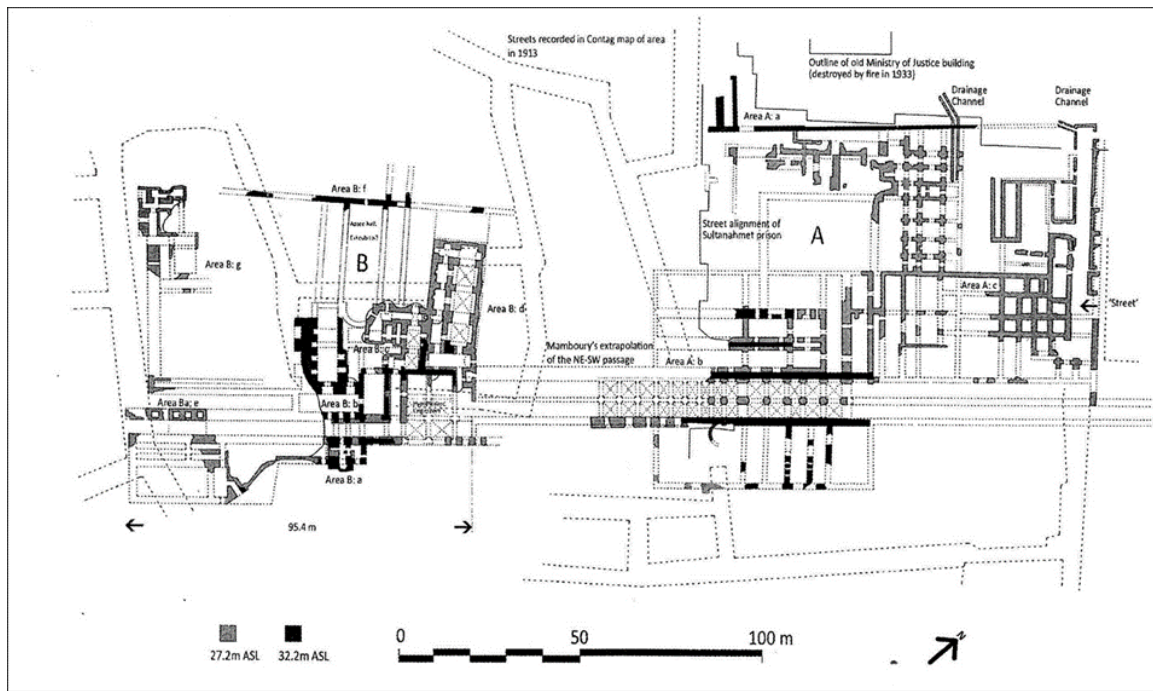
Fig. 34 : secteurs A et B, d'après Mamboury-Wiegand, Kaiserpaläste , revu par J. Macarlino, E. Lind, N. Westbrook, dans Westbrook, Architectural Interpretation , p. 197 (fig. 57)
