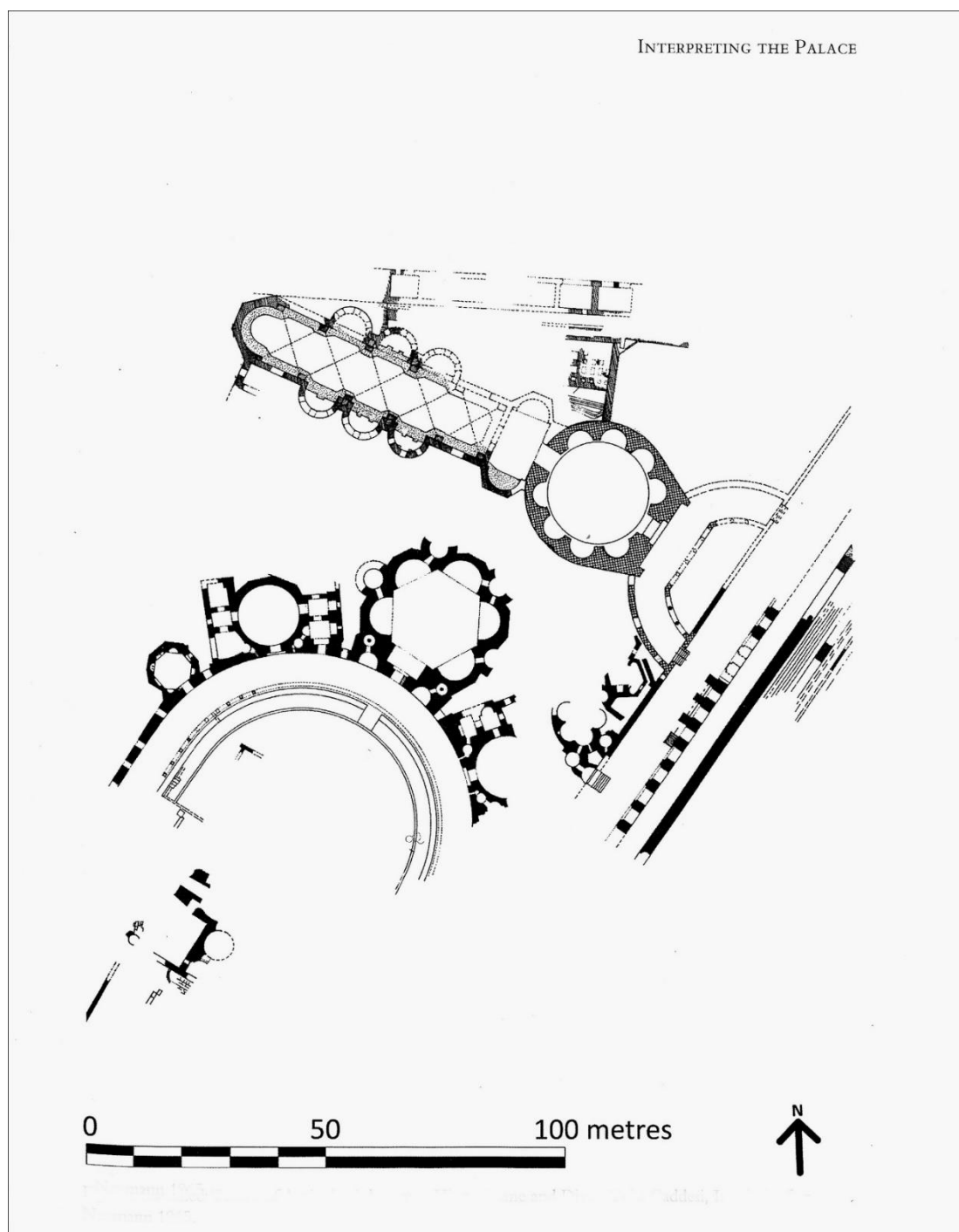
Fig. 192 : domus d'Antiochus : plan des fouilles, dans Westbrook, Architectural Interpretation , p. 77 (fig. 29)
