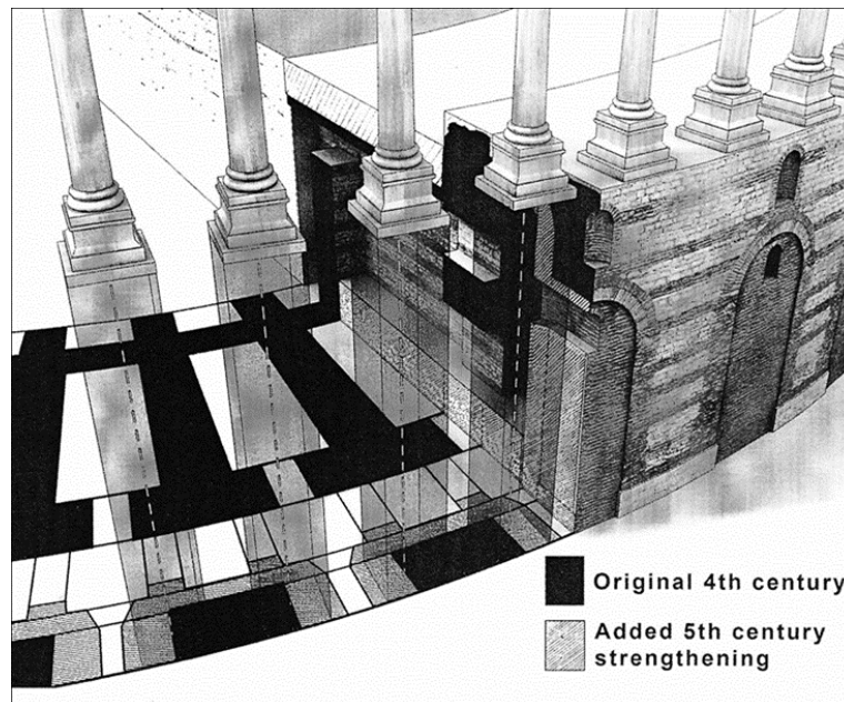
Fig. 144 : la sphendonè, dans Bardill, Hippodrome 1 , p. 133 (fig. 8.41) : en noir, la structure originelle ; en grisé les ajouts du V e siècle
