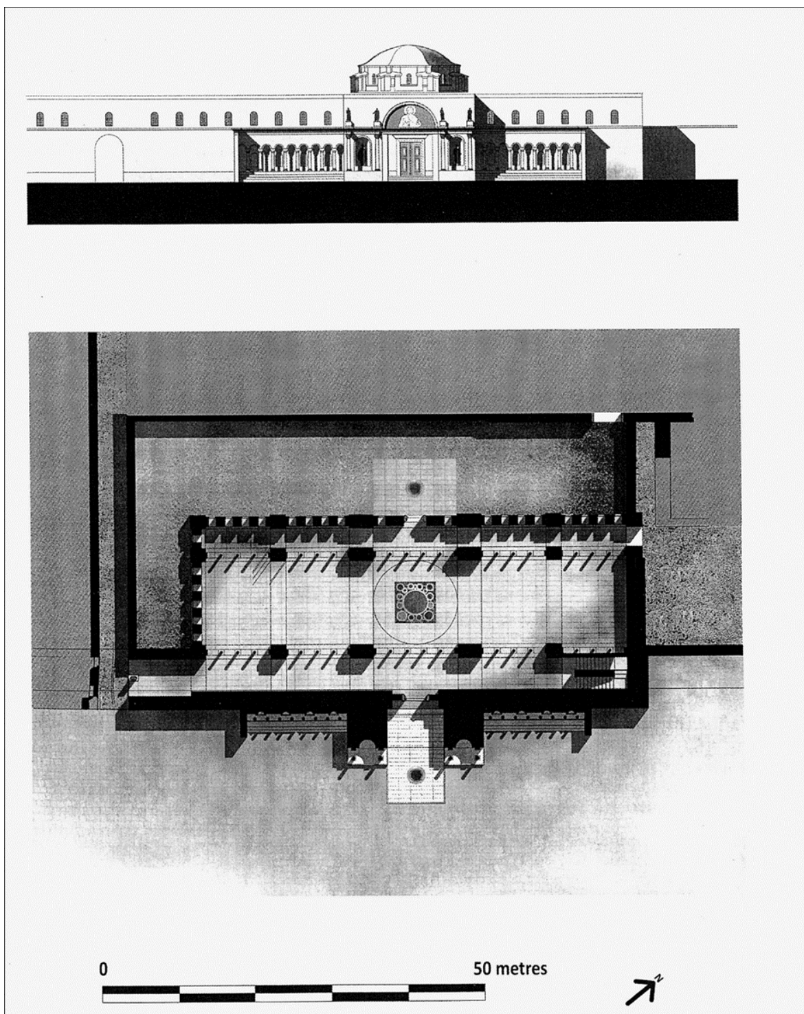
Fig. 43 : reconstitution hypothétique de la Chalkè, dans Westbrook, Architectural Interpretation , p. 189 (fig. 53-54)
