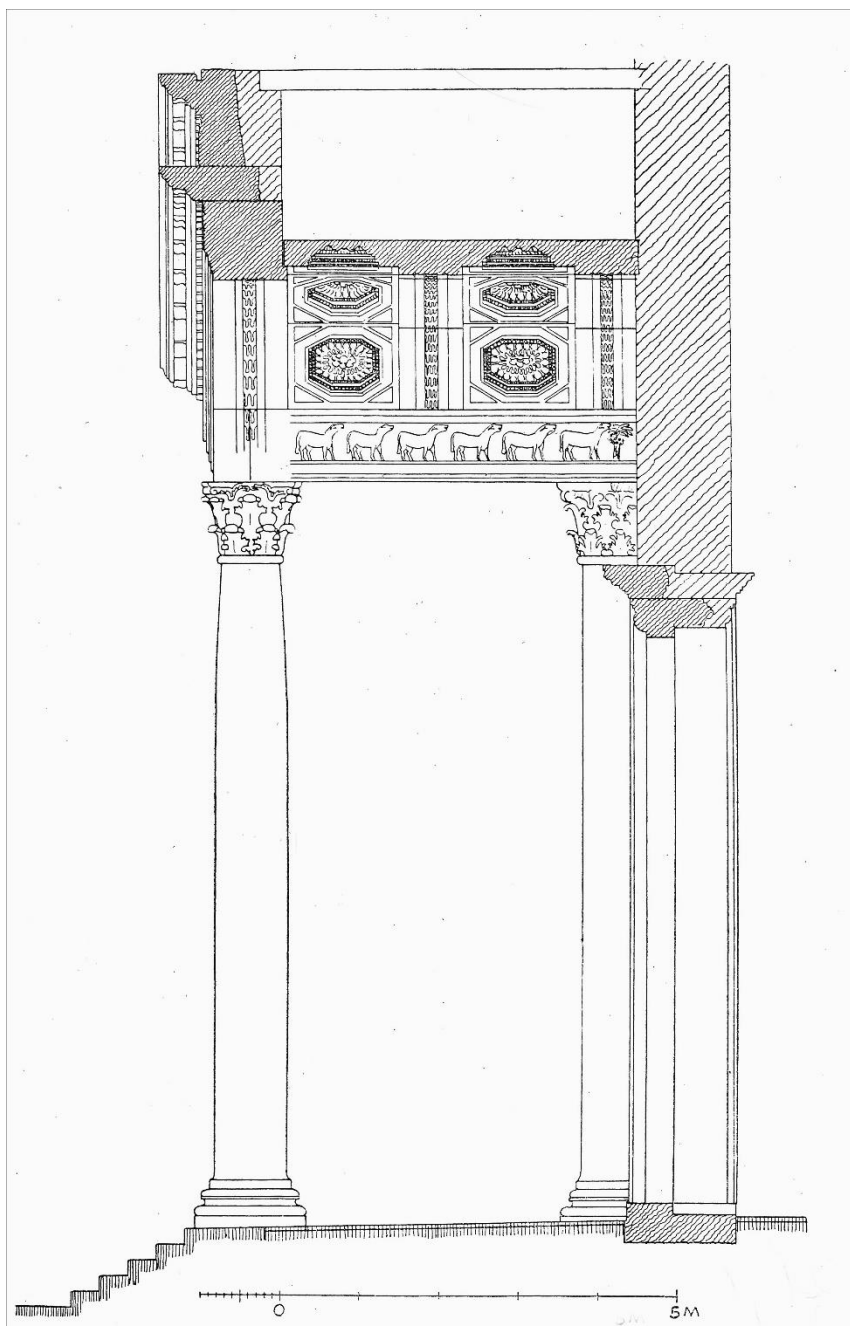
Fig. 53 : reconstitution du porche du portique de la Grande Église, dans Schneider, Grabung , tab. 4
