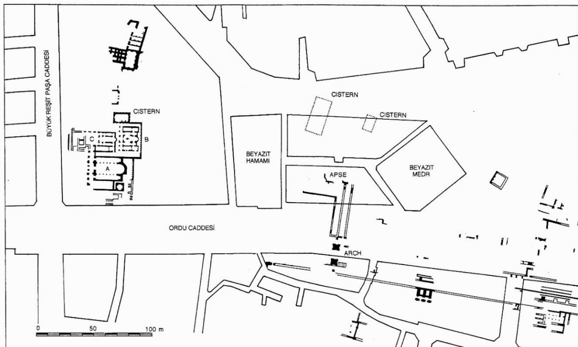
fig. 80 : plan montrant les vestiges du forum Theodosii , dans Bardill, Brickstamps , p. 131 (fig. 17)
