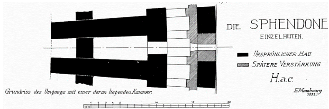
Fig. 140 : les substructures de la Sphendone, dans Mamboury-Wiegand, Kaiserpaläste , pl. CXI : en noir, la structure originelle ; en grisé, les structures de renforcement
