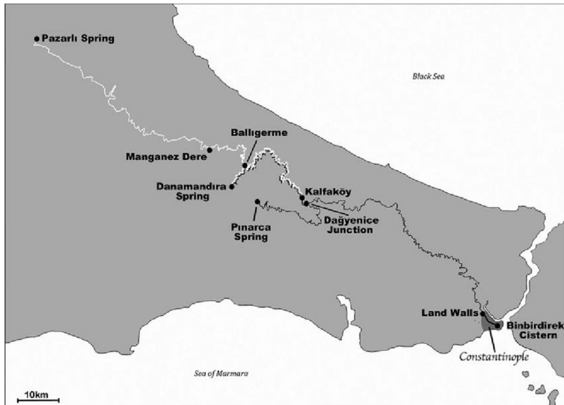
Fig. 158 : l'aqueduc de Thrace. En noir, la phase du IV e siècle. En blanc, la phase du V e siècle, dans Snyder, Landscape , p. 201 (fig. 2)
