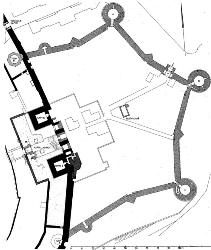
Fig. 136 : section entre la tour 8 et la Porte Dorée, dans Müller-Wiener, Bildlexicon , p. 292 (fig. 333)
