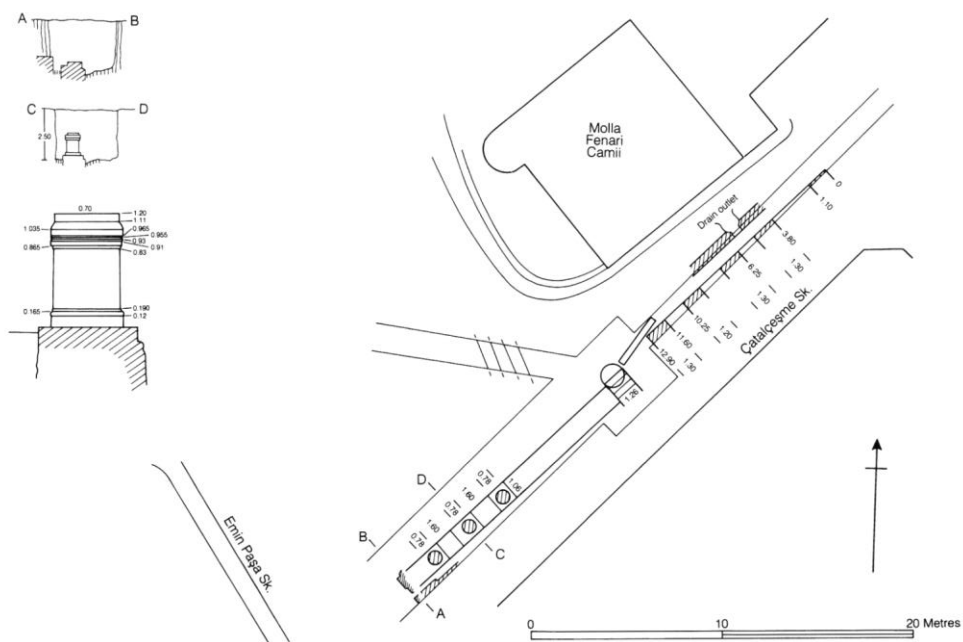
Fig. 15 : plan des découvertes dans Çatalçeşme Sokağı, dans Bardill, Lausus , p. 83 (fig. 9) (d'après E. Mamboury)
