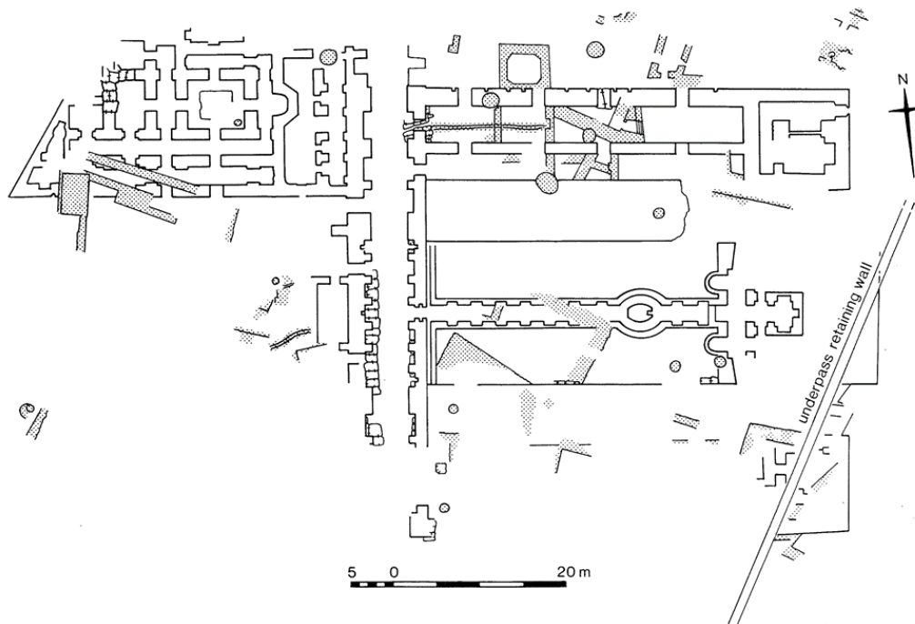
Fig. 216 : plan simplifié des fouilles de l'église Saint-Polyeucte, dans Harrison, Temple , p. 46 (fig. 39). Les structures du V e siècle sont en grisé
