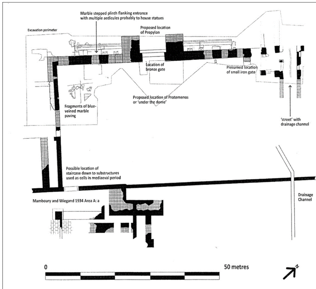
Fig. 35 : plan de la Chalkè d'après Girgin, Porte , fig. 19, repris dans Westbrook, Architectural Interpretation , p. 186 (fig. 52)
