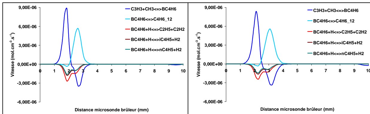
Figure 113 : Analyses des vitesses de formation et de consommation du but-1-yne ( \Phi = 2,16 à gauche; \Phi = 2,32 à droite).
