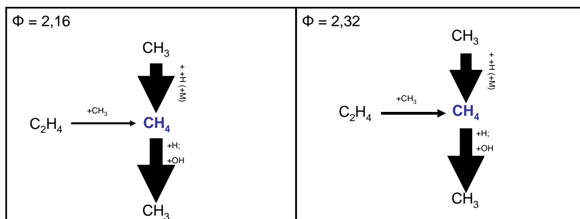
Figure 92 : Schéma cinétique de formation et de consommation du méthane dans les flammes n-butane/O 2 /N 2 ( \Phi = 2,16 et 2,32 à 1atm).
