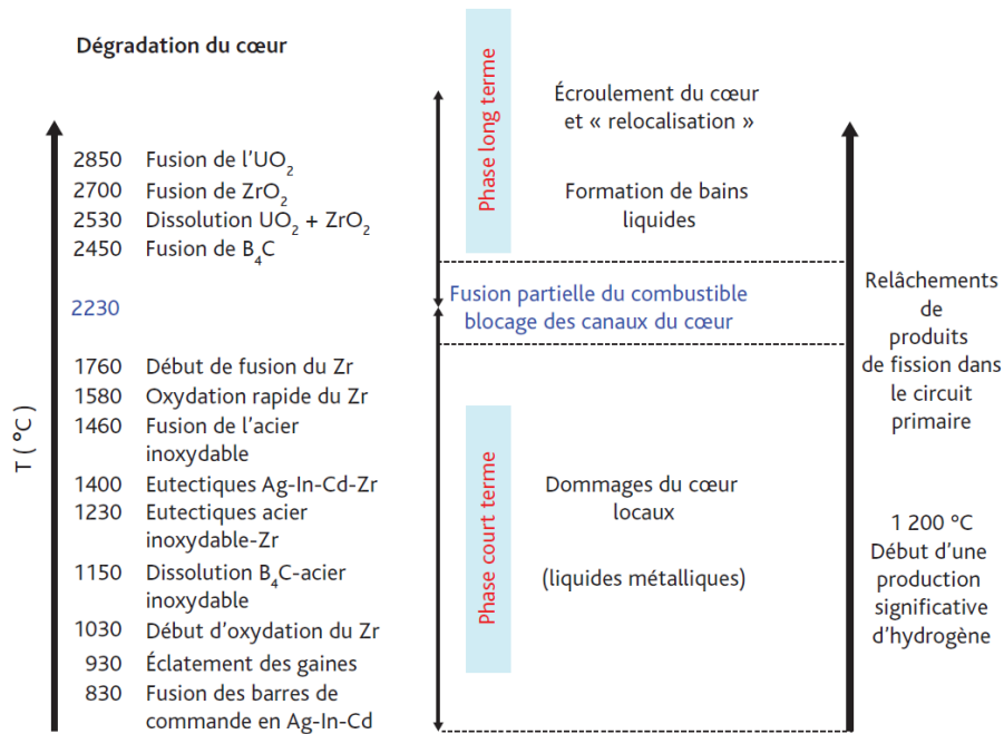
Figure 4. Principaux phénomènes intervenants au cours de la dégradation du cœur du réacteur ([5])
