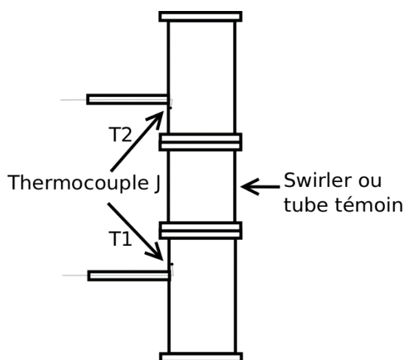
Figure 52. Dispositif de mesure de la température en paroi interne des tubes.
