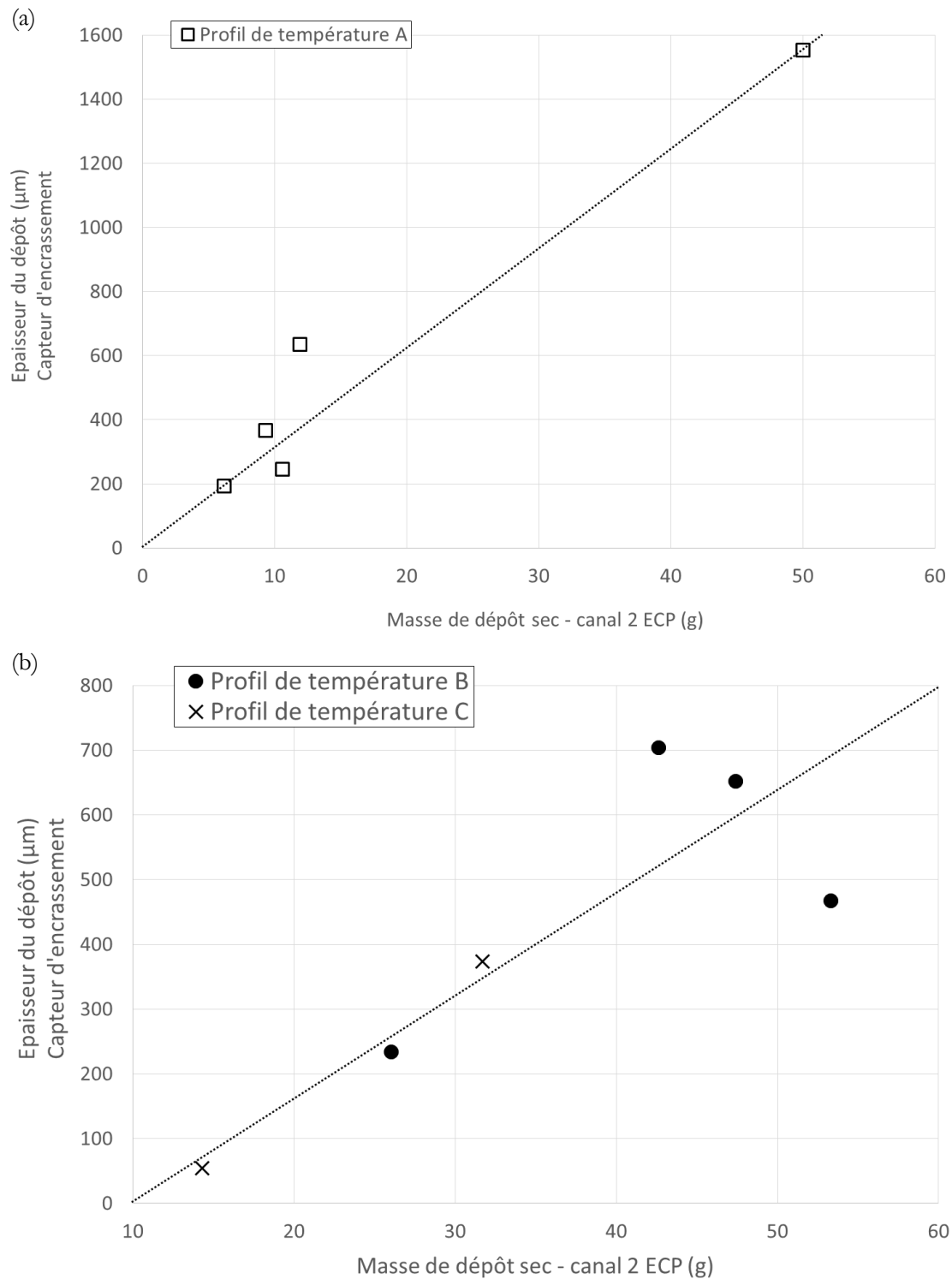
Figure 42. Épaisseur de dépôt mesurée par le capteur d'encrassement en fonction des masses de dépôt sec obtenues dans le canal 2 de l'échangeur pour les profils de température A, B et C.
