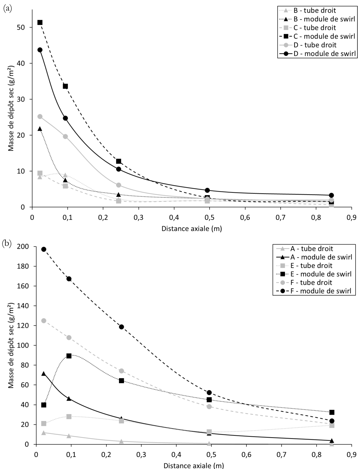
Figure 54. Évolution de la masse de dépôt sèche en aval du module de swirl ou d'un tube droit dans les conditions expérimentales A à F. L'erreur de mesure est inférieure à 1 \text{ g}/\text{m}^2 .
