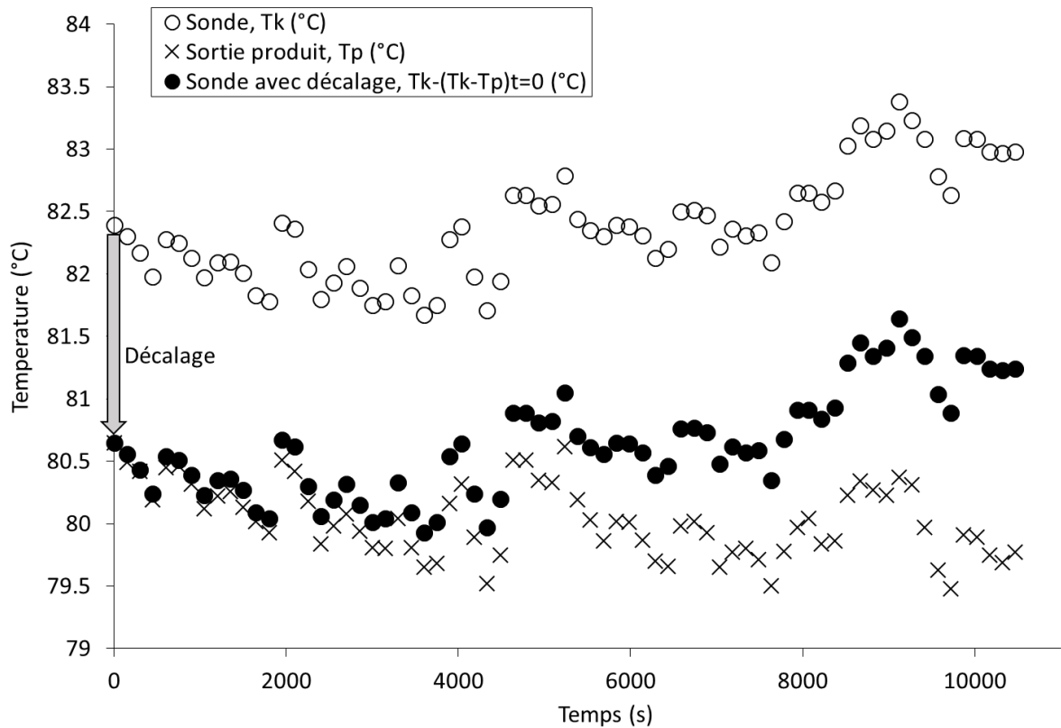
Figure 40. Températures enregistrées lors de l'encrassement avec le profil C.
