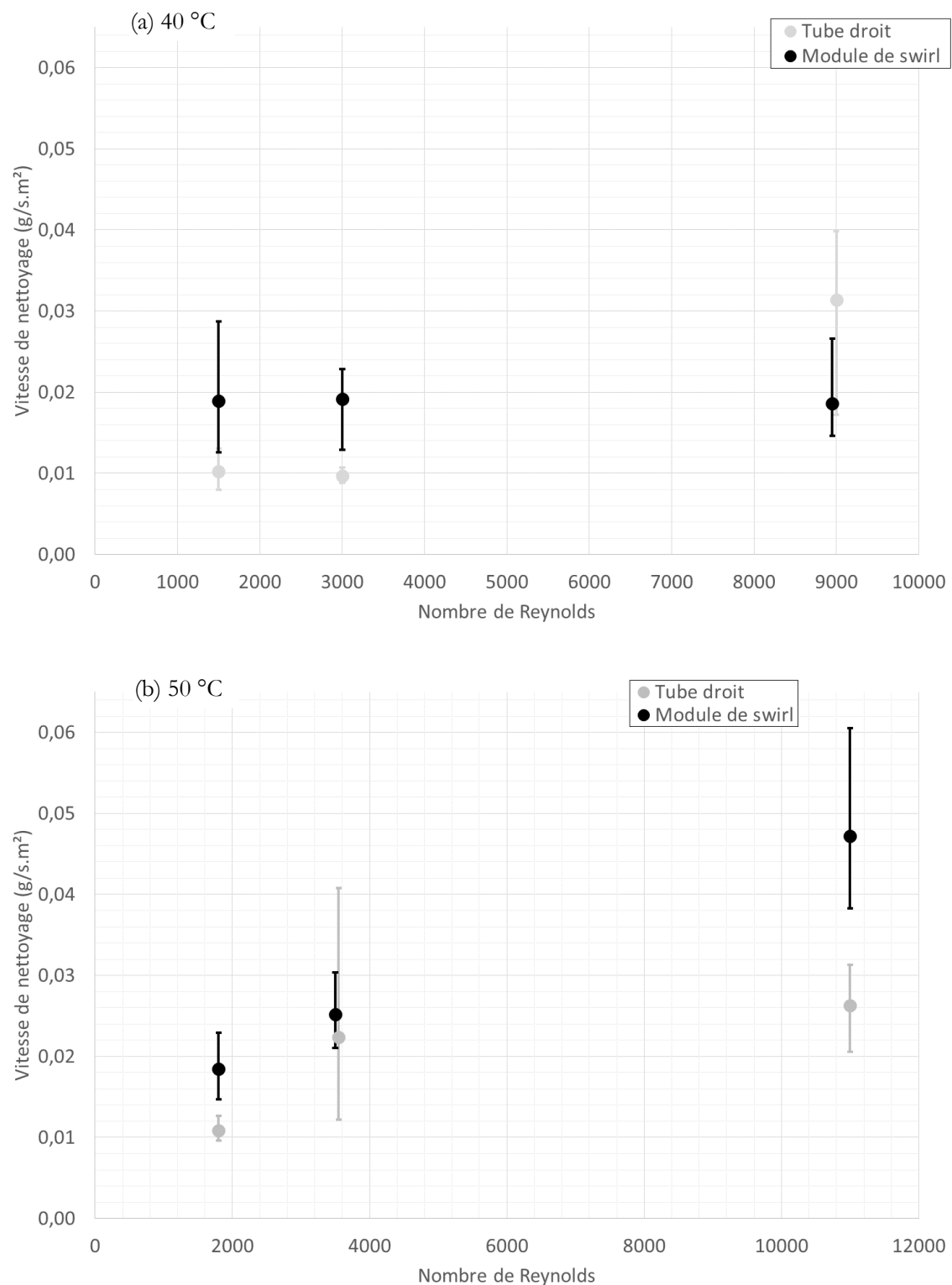
Figure 61. Comparaison des vitesses de nettoyage par une solution d'hydroxyde de sodium à 0,5 % (p/p) à une température de 40 °C (a) et 50 °C (b) après un tube droit ou un module de swirl. Les valeurs minimales, moyennes et maximales sont représentées.
