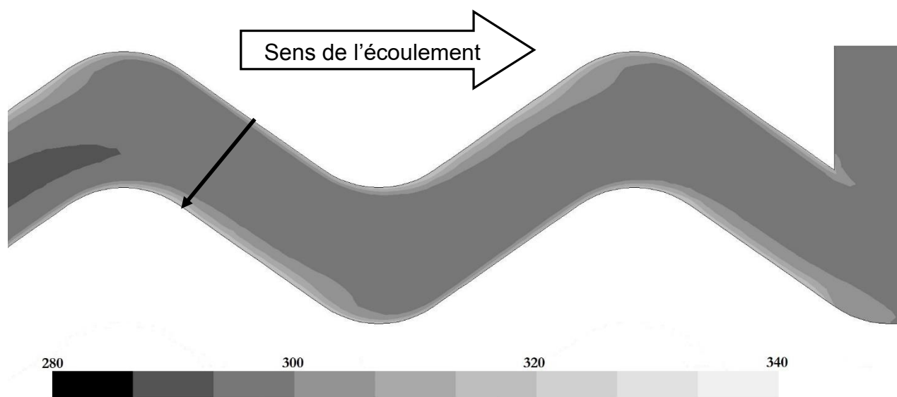
Figure 20. Champ de température (Kelvin) avant la sortie du 4 ème canal.
