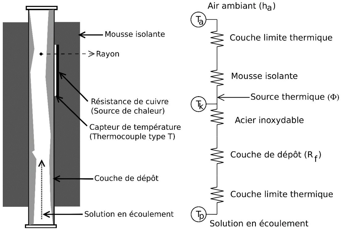
Figure 35. (a) Vue en coupe du capteur d'encrassement. (b) Schéma thermique équivalent sur un rayon. T_p , T_k et T_p symbolisent respectivement la température du fluide en circulation, du capteur et de l'air ambiant. h_a , \Phi et R_f représentent respectivement le coefficient de transfert thermique vers l'air ambiant, le flux de chaleur surfacique et la résistance thermique d'encrassement.
