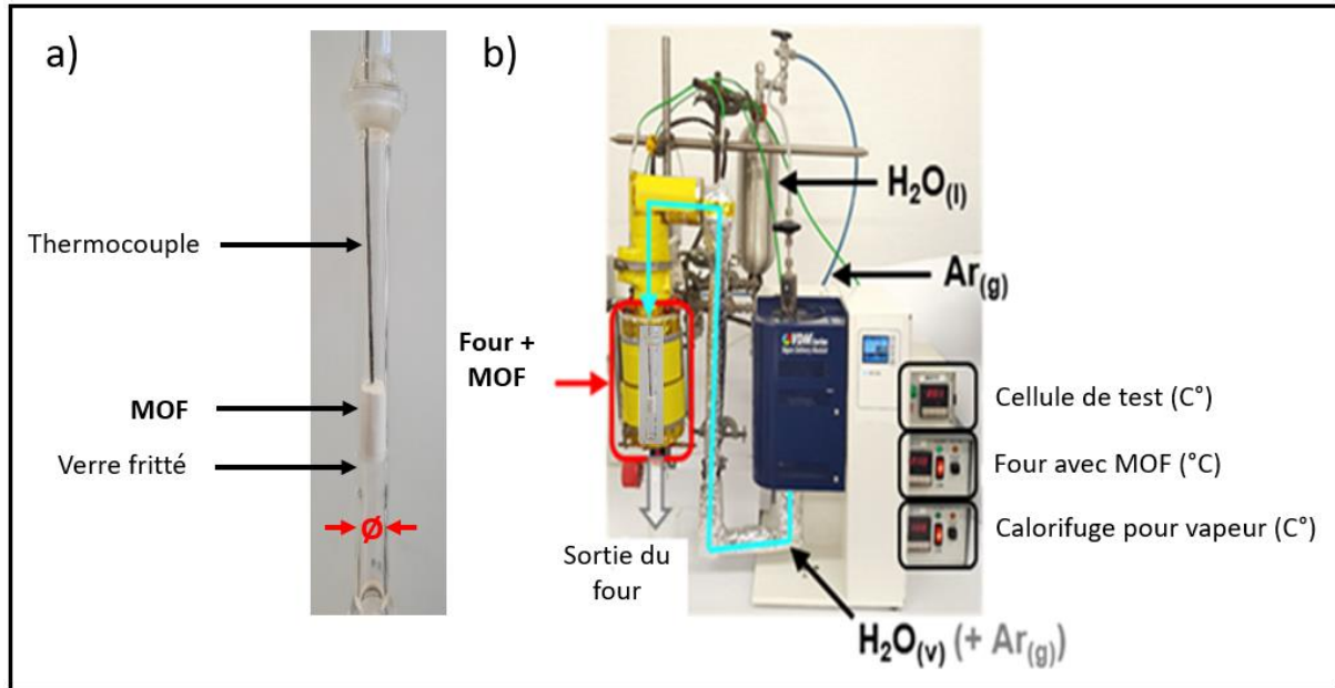
Figure 20 : a) Photo de la cellule d'échantillonnage avec un diamètre interne Ø de 10 mm ; b) Photo du montage expérimental, la ligne d'approvisionnement en vapeur est mise en évidence par un tracé bleu turquoise.
