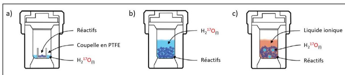
Figure 39 : Représentation de différents modes d'enrichissement ^{17}\text{O} pendant la synthèse du MOF : a) Approche DGC ; b) synthèse hydrothermale et c) synthèse ionothermale. Schémas issus des travaux d'Ashbrook et al. 7 .
