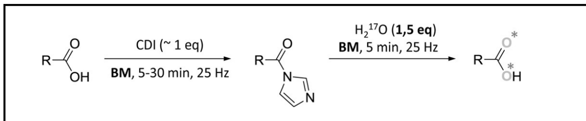
Figure 41 : Schéma de l'élaboration de composés enrichis en oxygène-17 par mécanosynthèse tiré des travaux de Métro et al. 19 . Au cours de cette thèse, cette méthode a été utilisée pour l'enrichissement des groupements carboxyliques de l'acide téréphthalique.
