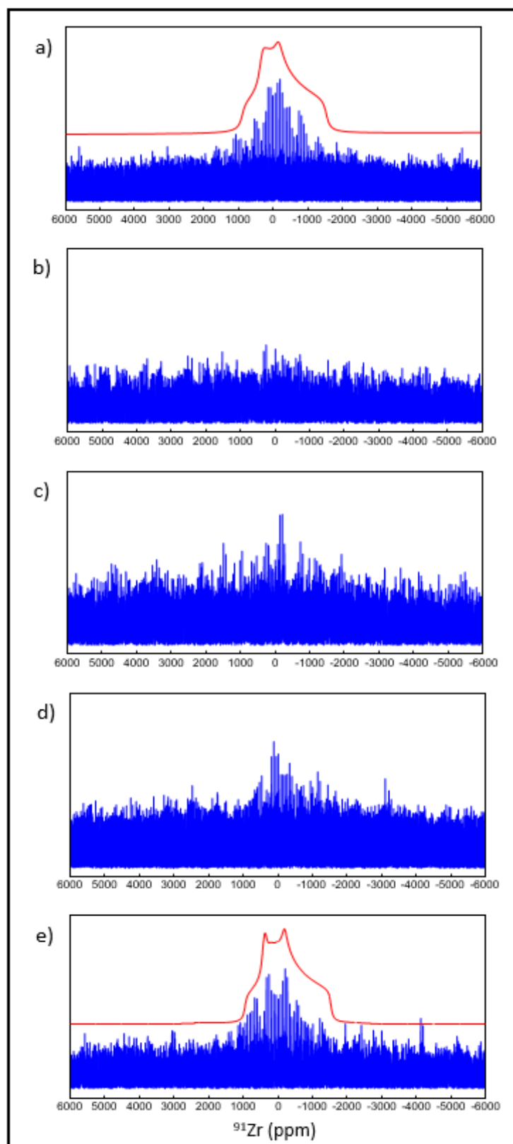
Figure 67 : Spectres RMN 1D ^{91}\text{Zr} WURST-QCPMG de l'UiO-67- \text{NH}_2(\text{Zr}) enregistrés à 120 K (a) avant et (b) après traitement à la vapeur d'eau à différentes températures (b) 80 °C (c) 100 °C, (d) 150 °C, et (e) 200 °C. Les spectres expérimentaux sont en bleu et l'enveloppe des spectres simulés avec le logiciel DMFIT sont en rouges. Les spectres sont accumulés pendant 20 heures ( NS = 70\,000 , RD = 1s ).
