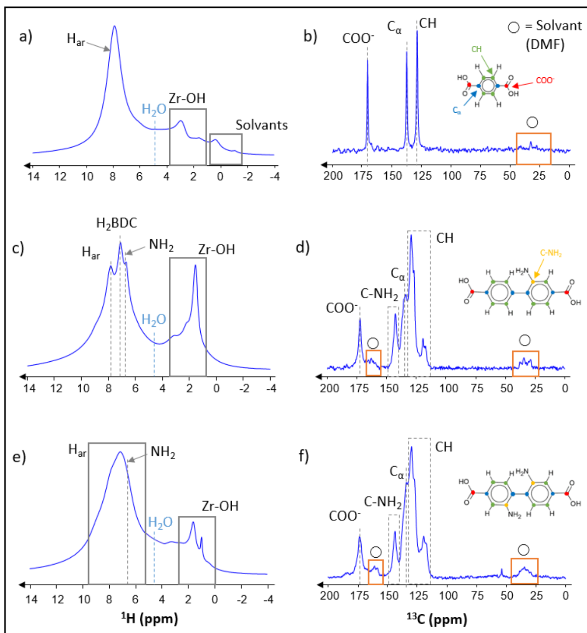
Figure 24 : Spectres RMN a – c – e) ^1\text{H} MAS et b – d – f) ^{13}\text{C} MAS des différents composés UiO-66(Zr) de référence (spectres a et b), UiO-67- \text{NH}_2 (Zr) de référence (spectres c et d) et UiO-67- (\text{NH}_2)_2 (Zr) de référence (spectres e et f) obtenus après synthèse. Les spectres sont enregistrés à B_0 = 9,4 \text{ T} et \nu_R = 20 \text{ kHz} . a – c – e) ^1\text{H} DEPTH NS = 16, \tau_{RD} = 5 \text{ s} et b – d – f) ^1\text{H} \rightarrow ^{13}\text{C} CPMAS NS = 1024, \tau_{RD} = 2 \text{ s} , \tau_{CP} = 2 \text{ ms} et un découplage ^1\text{H} SPINAL-64 a été employé pendant l'acquisition. L'attribution des spectres est indiquée sur la figure.
