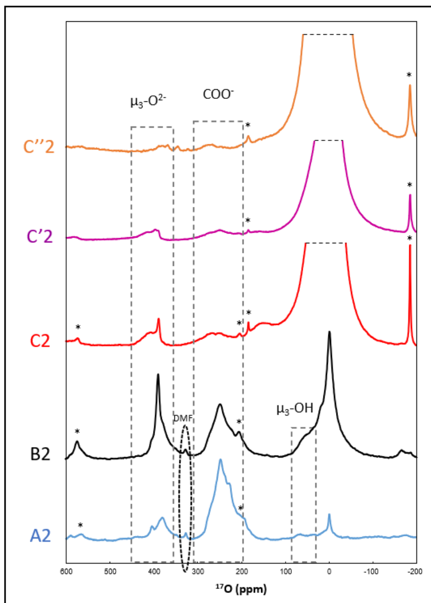
Figure 48 : Comparaison des spectres RMN ^{17}\text{O} 1D après diffusion d'eau (étape 2) pour les 5 échantillons. Les spectres sont enregistrés à B_0 = 18,8 \text{ T} et \nu_R = 20 \text{ kHz} , NS = 7500 et \tau_{RD} = 1 \text{ s} . * correspond aux bandes de rotation.
