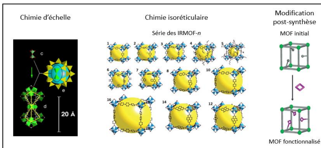
Figure 5 : Illustration des concepts de chimie d'échelle 24 et de chimie isoréticulaire 25 pour la série des IRMOF-n et des modifications post-synthèse 26 .
