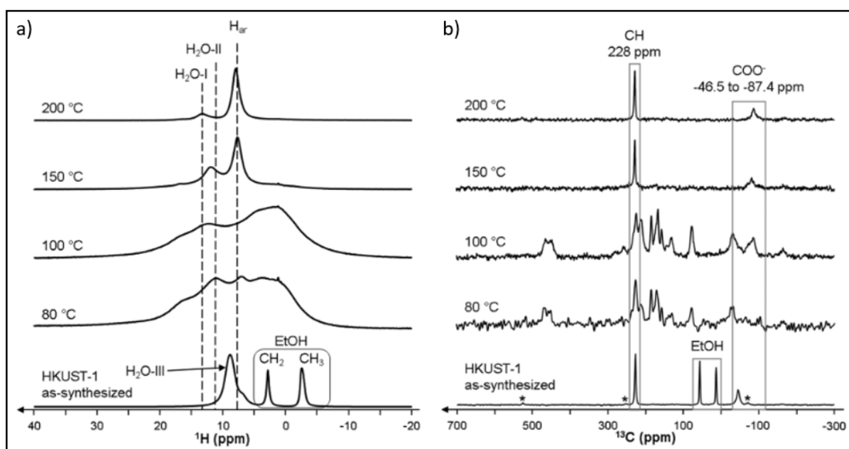
Figure 18 : Spectres RMN 1D a) ^1\text{H} et b) ^{13}\text{C} du composé HKUST-1 en fonction de son exposition à la vapeur d'eau à différentes températures extraites de la publication de Giovine et al. 1 .
