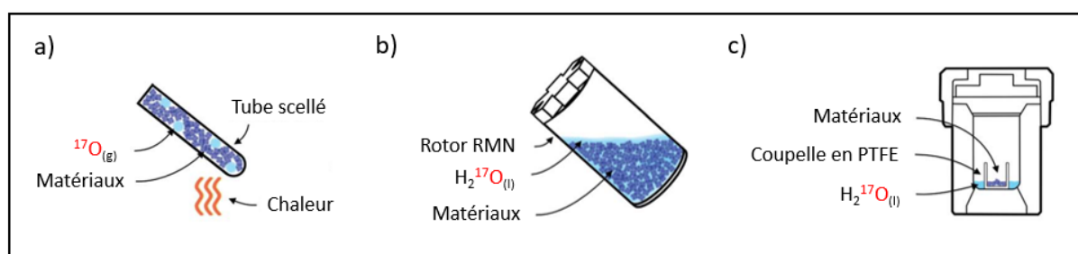
Figure 40 : Représentation de différents modes d'enrichissement ^{17}\text{O} après la synthèse du MOF : a) Enrichissement par gaz enrichi ^{17}\text{O}_{2(\text{g})} ; b) imprégnation dans le rotor RMN et c) échange hydrothermale avec \text{H}_2^{17}\text{O} . Schémas issus des travaux d'Ashbrook et al. 7 .
