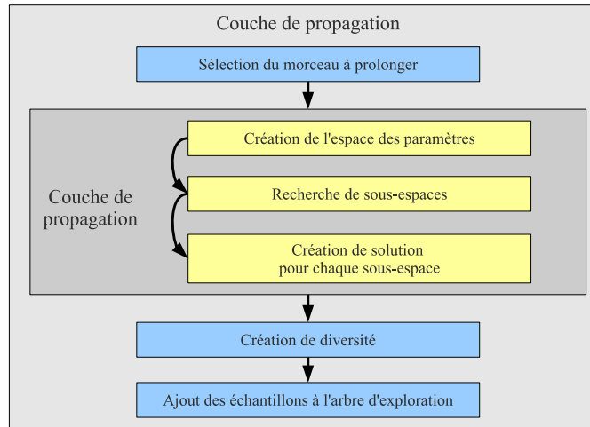
FIGURE 4.1 – Architecture de DKP, planificateur de trajectoires pour robots à deux roues indépendantes, basé sur une approche de planification de trajectoire par échantillon. Ce type d'architecture repose sur l'interaction d'une couche de propagation, qui génère des nouveaux échantillons, avec une couche de sélection, qui détermine les morceaux à prolonger placés dans un arbre d'exploration. L'originalité repose sur une nouvelle couche de propagation qui détermine un espace des paramètres représentant l'ensemble des solutions localement réalisables, avec le respect des contraintes posées sur le modèle du robot. Cette couche permet de plus de ne sélectionner que les parties de l'arbre réellement prolongeables
