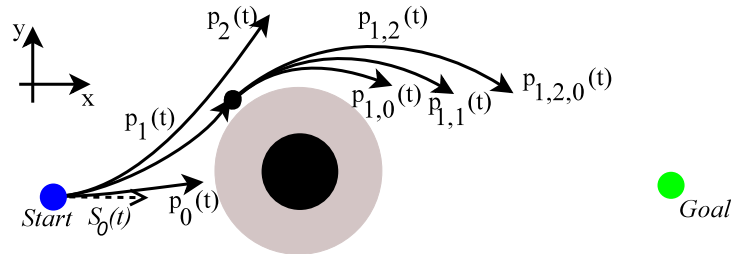
FIGURE 4.7 – La diversité de la durée des échantillons permet à l’arbre d’exploration de ne pas rester coincé dans les minima locaux. Les morceaux courts permettent d’avoir de la manœuvrabilité autour des obstacles alors que les morceaux longs permettent de franchir rapidement des zones larges sans obstacles.
