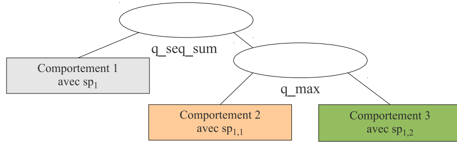
FIGURE 5.8 – Croissance d’une alternative dans l’arbre de pilotage lorsque plusieurs paramètres de pilotage sont associés à une même surface de déclenchement.
