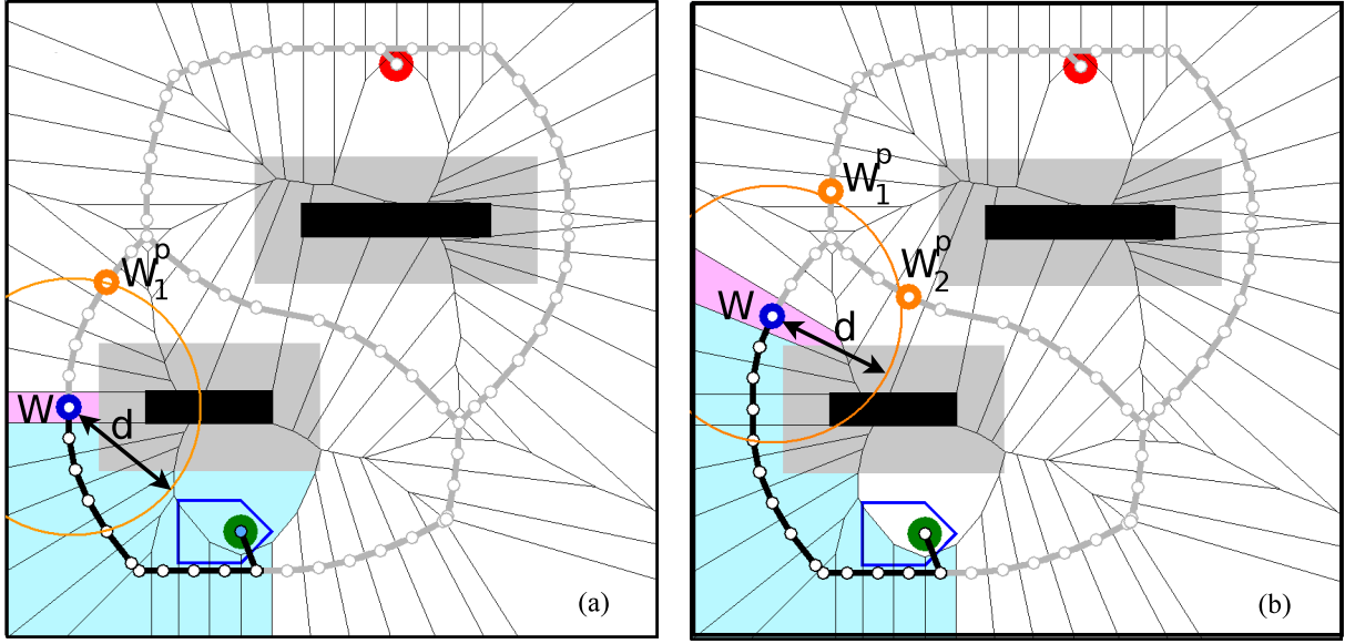
FIGURE 5.13 – Point de passage W de la roadmap choisi en fonction de la position du robot M et les points de passage projetés W_i^p à une distance d . (a) un point de passage projeté, sur une branche, avant un embranchement, (b) deux points de passage projetés, sur deux branches, après un embranchement.
