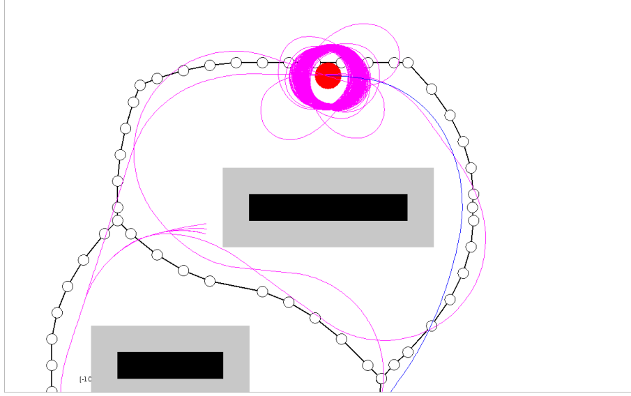
FIGURE 5.19 – Problèmes de convergence liés au surguidage du mode backtrack lors de l'atteinte d'un objectif, ici un disque de rayon 0.01m centré sur l'objectif.
