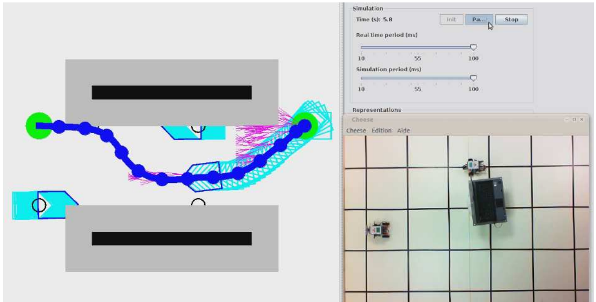
FIGURE 6.1 – Dépassement simulé par DKP puis appliqué à nos robots grâce à APM(Robot).
