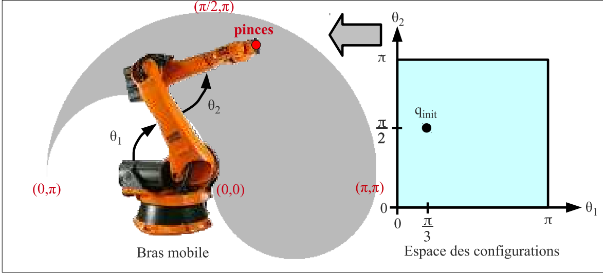
FIGURE 1.6 – Espace de travail dans un exemple continu : c'est la localisation possible du point de référence (ici, le centre des pinces) pour toutes les configurations (\theta_1, \theta_2) .
