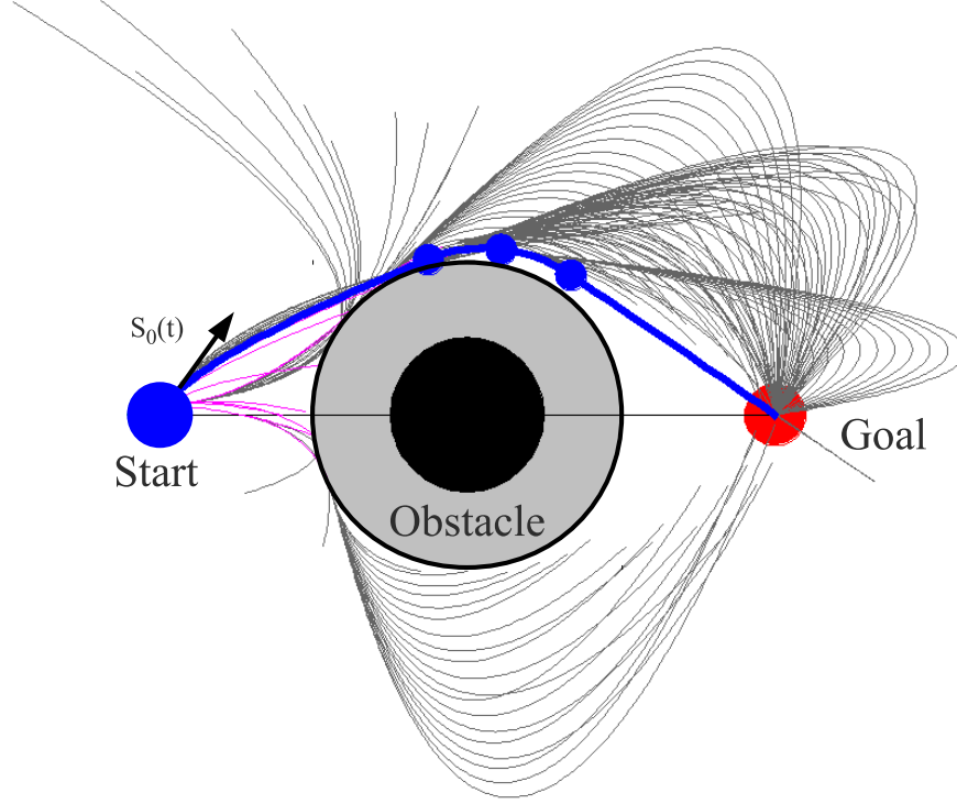
FIGURE 4.8 – Représentation de l'arbre d'exploration construit par DKP. Les échantillons de trajectoires apparaissent en gris foncé. Les échantillons sélectionnés par DKP pour être prolongés sont dessinés en magenta. En gras est tracée la première trajectoire qui satisfait le critère d'arrêt de la recherche de solution, c'est-à-dire rejoindre la région de l'environnement autour de Goal .
