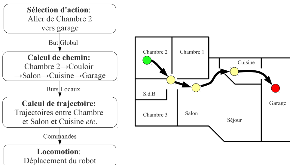
FIGURE 2.6 – Étapes de raisonnement à effectuer pour réaliser un déplacement selon le modèle Top Down de Craig Reynolds. Un robot est situé dans la chambre 2 ; le planificateur décide de l'objectif : aller au garage. Le niveau de planification discrète décide du chemin : passer par le couloir puis le salon, la cuisine et enfin le garage. Ensuite, la couche de planification continue établit les trajectoires entre ces points de passage : trajectoire entre la chambre 2/couloir, couloir/salon, salon/cuisine et cuisine/garage. Enfin, le niveau de locomotion effectue le déplacement effectif du robot depuis la chambre 2 jusqu'au garage en suivant les trajectoires déterminées par le niveau précédent.
