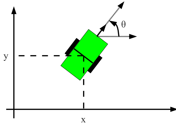
FIGURE 1.1 – Pour un robot à deux roues indépendantes, les variables permettant de décrire le robot dans un environnement ne sont que la position et l'angle du robot dans l'environnement. Le robot ne porte pas d'articulation : il ne possède donc pas de degré de liberté supplémentaire.
