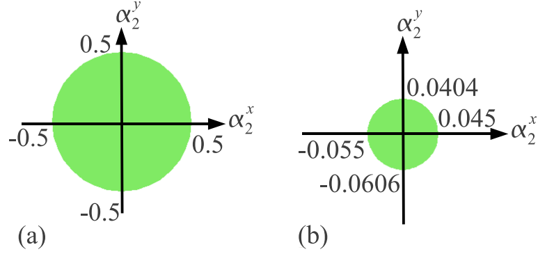
FIGURE 3.16 – Les contraintes (a) d'accélération linéaire et (b) de vitesse linéaire, projetées dans l'espace des paramètres après évaluation sur tous les pas de temps de la planification.
