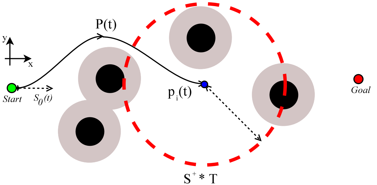
FIGURE 3.10 – La surface entourée par les tirets rouges délimite les points atteignables à partir de la borne maximale de la contrainte de vitesse S^+ pour le problème de planification local partant du point en bleu et sur un horizon de planification T .
