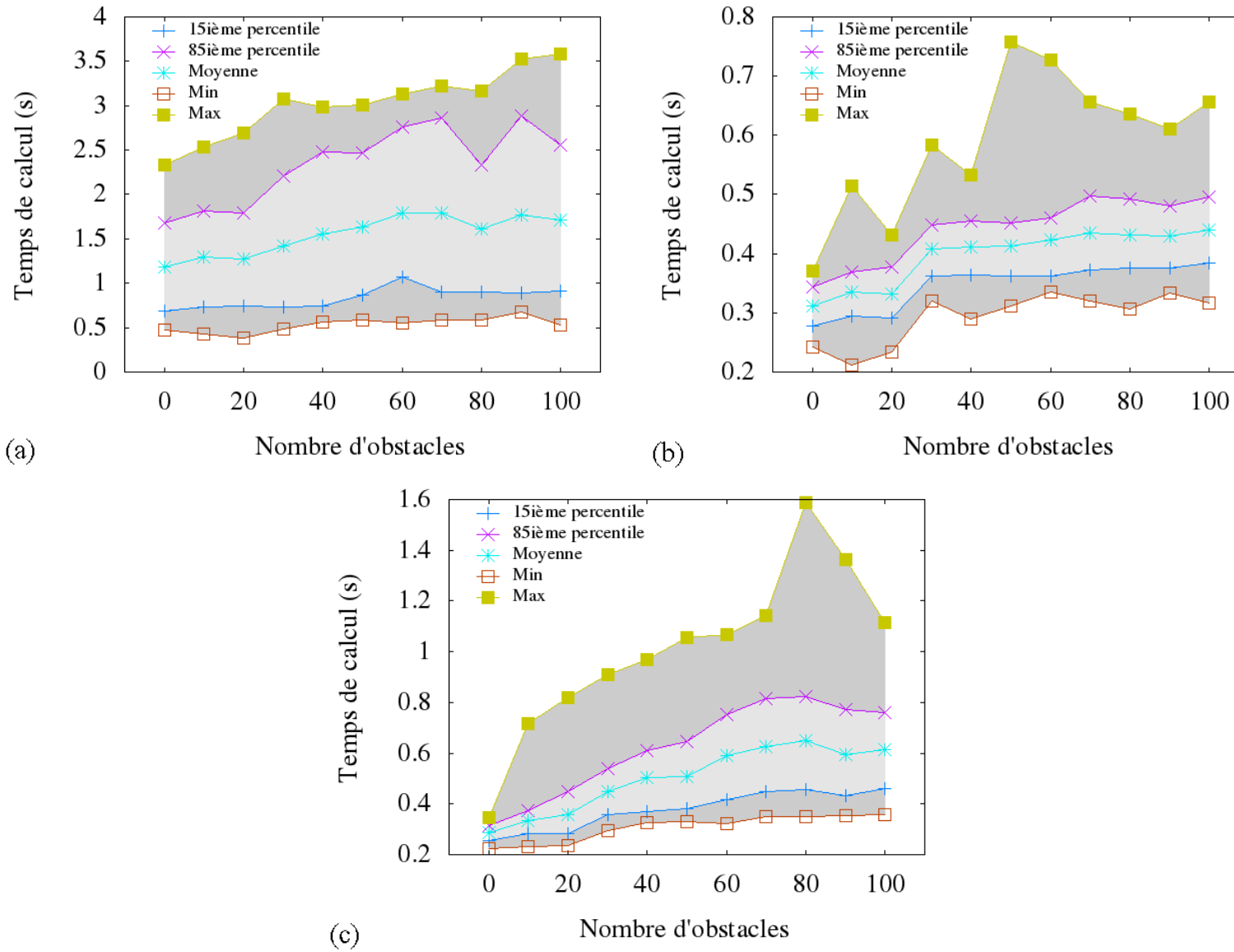
FIGURE 4.15 – Moyennes, minima, maxima, 15 ième et 85 ième percentiles des temps de calcul pour 1100 simulations de DKP dans le mode (a) optimal (avec les paramètres de la Table 4.1 ligne 2), (b) glouton (avec les paramètres de la Table 4.1 ligne 4) et (c) backtrack (avec les paramètres de la Table 4.1 ligne 5). Ces résultats sont donnés pour des environnements contenant [0, 10, \dots, 100] obstacles.
