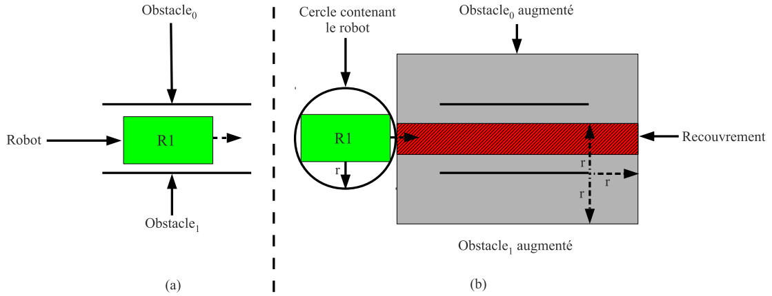
FIGURE 1.9 – Défaut dans l'approximation de la taille d'un robot dans le cas d'un passage exigü : (a) si sa forme exacte est prise en compte, le robot peut passer dans le couloir et (b) si le robot est ramené à un point, soit r le rayon du disque recouvrant complètement sa surface, si la taille des obstacles est augmentée de ce rayon, alors le passage n'apparaît plus franchissable car les obstacles se recouvrent dans la surface hachurée en rouge.
