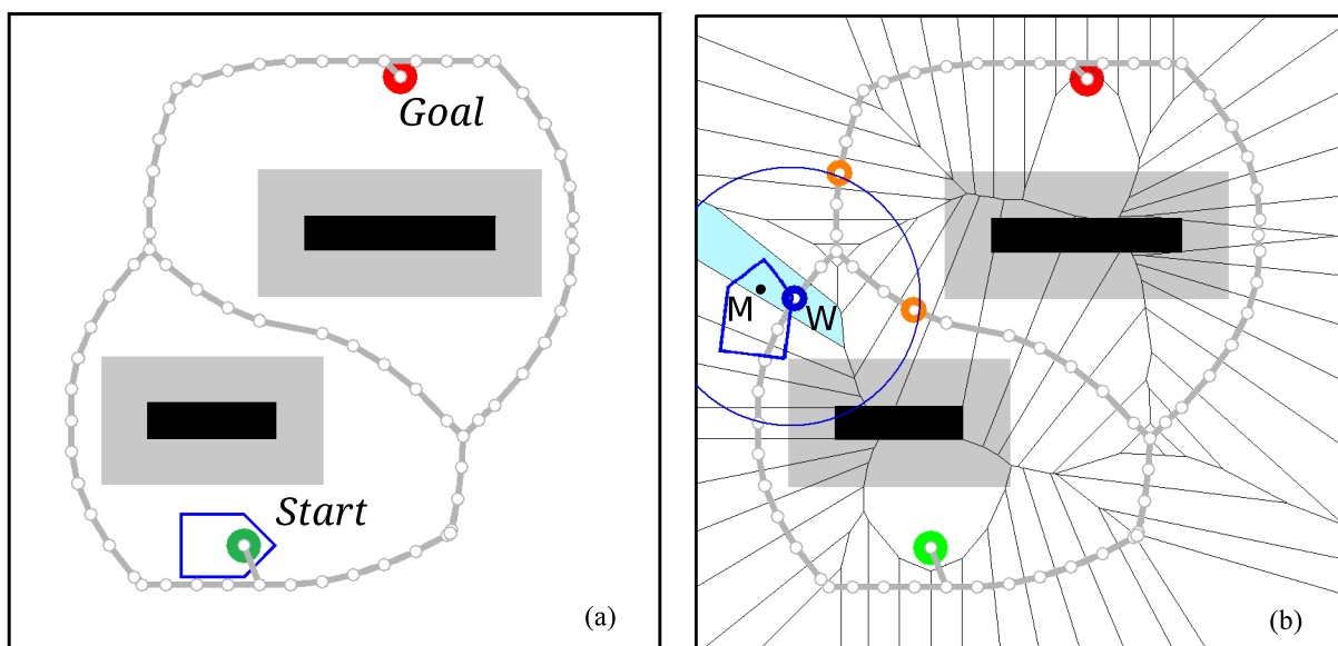
FIGURE 5.11 – (a) Une roadmap issue de la simplification du diagramme de Voronoï (les lignes grises épaisses). (b) Méta-diagramme de Voronoï (les lignes noires épaisses) associant une unique surface à chaque point de passage de la roadmap.
