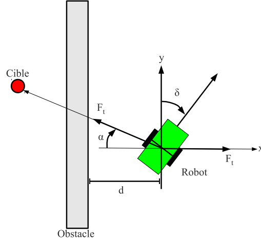
FIGURE 2.3 – Une situation généralisée de l'application des champs de potentiel.
