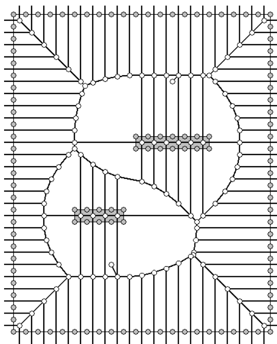
FIGURE 2.11 – Construction du diagramme de Voronoï à partir de la discrétisation du bord de l'environnement et des obstacles, obtenu à partir d'une triangulation de Delaunay.
