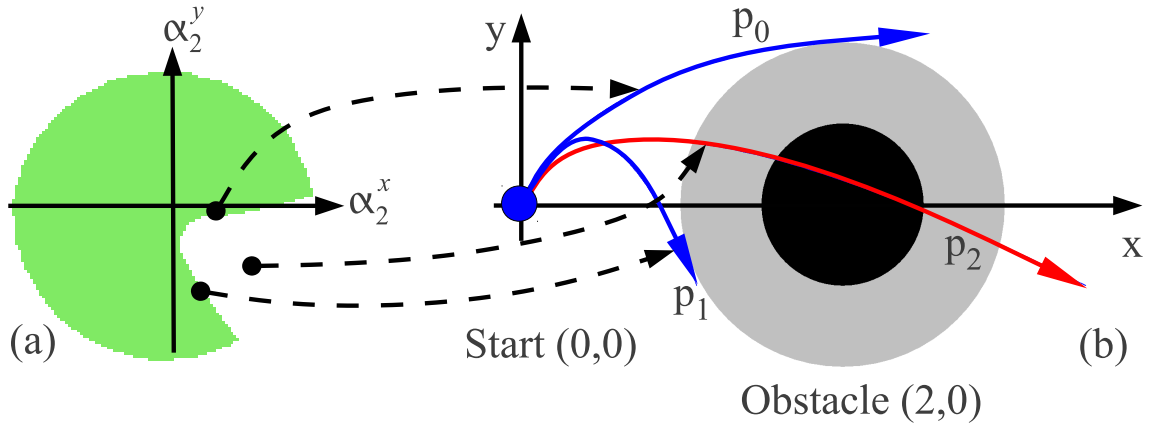
FIGURE 3.18 – La surface en vert (a) contient l'ensemble des paramètres (\alpha_2^x, \alpha_2^y) valides qui sont éligibles comme solutions, car ils respectent toutes les contraintes du problème. (b) montre l'impact du choix d'un point (\alpha_2^x, \alpha_2^y) sur la forme d'un échantillon. Le choix des paramètres (\alpha_2^x, \alpha_2^y) en dehors de l'espace des paramètres conduit à la violation d'une ou plusieurs contraintes, ici la contrainte d'évitement d'obstacle.
