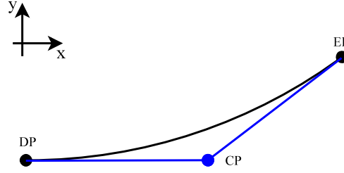
FIGURE 7.2 – Une quadratique et son polygone de contrôle.
