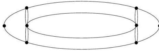
FIGURE 2.12 – Points critiques obtenus dans un tore par la méthode silhouette, image tirée de [LaValle, 2006].
