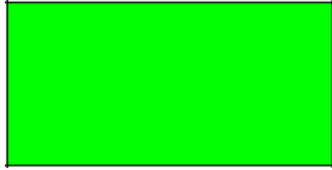
FIGURE 7.5 – Un rectangle et ses sommets.
