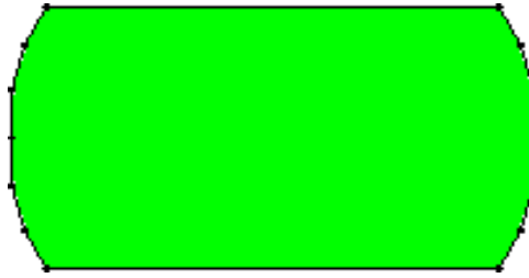
FIGURE 7.8 – L'intersection d'un disque par un rectangle.
