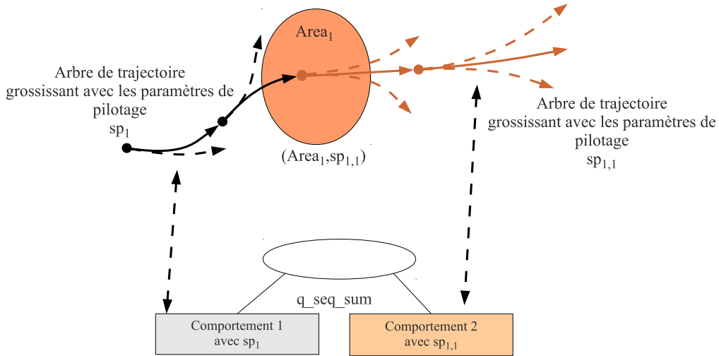
FIGURE 5.6 – Croissance d'une séquence dans l'arbre de pilotage lorsqu'un paramètre de pilotage est le seul successeur d'un paramètre de pilotage précédent.
