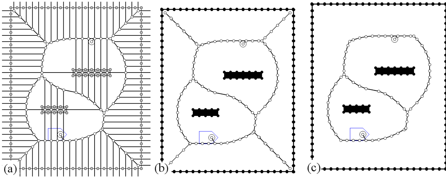
FIGURE 5.10 – Étapes de construction du diagramme de Voronoï sur l'environnement proposé dans cet exemple : (a) un diagramme de Voronoï est construit autour de la discrétisation des obstacles et des bords ; (b) les segments coupant un obstacle ou le bord sont retirés ; (c) les segments menant à une impasse sont retirés
