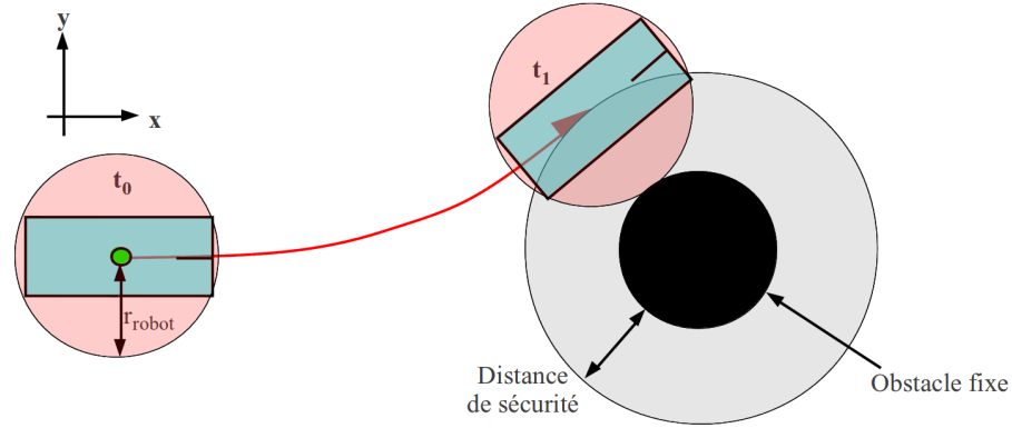
FIGURE 3.7 – Contrainte sur un obstacle fixe, avec grossissement de l’obstacle en fonction d’un écartement prenant en compte à minima l’empatement du robot.
