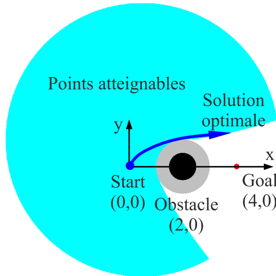
FIGURE 3.19 – La surface en cyan est construite à partir de tous les points finaux des trajectoires valides construites à partir de points de l'espace des paramètres. Cette figure est simplement obtenue en projetant l'espace des paramètres dans l'espace des positions pour t = T . Sur cette surface, il suffit de rechercher le point minimisant la distance à Goal pour obtenir la trajectoire localement optimale.
