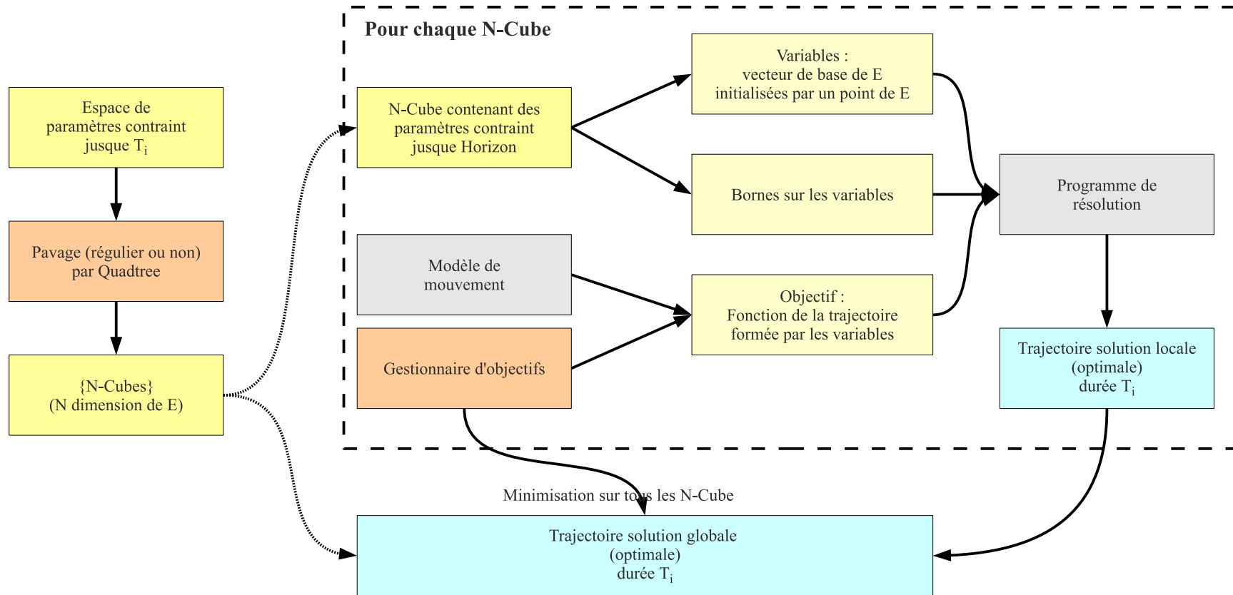
FIGURE 3.12 – Dans cette approche, l'espace des paramètres est d'abord pavé par un Quadtree. L'avantage de cette approche est que l'on peut utiliser un programme de résolution de problèmes d'optimisation non-linéaires à variable continues bornées. Les variables sont les paramètres laissés libres de la solution. Ces variables sont bornées par les n-cubes. De tels programme de résolution comme BLMVM peuvent fournir la solution optimale sur le pavé considéré. La contrainte est qu'il faut itérer cette méthode sur tous les pavés
