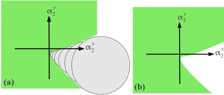
FIGURE 3.17 – La contrainte d'évitement d'obstacle projetée dans l'espace des paramètres. La figure (a) montre l'empreinte de l'obstacle qui extrude sur la figure (b) l'espace des paramètres pour chaque pas step jusqu'à l'horizon de planification T .
