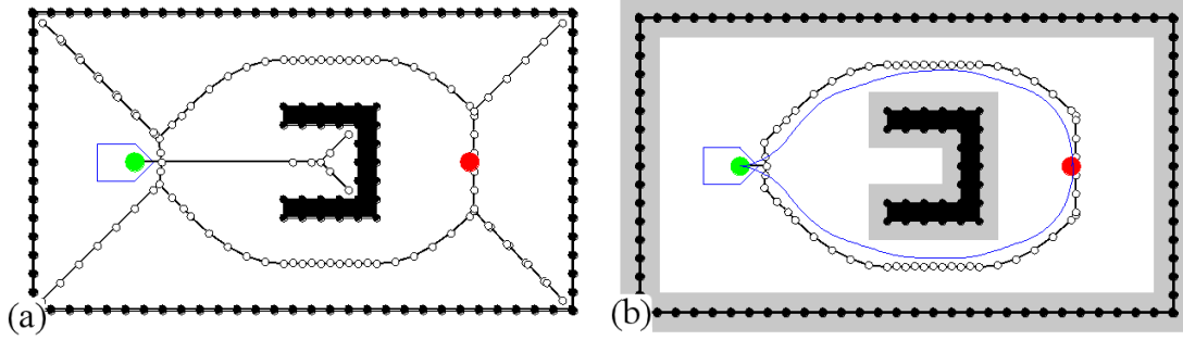
FIGURE 5.18 – Solutions obtenues en utilisant le mode backtrack de DKP et avec guidage sur un obstacle U. La roadmap est initialement constituée de trois parties : la première branche va vers le fond du U, les deux autres contournent l’obstacle. Toutefois, seules ces deux dernières servent au guidage et permettent le développement de deux solutions symétriques.
