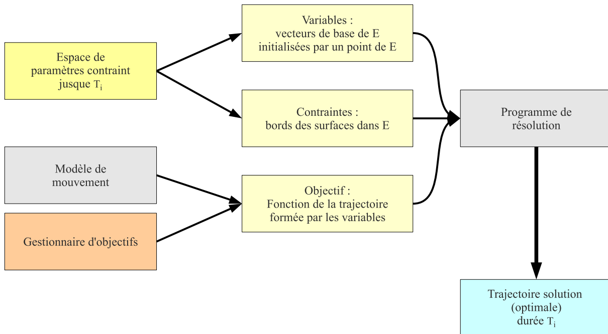
FIGURE 3.11 – Le problème de planification de trajectoire est fourni à un programme de résolution de problèmes d'optimisation non-linéaires à variables continues sous contraintes non-linéaires. Les variables sont les paramètres laissés libre de la solution. L'espace des paramètres est transformé en un jeu de contraintes permettant de borner les valeurs des variables dans cet espace. Le problème est initialisé avec un point appartenant à l'espace des paramètres. Enfin, la recherche est effectuée selon un critère d'optimisation appliqué aux variables.
