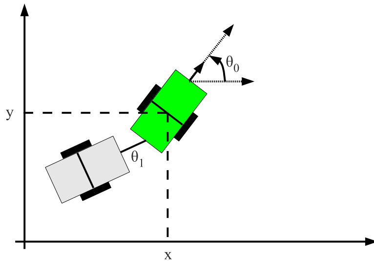
FIGURE 1.2 – Pour un robot à deux roues indépendantes tirant un chariot, les variables permettant de décrire le robot dans un environnement sont la position et l'angle \theta_0 du robot dans l'environnement, ainsi que l'angle \theta_1 entre le robot et son chariot.
