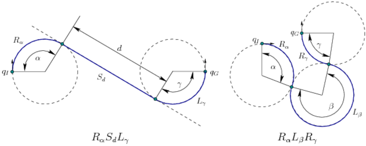
FIGURE 2.17 – Exemples de déplacements produits avec des courbes de Dubins/Reeds-Shepp, tirée de [LaValle, 2006].
