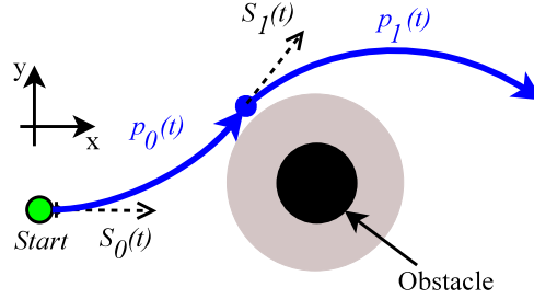
FIGURE 3.2 – Contrainte sur la continuité en vitesse et position entre deux morceaux.
