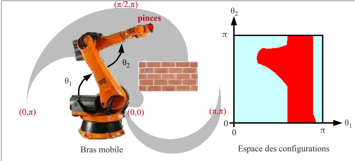
FIGURE 1.8 – Espace des configurations libres dans un exemple continu : la surface rouge illustre les configurations pour lesquelles le bras n’entre pas en collision avec l’obstacle (voir le chapitre 4 de [LaValle, 2006] pour les méthodes de calcul).
