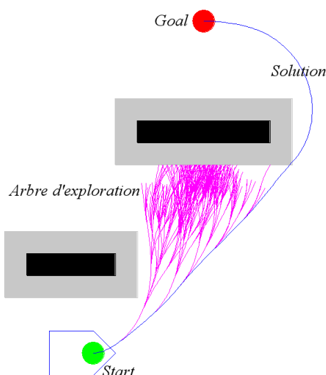
FIGURE 5.15 – Solution obtenue avec le mode backtrack de DKP sans guidage : DKP est bloqué par un minimum local qui l’empêche de trouver rapidement le franchissement de l’obstacle du haut.
