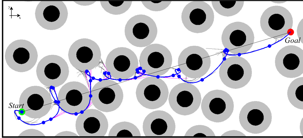
FIGURE 4.12 – Une trajectoire construite par DKP pour un robot à deux roues indépendantes contraint de tourner uniquement sur sa gauche à cause de la défaillance d'un moteur.
