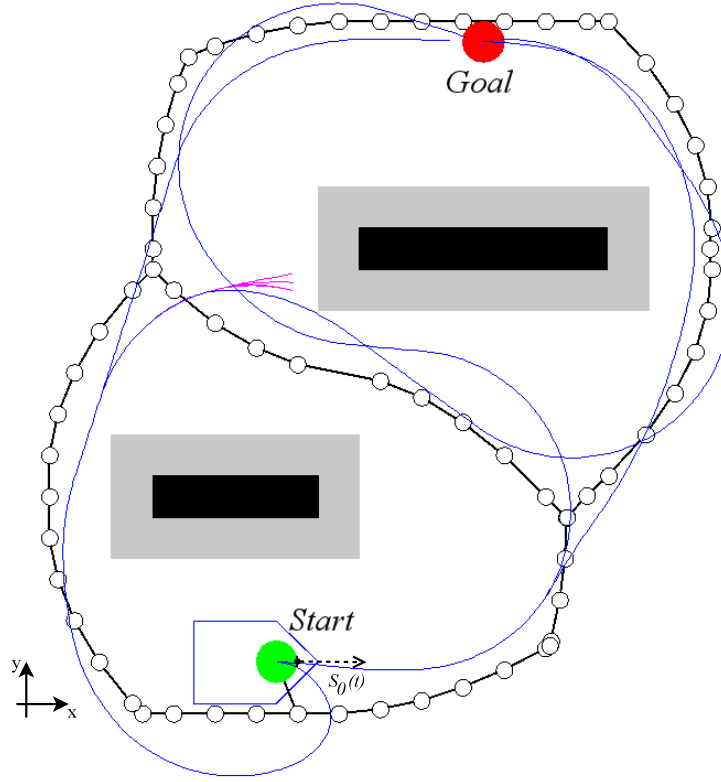
FIGURE 5.14 – Les quatre solutions obtenues avec le guidage par comportement de pilotage basé sur une roadmap.
