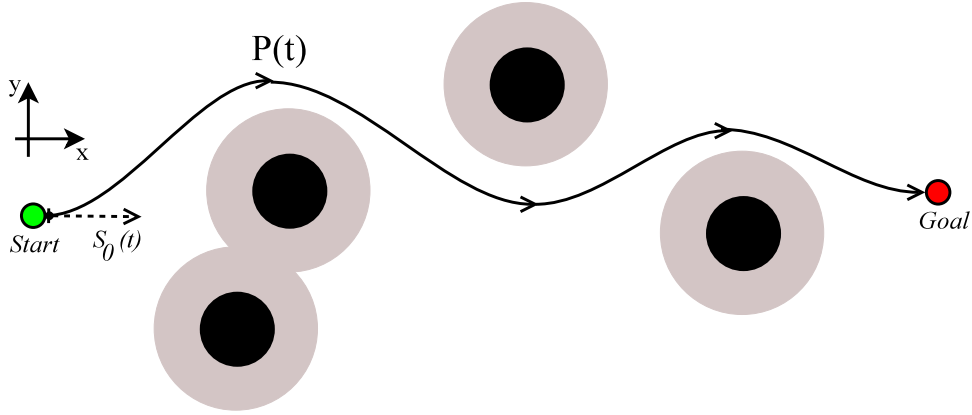
FIGURE 3.3 – Problème complet de planification de trajectoire depuis l'état de départ Start jusque l'état d'arrivée Goal .
