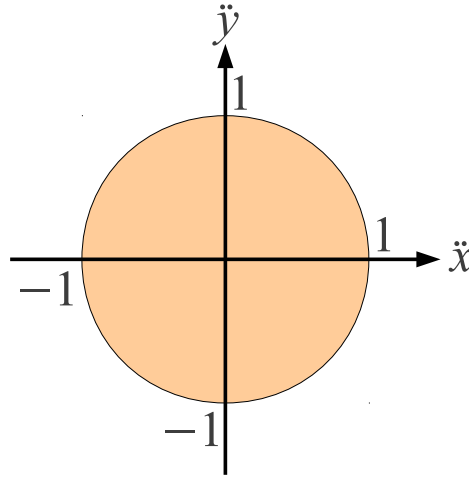
FIGURE 3.5 – Contrainte sur l'accélération linéaire bornée par [0, 1] représentée dans la base des accélérations.
