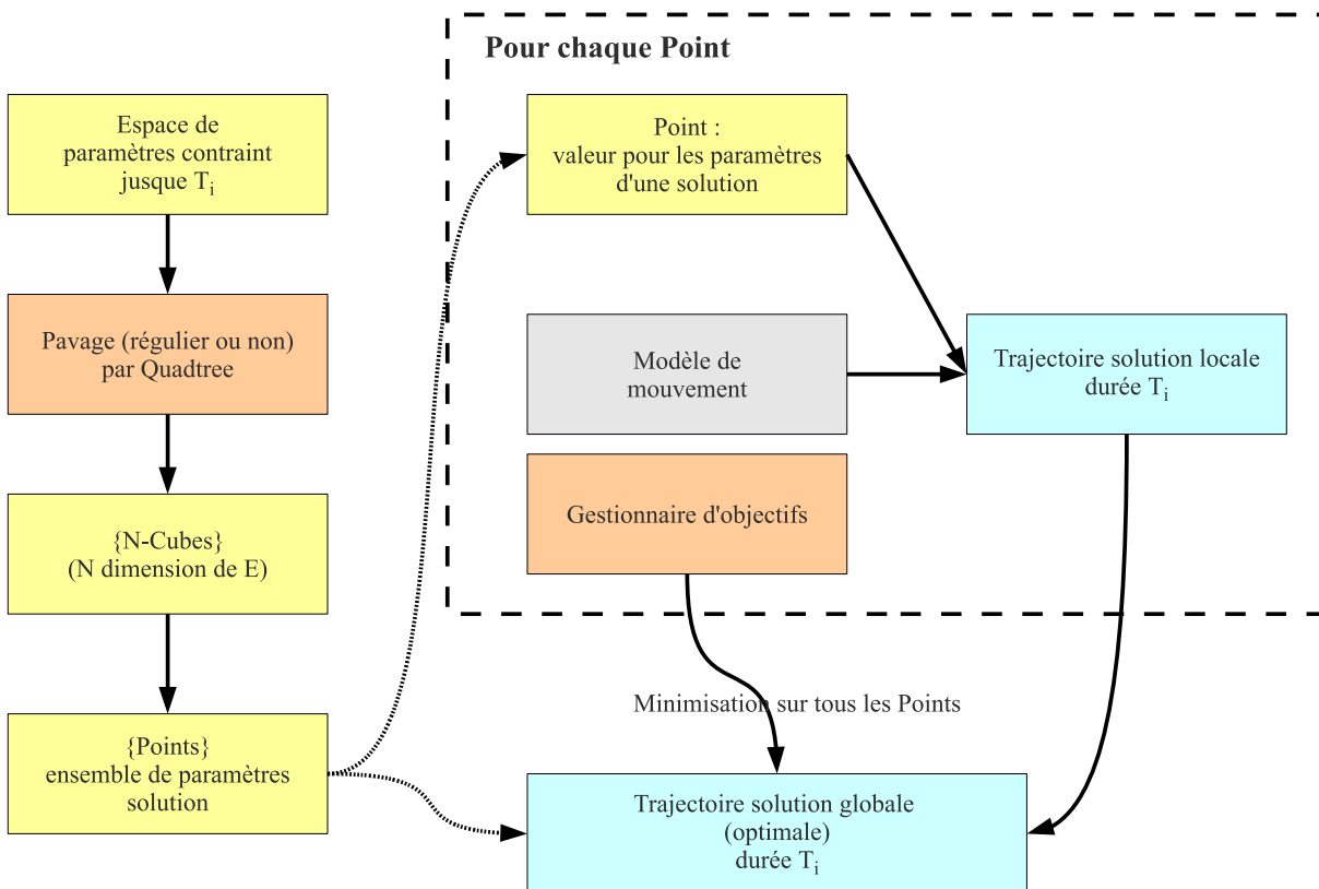
FIGURE 3.13 – Dans cette méthode de recherche de solution, l'espace des paramètres est d'abord pavé par un Quadtree. Puis de chaque pavé est tiré un ensemble de points. À partir de ces points sont générés des échantillons candidats sur lesquels est appliqué le critère de recherche afin de sélectionner la meilleure solution.
