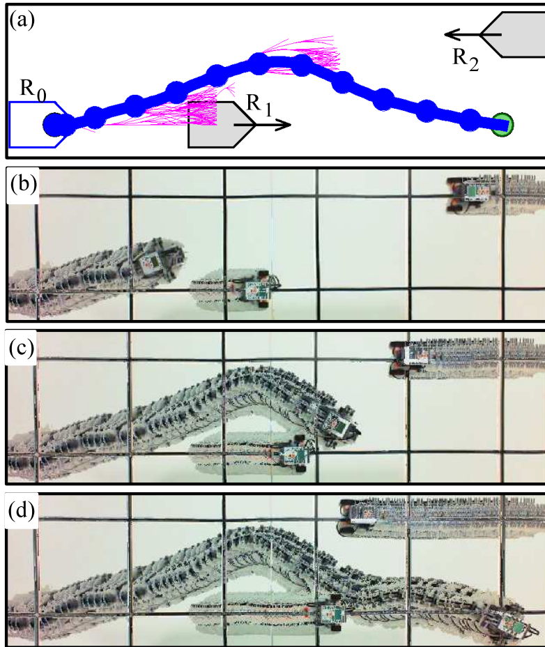
FIGURE 4.23 – Expérimentation d'un cas du dépassement d'un robot R_1 par R_0 en évitant R_2 avec (a) trajectoire planifiée appliquée au robot de (b) jusque (d).
