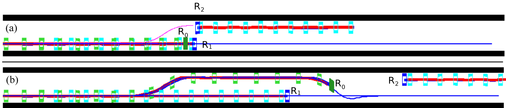
FIGURE 5.27 – Différentes situations de dépassement. (a) R_0 , en vert, ne peut pas dépasser à cause de la présence de R_2 . Il doit suivre le robot R_1 en utilisant la trajectoire en bleu. (b) R_0 peut suivre ou dépasser R_1 car le robot R_2 ne gêne pas la manœuvre : on obtient deux trajectoires alternatives en bleu. R_0 est dessiné sur celle qui dépasse
