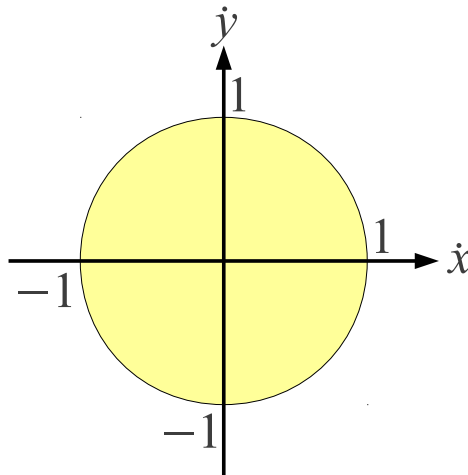
FIGURE 3.4 – Contrainte sur la vitesse linéaire bornée par [0, 1] représentée dans la base des vitesses.
