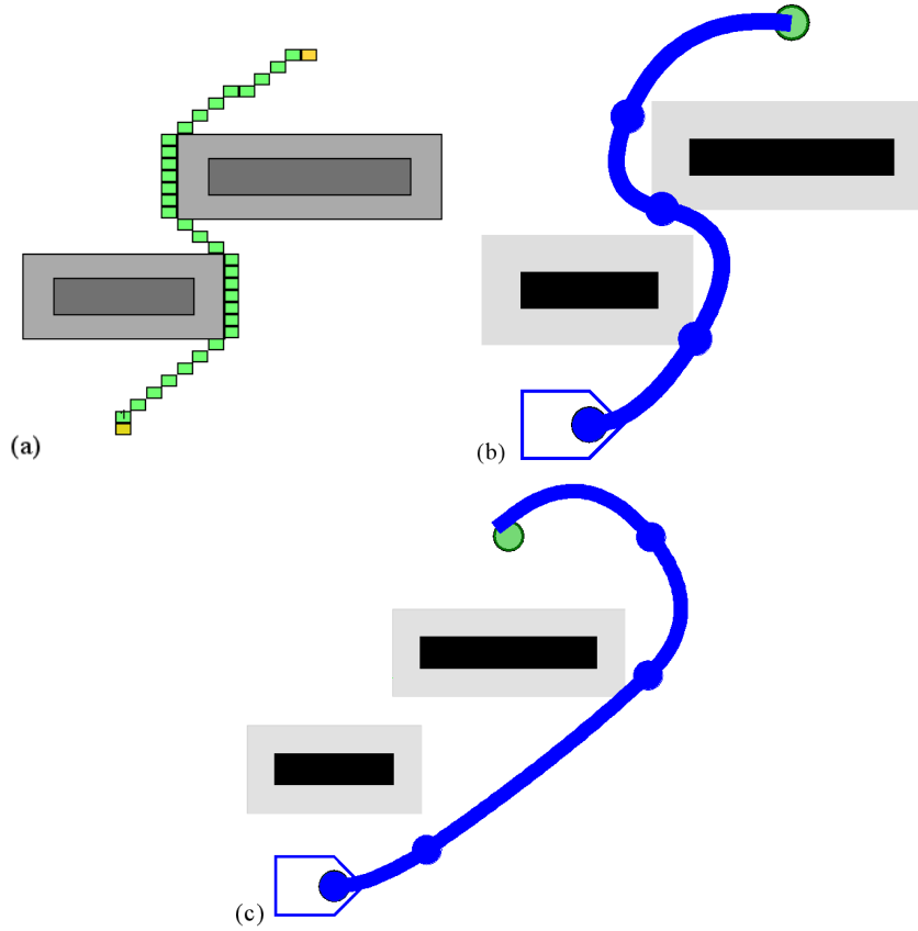
FIGURE 4.9 – Figure 4.9. Problème de planification de trajectoire (obstacles en gris). Le robot possède une borne inférieure sur sa vitesse linéaire et supérieure sur sa vitesse angulaire. (a) Solution trouvée par Dijkstra (grille 50x50). Cette solution sera toujours fournie quel que soit le modèle du robot. Elle ne sera donc pas nécessairement réalisable. (b) Solution trouvée par DKP pour une vitesse angulaire maximale élevée et (c) pour une vitesse angulaire maximale faible.
