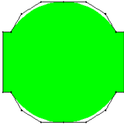
FIGURE 7.6 – L'union d'un disque avec un rectangle.
