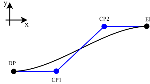
FIGURE 7.3 – Une cubique et son polygone de contrôle.
