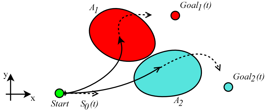
FIGURE 5.3 – Mécanisme de propagation permettant le guidage local de DKP : lorsqu’il propage des morceaux de trajectoire dans une partie A_k de l’environnement, les morceaux sont optimisés en direction de l’objectif associé à cette surface A_k .
