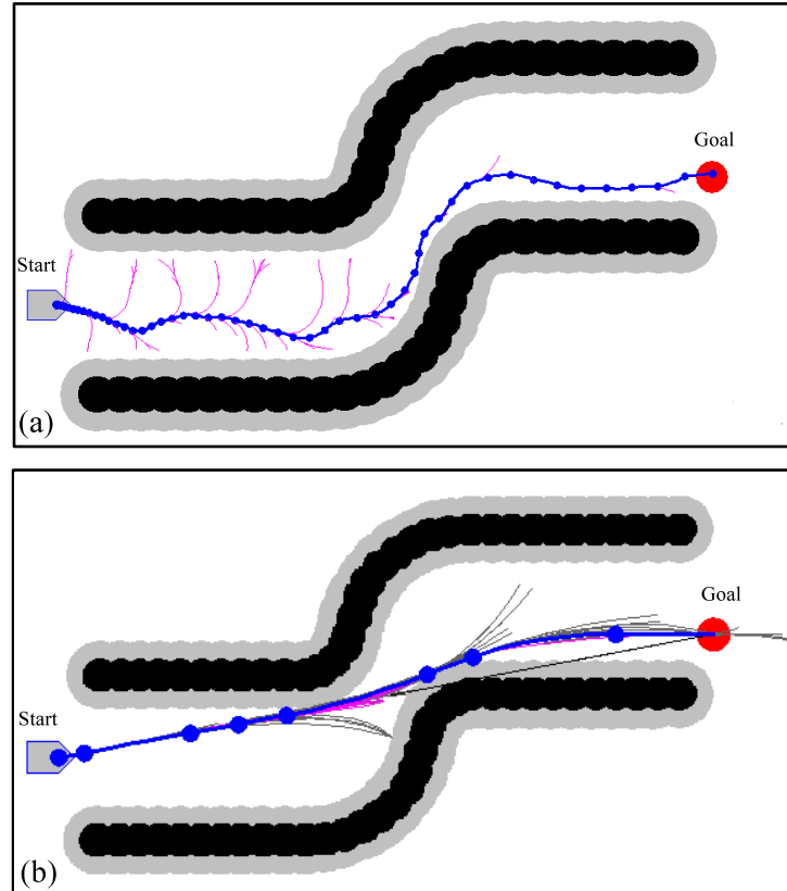
FIGURE 4.10 – Échantillons et trajectoires finales obtenues par (a) RRT et (b) DKP. Les trajectoires finales apparaissent en gras : (a) la longueur de la trajectoire est de 9.04m, sa durée est de 12.6s. Cette solution est obtenue par RRT en 67s. (b) la longueur de la trajectoire est de 8.19m, sa durée est de 3.2s. Cette solution est obtenue par DKP en 27.6s.
