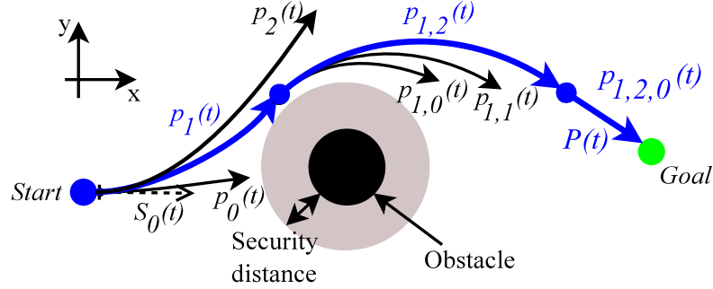
FIGURE 4.4 – DKP construit des trajectoires splines depuis Start jusqu'à Goal avec des échantillons p_{k_0 \dots k_n}(t) organisés dans un arbre d'exploration. La distance de sécurité prend en compte l'empattement du robot
