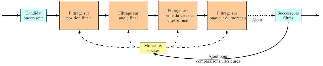
FIGURE 4.6 – Le filtrage s’insère entre la couche de propagation et l’ajout des morceaux à prolonger dans l’ensemble des ouverts afin de limiter la taille de l’arbre d’exploration et donc la complexité générale de DKP.
