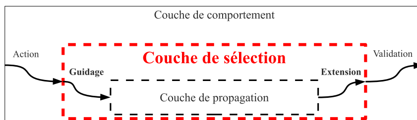
FIGURE 4.2 – Architecture retenue pour exprimer des comportements de pilotage pour la planification de trajectoire sous contraintes cinématiques. Ce chapitre se focalise sur le niveau de sélection et ses interactions avec la couche de propagation
