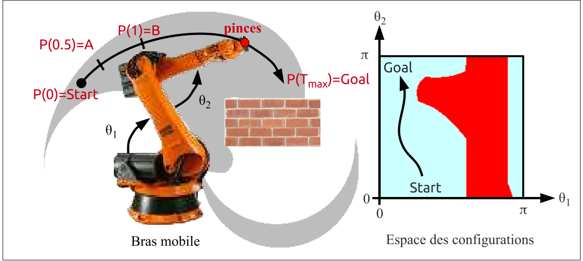
FIGURE 1.13 – Illustration d'une trajectoire planifiée dans l'espace des configurations et sa conséquence sur la position des pinces dans l'espace de travail.
