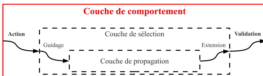
FIGURE 5.2 – Architecture retenue pour exprimer des comportements de pilotage dans le cadre de la planification de trajectoire sous contraintes. DKP assure la vérification de ces dernières tandis que les comportements de pilotage régulent le comportement de DKP.
