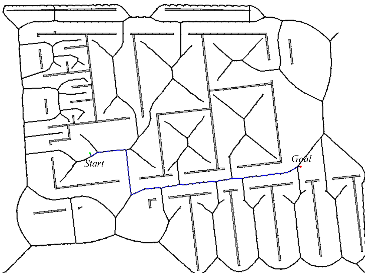
FIGURE 5.21 – Une roadmap issue de la simplification du diagramme de Voronoï (les lignes grises épaisses) sur les plans de l'ISEN. Le chemin optimal en distance sur la roadmap est représenté en bleu.
