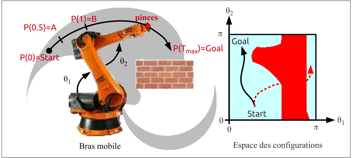
FIGURE 1.15 – Trajectoire planifiée dans le cas continu : le bras ne peut se déplacer qu'à une vitesse continue et finie dans l'espace de travail.
