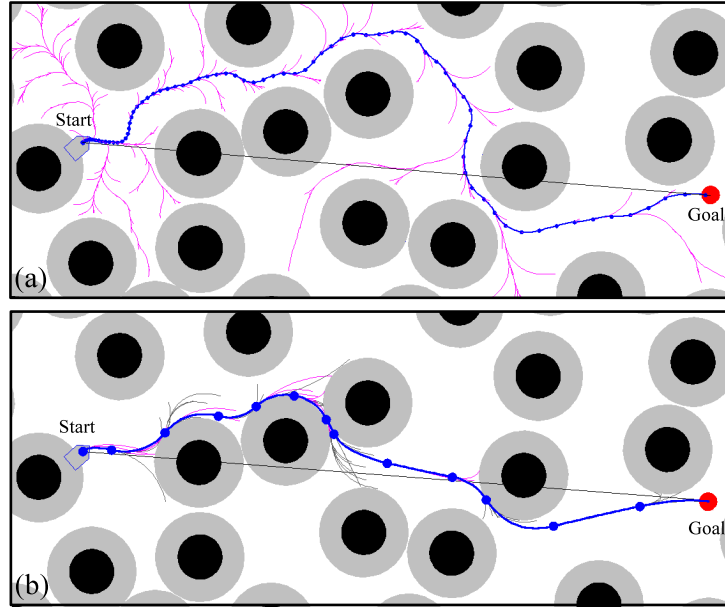
FIGURE 4.11 – Échantillons et trajectoires finales obtenues par (a) RRT et (b) DKP. Les trajectoires finales apparaissent en gras : (a) la longueur de la trajectoire est de 19.44m, sa durée est de 18.51s. Cette solution est obtenue par RRT en 168s. (b) la longueur de la trajectoire est de 16.41m, sa durée est de 18s. Cette solution est obtenue par DKP en 13.7s.
