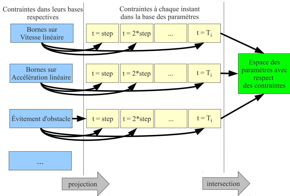
FIGURE 3.8 – Première méthode de construction de l'espace des paramètres : chaque contrainte est projetée dans la base des paramètres pour chaque pas de planification. L'intersection de l'ensemble ainsi obtenu avec l'espace des paramètres permet de retirer progressivement les n-uplets de paramètres qui ne respectent pas les contraintes du problème.
