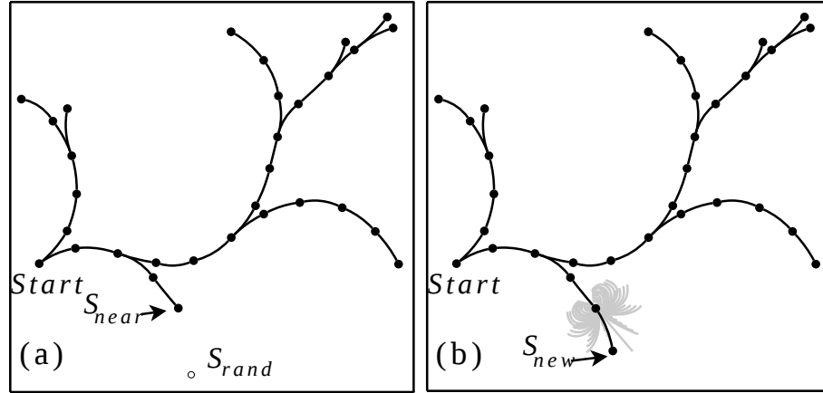
FIGURE 2.18 – Exploration de l'espace des états avec RRT. Après tirage aléatoire d'une configuration S_{rand} (a) le niveau de sélection choisit un nœud S_{near} pour son expansion; (b) le couche de propagation génère un nœud suivant valide S_{new} .
