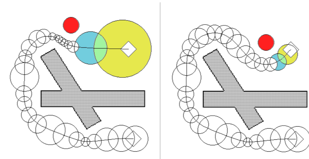
FIGURE 2.13 – Illustration provenant de [Quinlan et Khatib, 1993] montrant la déformation d'un chemin grâce aux forces créées par le déplacement d'un obstacle en rouge. Ces forces déplacent les bulles disposées sur le chemin : la déformation est acceptable tant que les bulles voisines, par exemple celles en couleur, partagent une partie commune.
