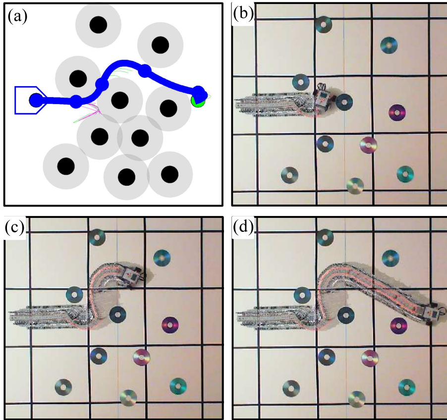
FIGURE 4.21 – Expérimentation dans un environnement chargé d'obstacles avec (a) trajectoire planifiée appliquée au robot de (b) jusque (d).
