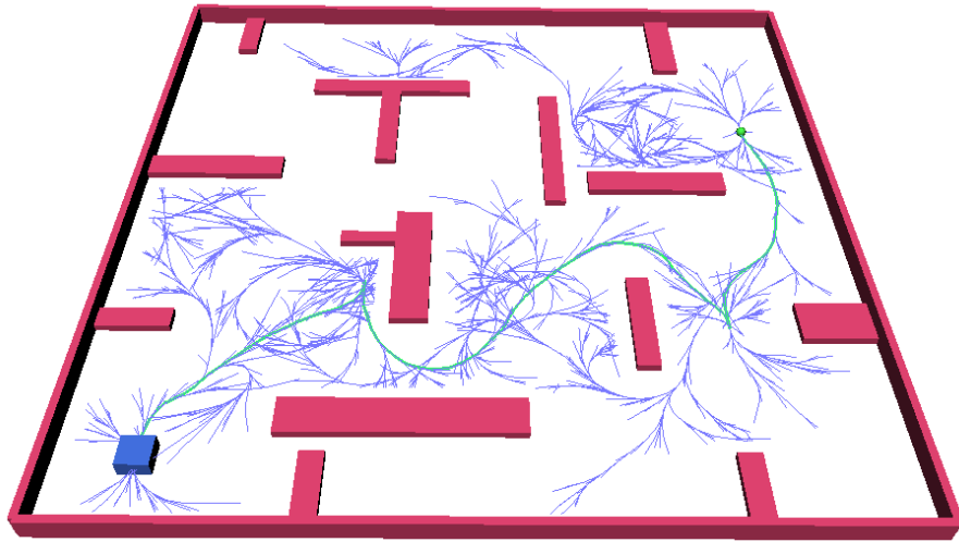
FIGURE 2.19 – RRT étend un arbre d'exploration dans l'espace des positions atteignables. Il est prouvé que les processus aléatoires de propagation et de sélection des morceaux à prolonger permettent d'obtenir nécessairement une solution (éventuellement en réitérant la planification).
