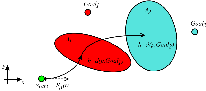
FIGURE 5.4 – Mécanisme de sélection permettant l’optimisation du choix des morceaux à prolonger : lorsque DKP propage des morceaux de trajectoire dans une partie A de l’environnement, les morceaux qui occupent cette surface propagent des scores qui sont fonction de la distance entre la fin du morceau et l’objectif associé à A .
