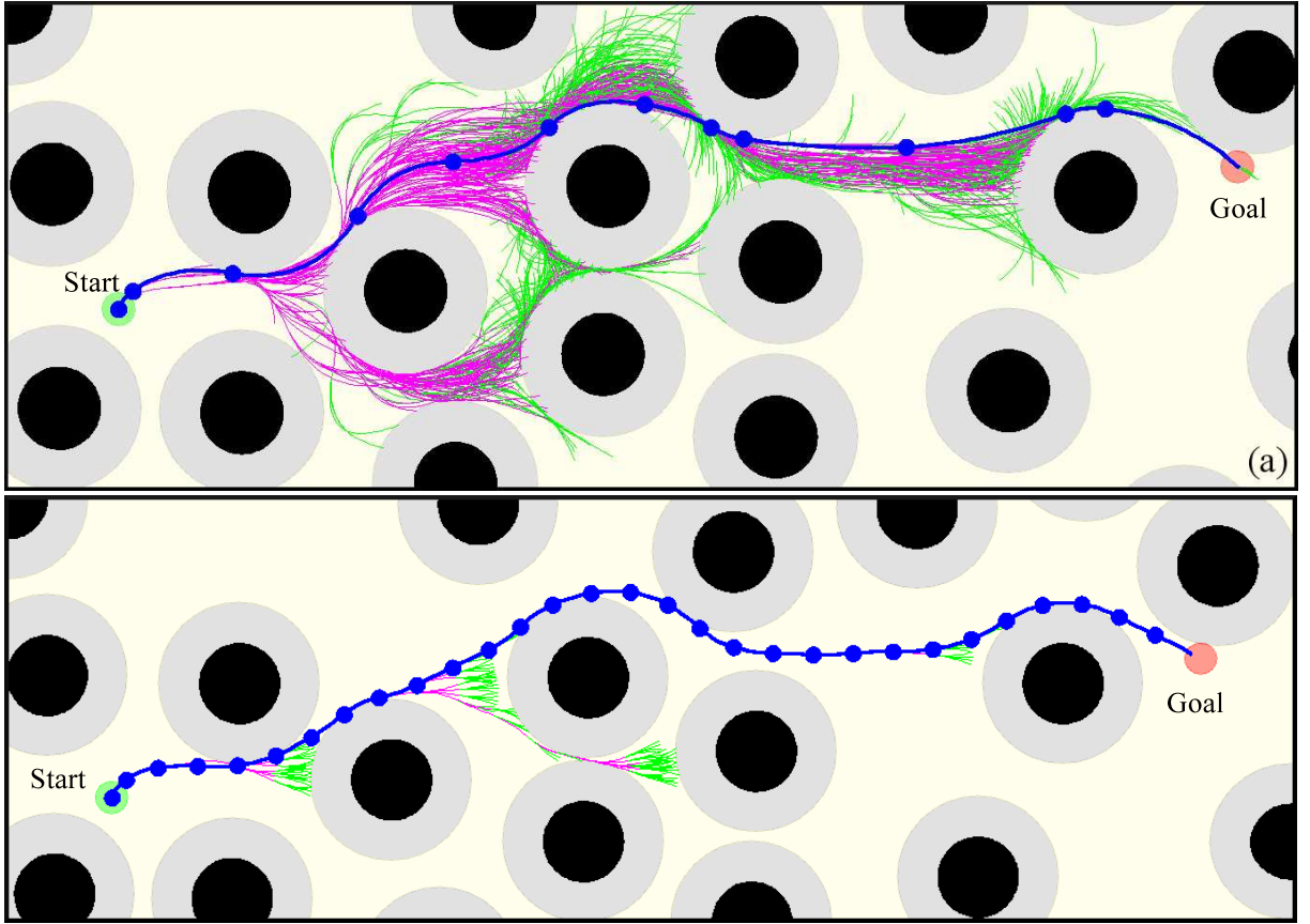
FIGURE 4.13 – Arbre d'exploration de trajectoire pour (a) une recherche en mode optimal et (b) une recherche en mode backtrack.
