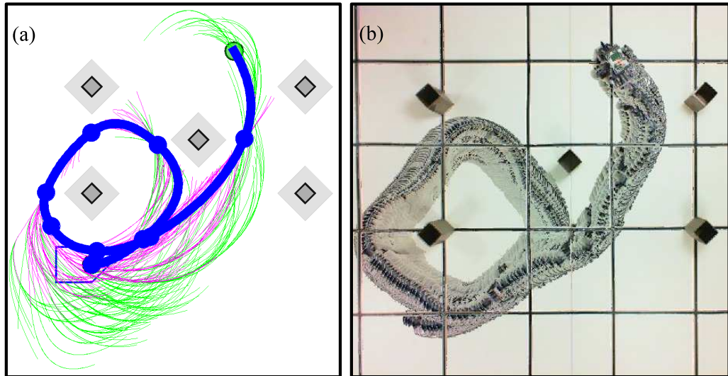
FIGURE 4.22 – Expérimentation d'une situation où le robot est confronté à une panne avec en (a) trajectoire planifiée appliquée au robot en (b).
