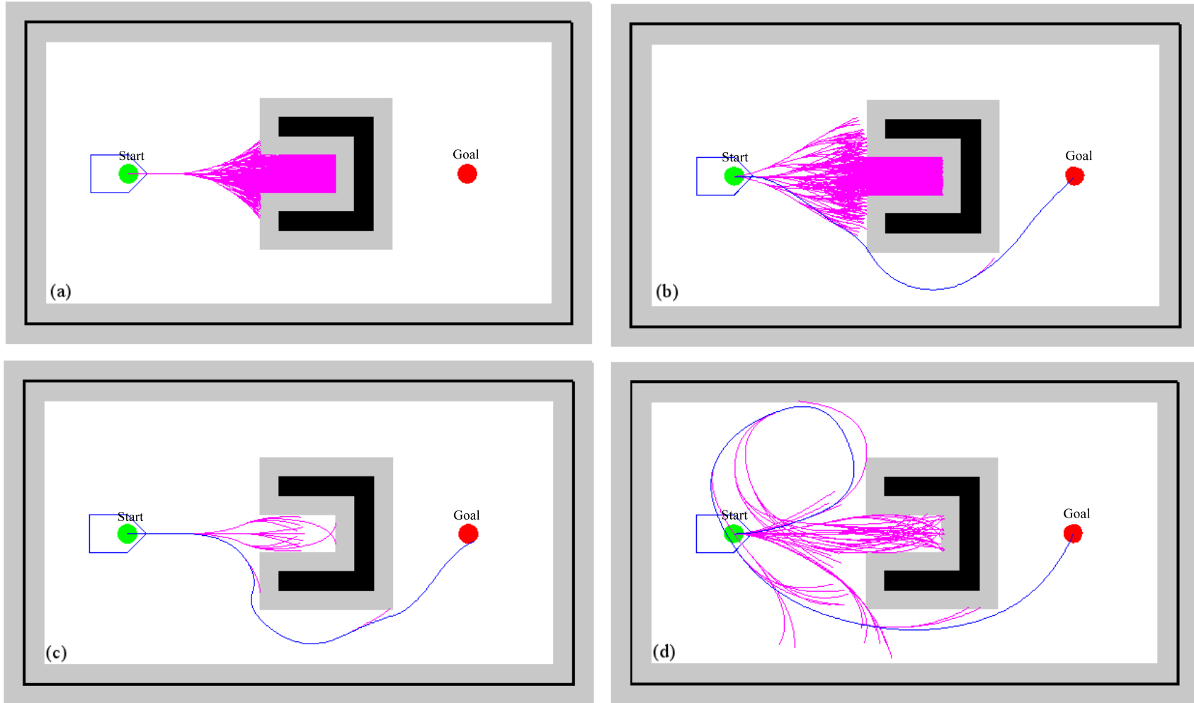
FIGURE 4.14 – DKP en mode backtrack sur le problème de l'obstacle en U montrant : (a) l'exploration interrompue avec des échantillons de 0.5s ; (b) l'arbre d'exploration et la solution avec des échantillons de 1s ; (c) l'arbre d'exploration et la solution avec des échantillons de 2s ; (d) l'arbre d'exploration et la solution avec des échantillons de 4s avec une manœuvrabilité limitée.
