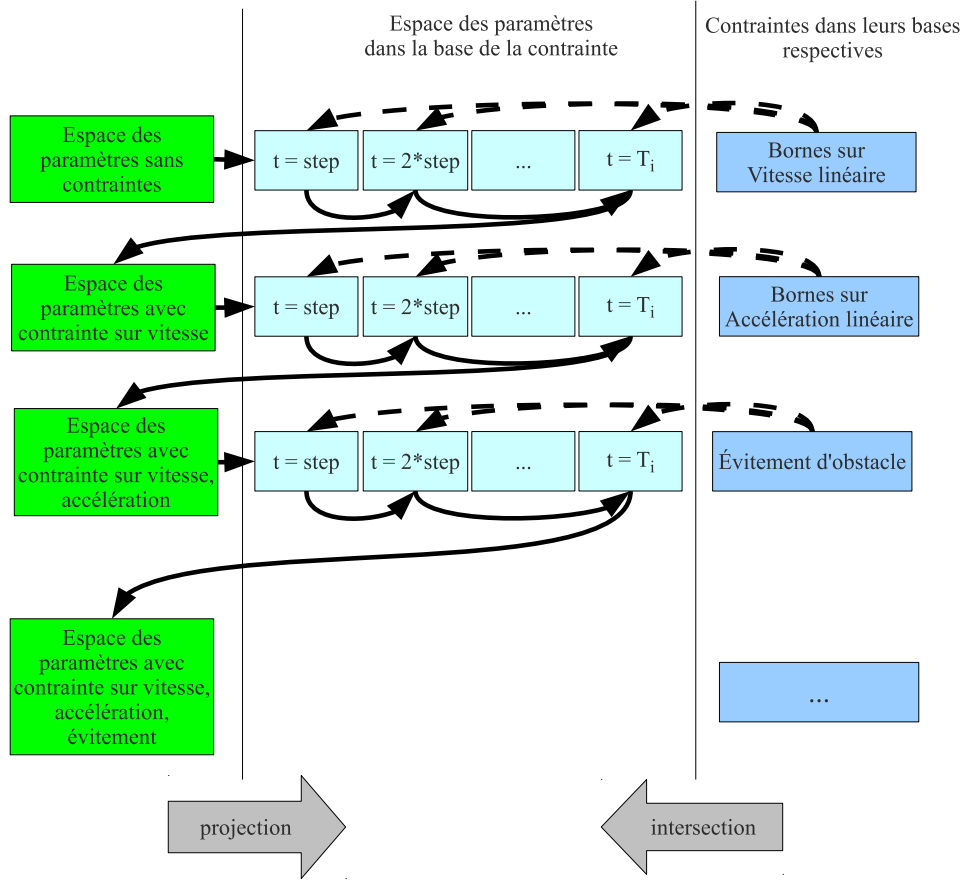
FIGURE 3.9 – Seconde méthode de construction de l’espace des paramètres : l’espace des paramètres est projeté dans la base de chaque contrainte pour chaque pas de planification. L’intersection de l’ensemble ainsi obtenu avec l’ensemble de valeurs admissibles de chaque contrainte permet de ne conserver dans l’espace des paramètres que les valeurs qui respectent les contraintes.
