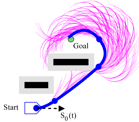
FIGURE 5.9 – Rappel de la trajectoire obtenue par DKP sur le problème de franchissement avec le respect de contraintes de vitesse et d'accélération linéaire.
