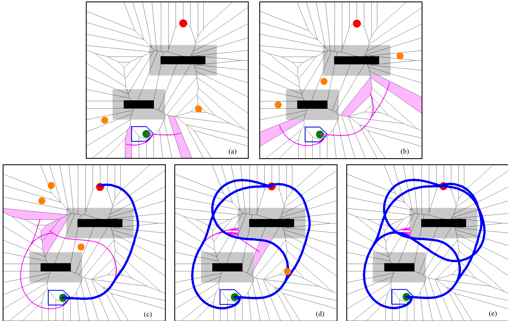
FIGURE 5.17 – L’arbre de trajectoires guidé par l’arbre de pilotage de la Figure 5.16. Les courbes bleues représentent les trajectoires alternatives qui atteignent l’objectif. Les courbes en magenta sont des échantillons de trajectoire en cours de construction ou abandonnés. Les polygones en rose clair correspondent aux surfaces où les trajectoires en construction poursuivent à cet instant leur progression. Les points oranges sont associés aux objectifs intermédiaires, fournis par l’arbre de trajectoires
