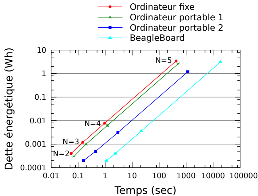
FIGURE 8.2 – Dette énergétique de l’algorithme sur différents équipements. La dette énergétique de l’algorithme diffère suivant l’équipement cherchant le plan de répartition optimisé. De même le temps de calcul diffère d’un équipement à un autre.
