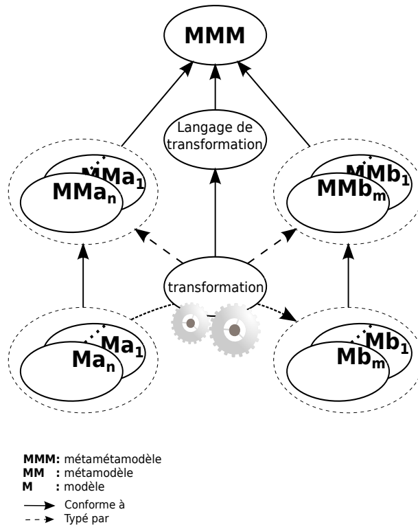
FIGURE 13: Relation entre les transformations de modèles et les modèles (modèle, métamodèle et métamodèle)
