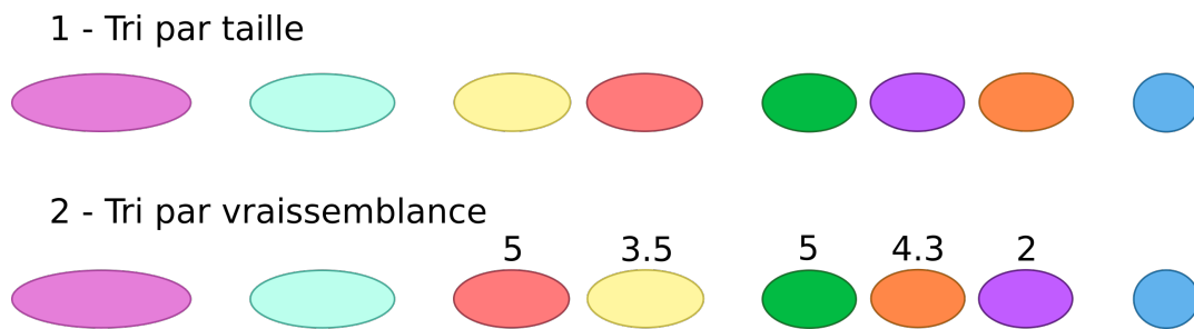
Figure 2.29: Tri pour le pavage glouton. Les résidus sont triés par taille puis par vraisemblance.
