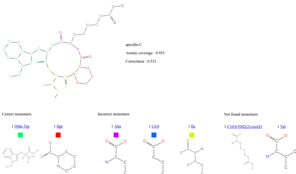
Figure 2.35: Le résultat HTML de l'exécution de s2m sur l'apicidine C
