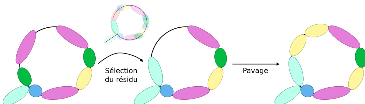
Figure 2.30: Représentation d’une étape de modulation. La première transition se fait par l’ajout forcé d’un résidu non choisi lors du pavage et de la suppression de tous les résidus le chevauchant. La seconde transition est effectuée par une étape de pavage glouton sur les zones non couvertes du peptide. Si une modulation ne suffit pas, cette étape est répétée de multiples fois au sein d’un algorithme de backtracking.
