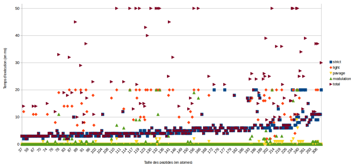
Figure 2.40: Temps d'exécution de s2m pour un extrait aléatoire de 350 molécules. Les données ont été tronquées au delà de 50ms pour ne pas écraser le graphique.
