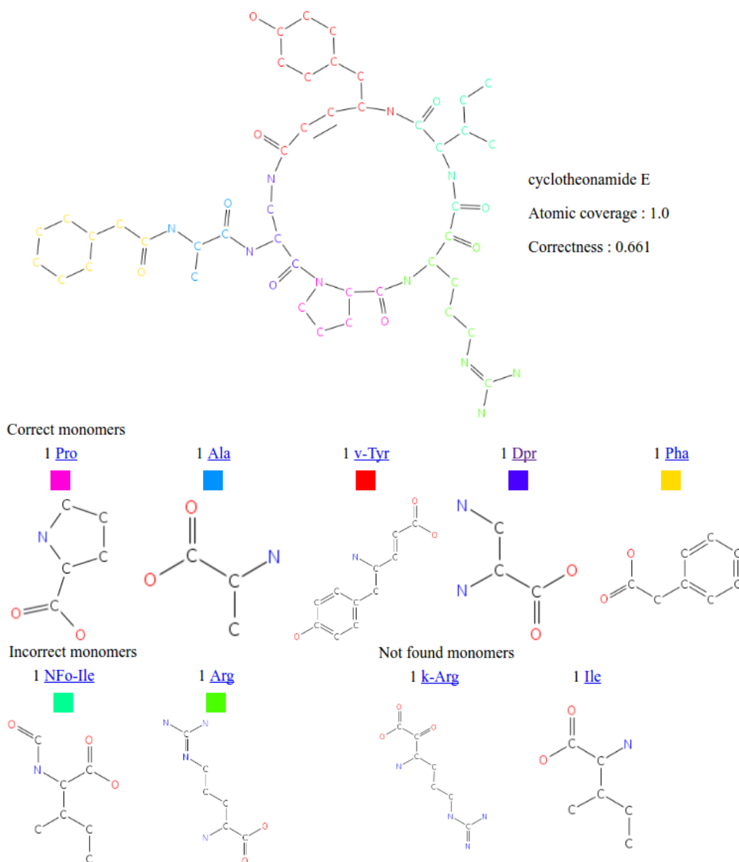
Figure 2.45: Résultat de s2m pour la Cyclotheonamide E (peptide de Norine). L'annotation monomérique recouvre l'entièreté des atomes du peptide mais n'est pas correcte à cause d'une équivalence entre monomères.
