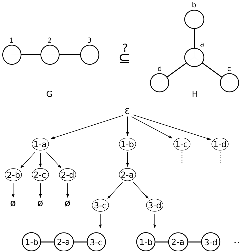
Figure 2.13: Backtracking de VF2 pour extraire l'ensemble de tous les SI possibles.
