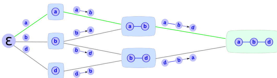
Figure 2.19: Ensemble des chaînes générées à partir du motif a-b-d avec en vert le chemin pris par l'algorithme glouton.
