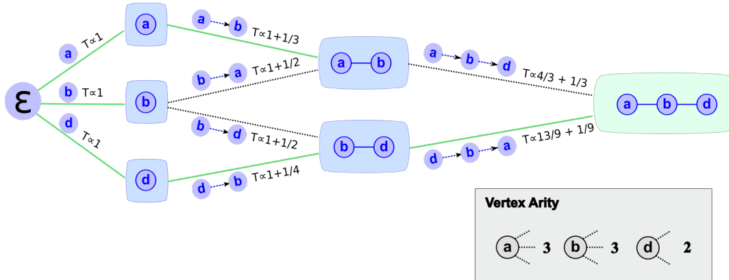
Figure 2.21: En vert, les chemins pris par la programmation dynamique pour finalement obtenir le chemin optimal vers le motif a-b-d. Il est également possible de rechercher le chemin optimal en utilisant l'algorithme de Dijkstra mais la mise en place des structures de données nécessaires ralentiraient le calcul pour de petites données. Comme nous le verrons en section 2.5.3.1, nous ne calculerons jamais de grandes chaînes exactes sur nos données (chaînes exactes de taille 3 en général).
