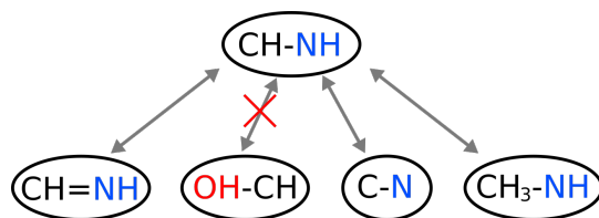
Figure 2.32: Exemple d'application de la fonction de matching lighth d'étiquettes. Puisque le nombre d'atomes d'hydrogène n'est plus un critère sélectif et que l'arité de la liaison chimique non plus, la comparaison est valide dès que les deux atomes non hydrogène sont identiques.
