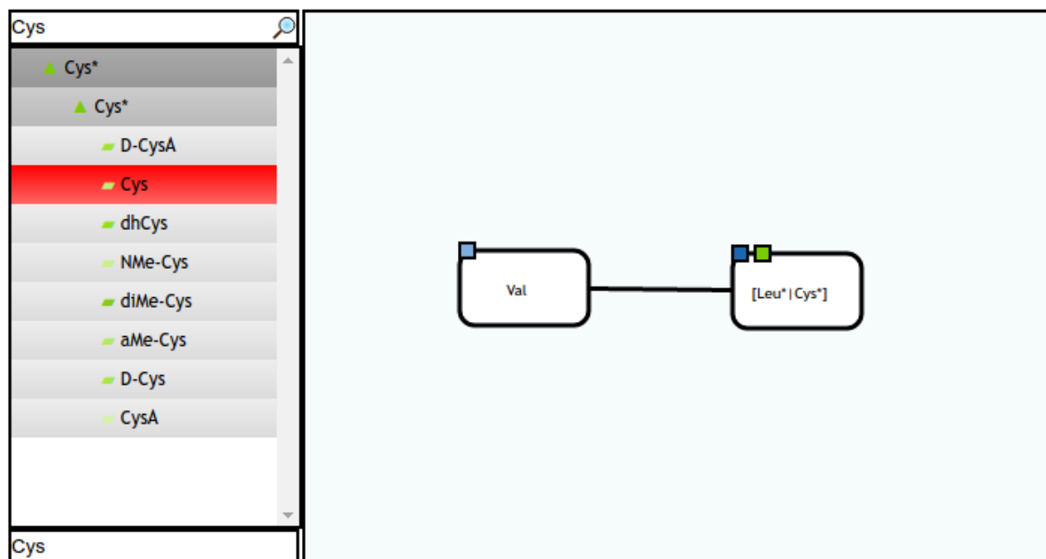
Figure 3.4: Éditeur graphique pour la construction de requêtes dans Norine. Ici, nous avons construit graphiquement la requête Val,[Cys*|Leu*]@1@0 .
