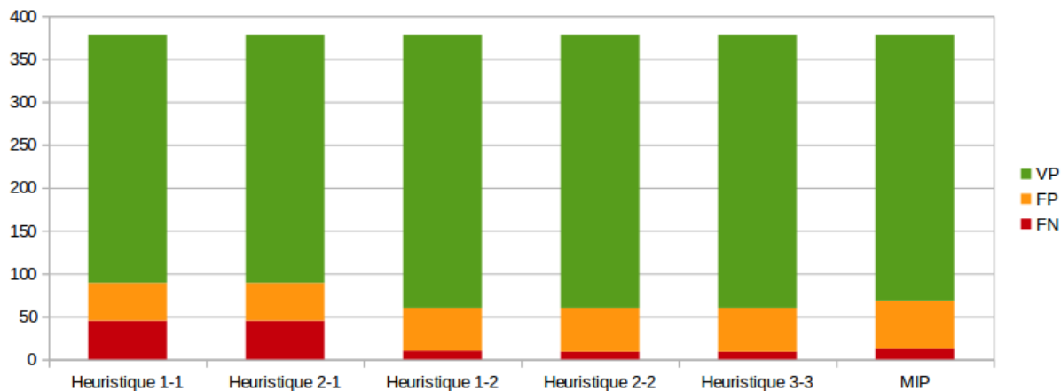
Figure 2.38: Diagramme en barre des résultats sur CCD
