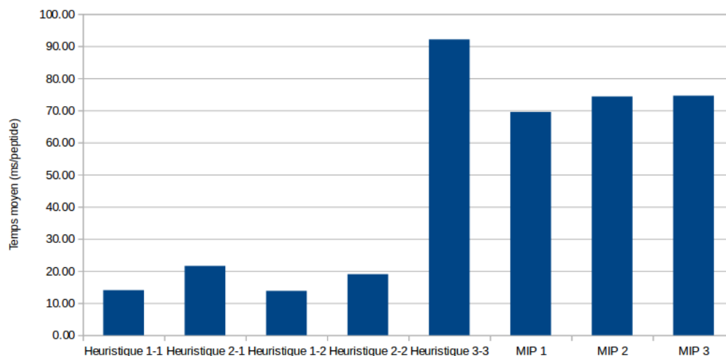
Figure 2.39: Temps d'exécution moyen par peptide (en ms) en utilisant les deux pavages et différents paramètres pour chacun d'eux.
