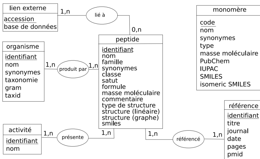
Figure 3.1: Schéma simplifié de la base de données Norine. Figure extraite de la thèse de Ségolène Caboche avec son accord.
