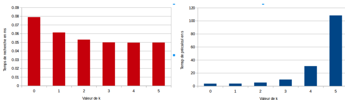
Figure 2.36: Évaluation de l'efficacité d'apprentissage des chaînes sur l'ensemble des monomères des deux jeux de données. À gauche : représentation du temps de recherche moyen d'une chaîne dans un peptide selon k . À droite : temps d'apprentissage pour tous les monomères selon k .
