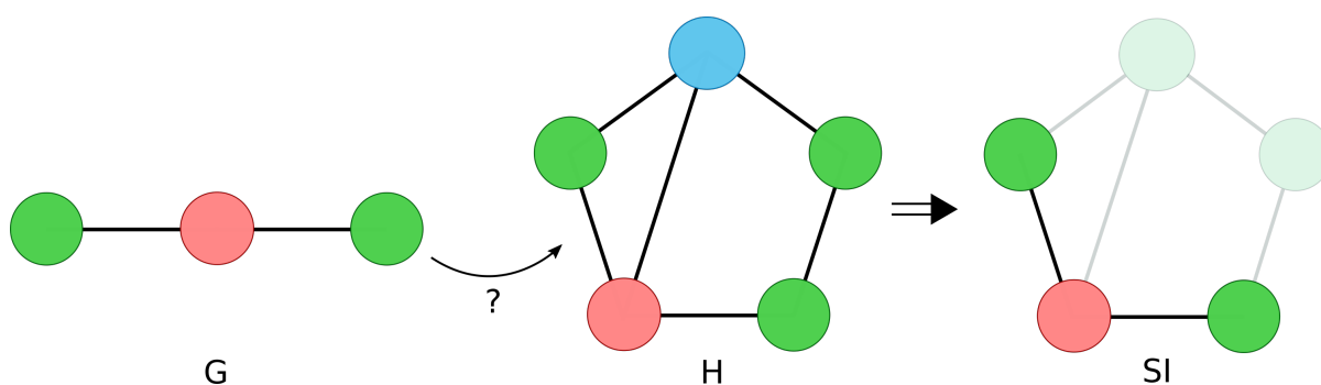
Figure 2.11: SI obtenu à partir de la recherche du graphe G dans H. Sur cet exemple, il n'y a qu'une seule possibilité mais si nous avions cherché une chaîne comme Vert-Rouge-Bleu, nous aurions obtenu deux SI différents.
