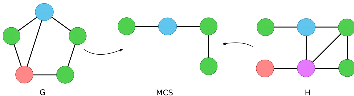
Figure 2.8: MCS obtenu à partir des graphes G et H. Le MCS obtenu ne contient pas le nœud étiqueté “rouge” du fait des liens vers ce nœud qui ne sont pas les mêmes dans G et H.
