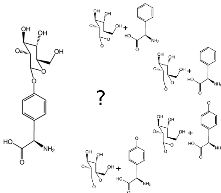
Figure 2.5: Dans le cas de ce dimère, un sucre est lié à une Hydroxy-Phenil-Glycine (Hpg). En utilisant la règle de découpe à appliquer pour les liaisons hydroxyle, une ambiguïté et une erreur apparaissent. Nous ne pouvons savoir de quel côté les découpes vont être les plus pertinentes avant d'essayer de reconnaître les monomères. De ce fait, 4 découpes différentes sont possibles. De plus, le cycle du sucre se voit ouvert alors que la découpe est inutile.
