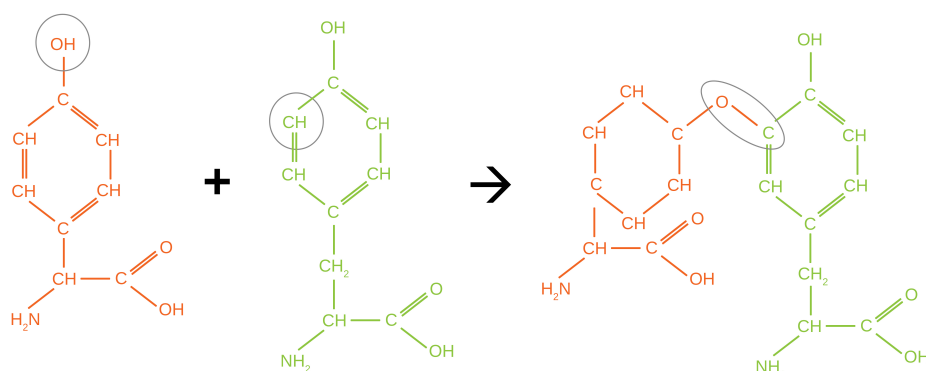
Figure 1.6: Exemple de liaison effectuée au sein d'un cycle benzène
