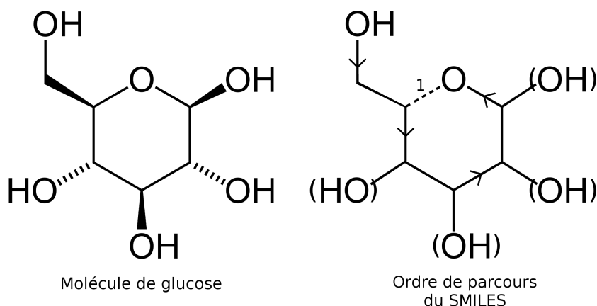
Figure 4: Molécule de glucose et son ordre de parcours dans le SMILES cyclique exemple.
