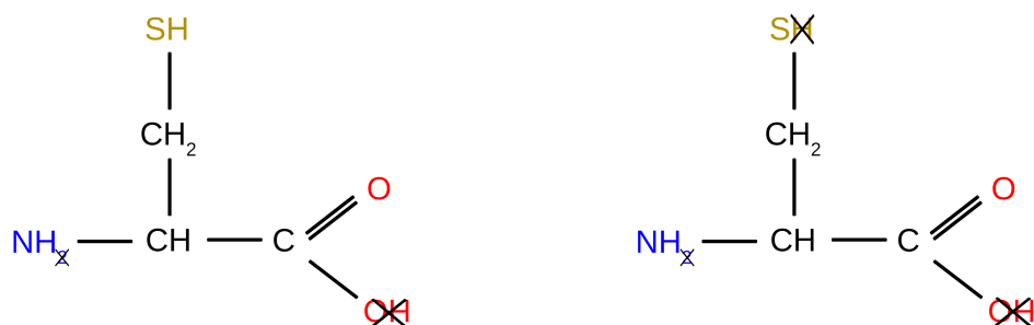
Figure 2.22: Deux résidus différents présents dans deux peptides différents tous deux obtenus à partir de la Cystéine
