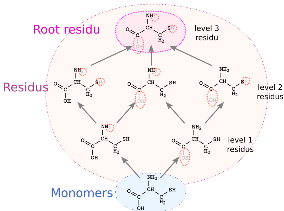
Figure 2.23: Représentation de la construction de la famille des résidus de la cystéine.
