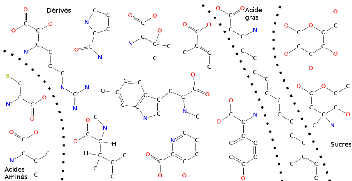
Figure 1.3: Patchwork de monomères NRP. De gauche à droite : deux représentants des acides aminés classiques ; plusieurs dérivés d'acides aminés ; un acide gras ; deux sucres.
