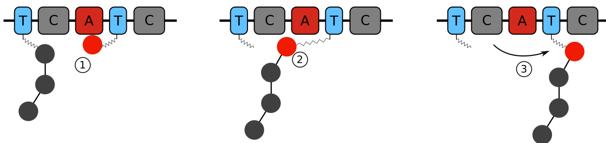
Figure 1.10: Rôle du domaine T au sein d'une NRPS. 1 - Liaison entre le monomère capturé par le domaine A et le bras du module T. 2 - Liaison entre le monomère et la chaîne peptidique en cours d'élongation. 3 - Déplacement du peptide vers le domaine C suivant
