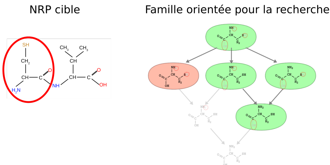
Figure 2.24: Représentation de la recherche de la cystéine dans un di-peptide, en utilisant sa famille de résidus. En vert, les résidus trouvés dans le NRP cible, en rouge ceux non trouvés et en transparent, les non cherchés.
