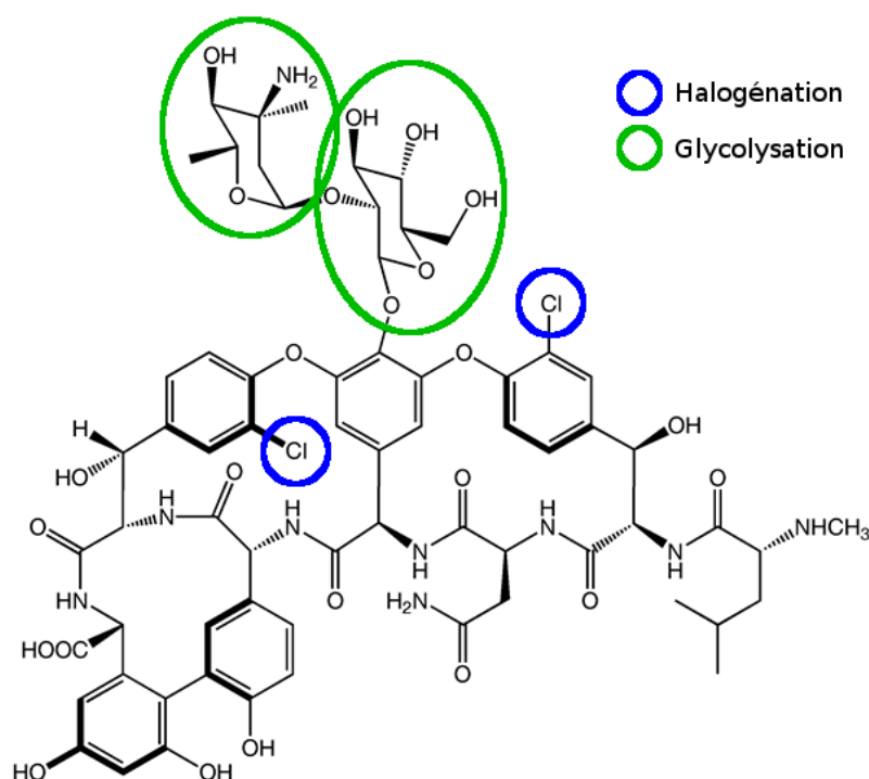
Figure 1.15: Modifications post-synthèse NRP pour la vancomycine
