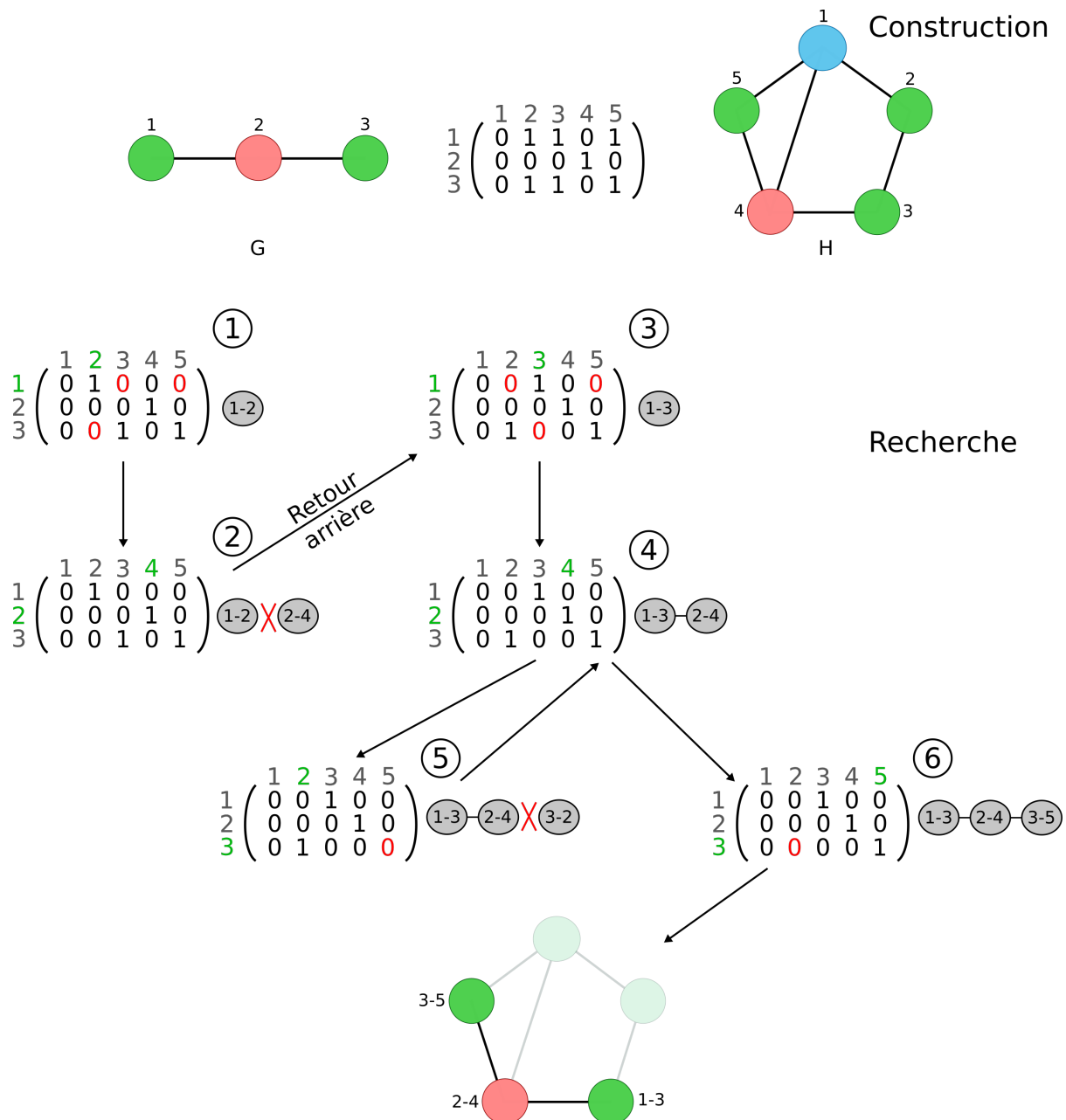
Figure 2.12: Recherche d'un isomorphisme de sous-graphe par l'algorithme d'Ullman. Dans la partie "construction", vous pouvez voir la matrice créée à partir des graphes G et H. Dans la partie "recherche" sont présentées les étapes successives de création d'un SI (voir le texte pour les détails). Si nous avions voulu obtenir tous les isomorphismes (et pas juste un seul), il aurait fallu continuer le backtracking jusqu'au bout.
