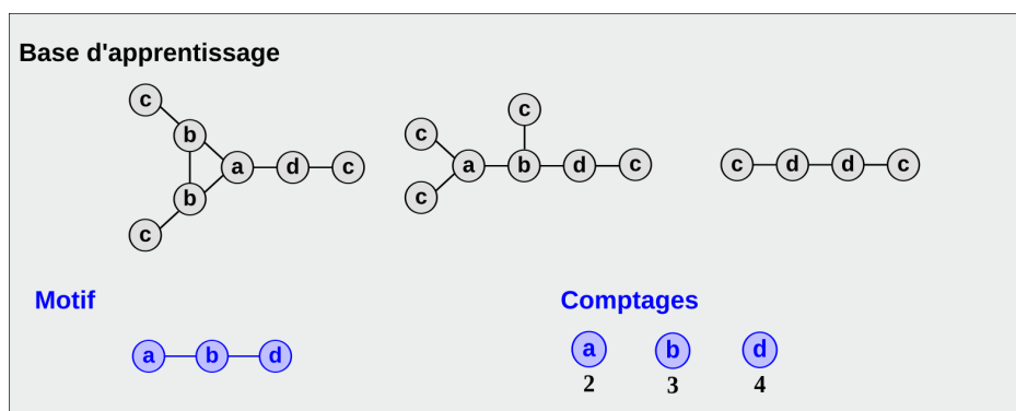
Figure 2.18: En haut de l’image est représentée la base d’apprentissage puis en bas, le motif qui doit être indexé ainsi que les fréquences d’apparition de chacun de ses nœuds dans la base d’apprentissage
