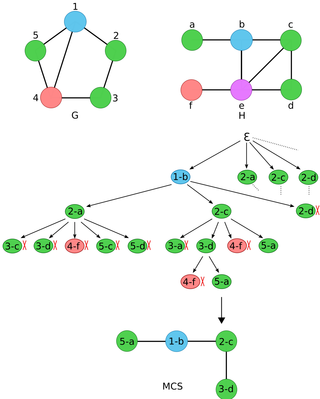
Figure 2.10: Exemple de résolution de MCS par un backtracking naïf. L'arbre part d'une bijection vide et ajoute un couple à chaque étape. Parfois l'algorithme tombe sur un couple compatible mais dont les voisins ne sont pas présents dans la bijection. La solution est alors rejetée (croix rouge). La solution est trouvée par l'ensemble des chemins qui mènent aux feuilles valides les plus profondes dans l'arbre.
