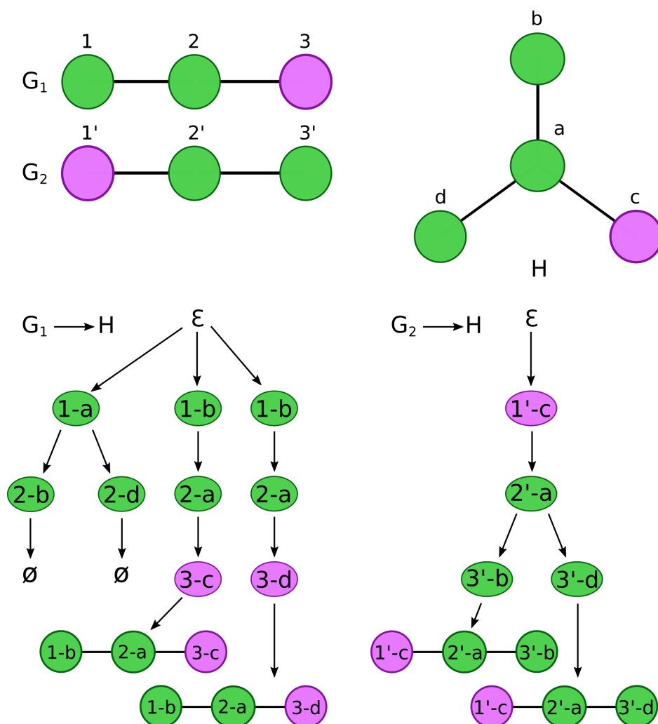
Figure 2.14: Modification de VF2 pour son application aux graphes étiquetés. On voit nettement sur cet exemple que l'ordre de recherche des étiquettes influence le temps d'exécution de l'algorithme.
