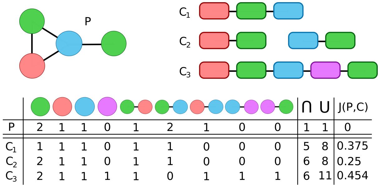
Figure 3.13: Exemple de calcul de distance entre un peptide P et trois clusters de gènes C_1 , C_2 et C_3 . Les clusters de gènes sont représentés par une suite de modules colorés en fonction de la couleur du monomère qui sera inclus. Dans le tableau sont présents les différents fingerprints pour le monomère et les clusters accompagnés du calcul de la distance de Jaccard.
