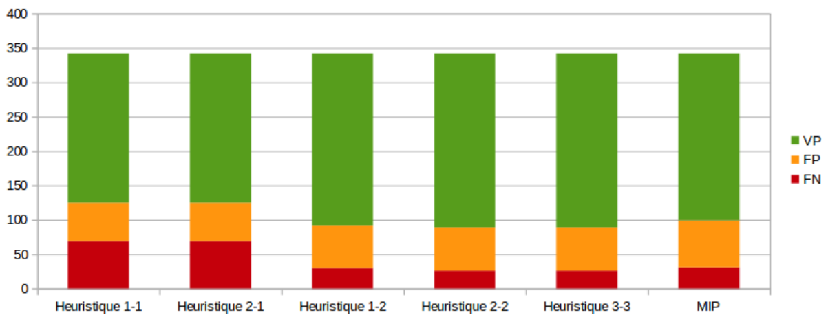
Figure 2.37: Diagramme en barre des résultats sur Norine
