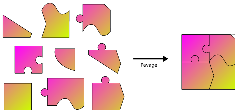
Figure 2.25: Phase de pavage. Choix parmi toutes les pièces disponibles pour former le puzzle le plus grand possible
