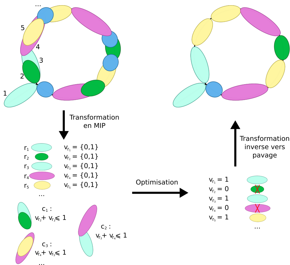
Figure 2.28: Représentation globale de la réduction du problème de pavage en MIP puis reconstruction de la solution
