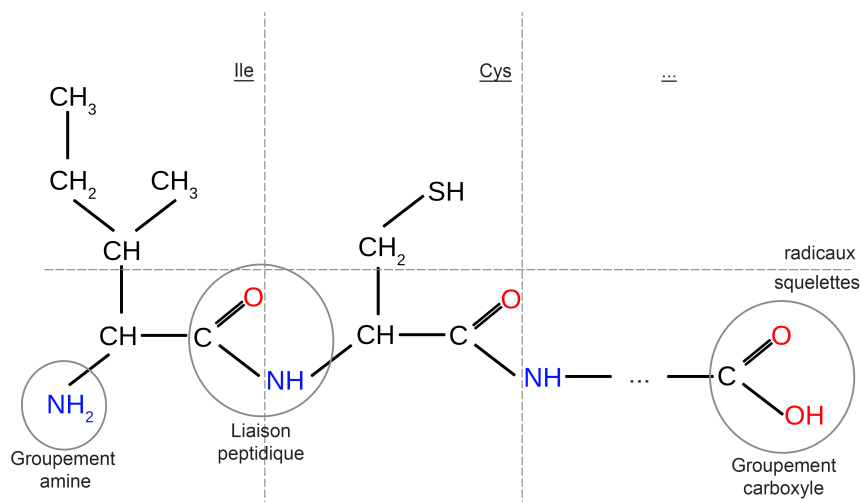
Figure 1.1: Présentation d'une chaîne peptidique. Chaque trait pointillé vertical sépare un acide aminé d'un autre et le trait horizontal sépare le squelette de la chaîne latérale des acides aminés.
