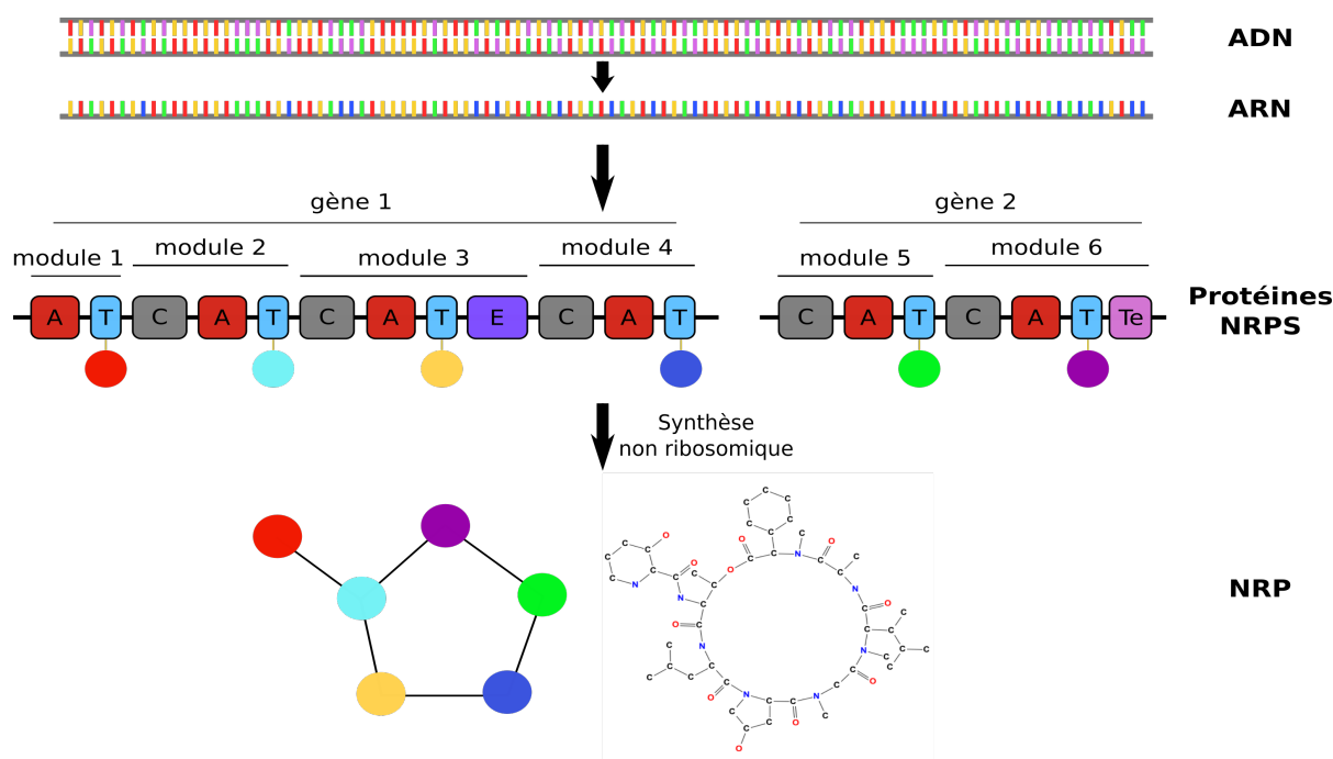
Figure 1.2: Voie de synthèse non ribosomique : groupés en cluster, les gènes codant les protéines NRPS sont transcrits puis traduits par le ribosome. Les domaines A de la NRPS capturent ensuite des monomères (billes de couleur ici) dans l'environnement afin de les assembler en peptide. Enfin, le NRP assemblé est relâché.
