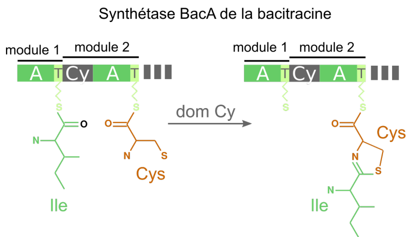
Figure 1.11: Cyclisation entre deux monomères par un domaine Cy
