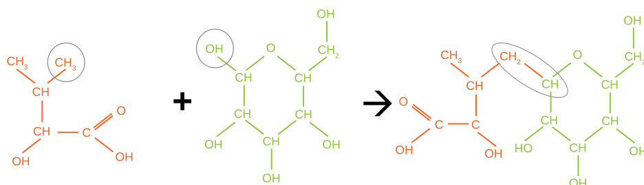
Figure 1.7: Exemple de liaison effectuée avec un sucre
