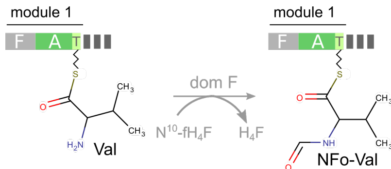
Figure 1.14: Formylation d'un monomère par un domaine F
