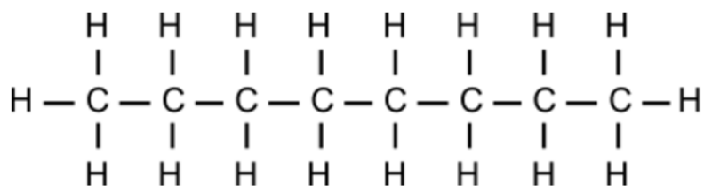
Figure 2: Formule développée de la molécule d'octane.
