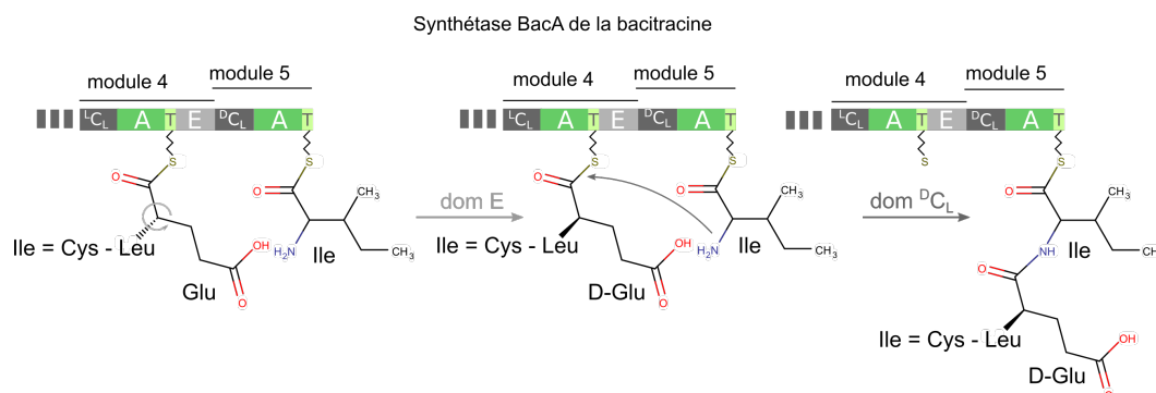
Figure 1.12: Épimérisation d'un monomère par un domaine E
