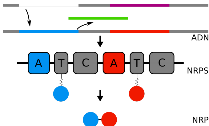
Figure 3.11: La séquence correspondant au domaine A incluant un monomère vert est remplacée par la séquence d'un domaine A correspondant à un monomère bleu. En conséquence, le monomère inclus par la synthétase est bleu.
