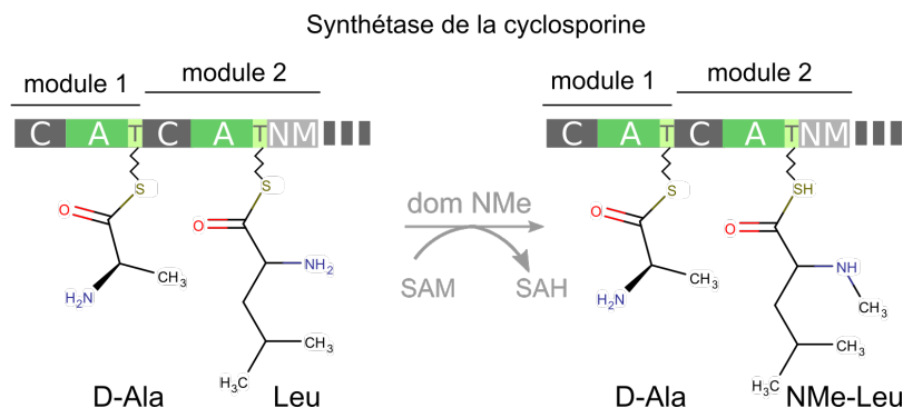
Figure 1.13: Méthylation d'un monomère par un domaine NM
