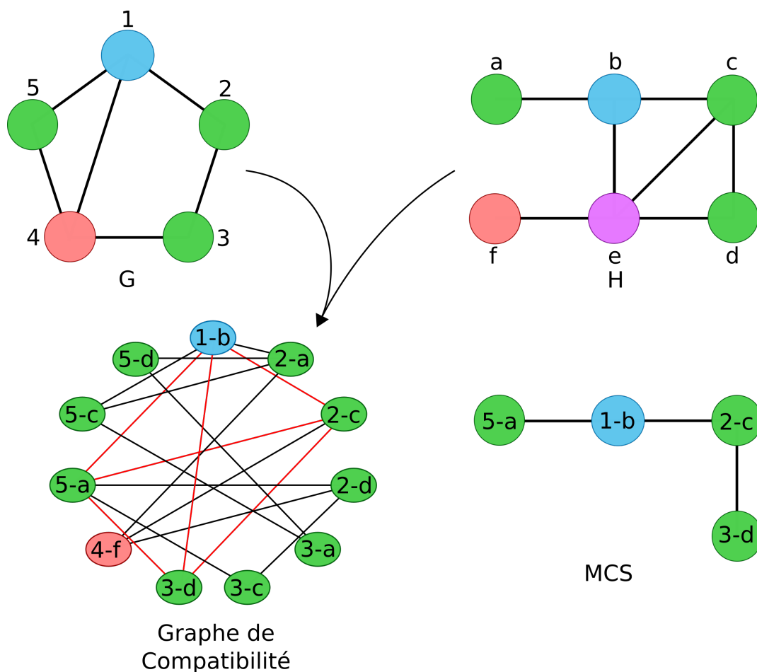
Figure 2.9: Résolution d'un MCS par réduction en clique maximale. Les couleurs représentent les étiquettes des nœuds. Dans le graphe de compatibilité les arêtes rouges identifient la clique maximale détectée.
