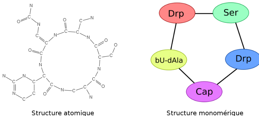
Figure 2.1: Structures atomique et monomérique de la Caprieomycin IIA.
