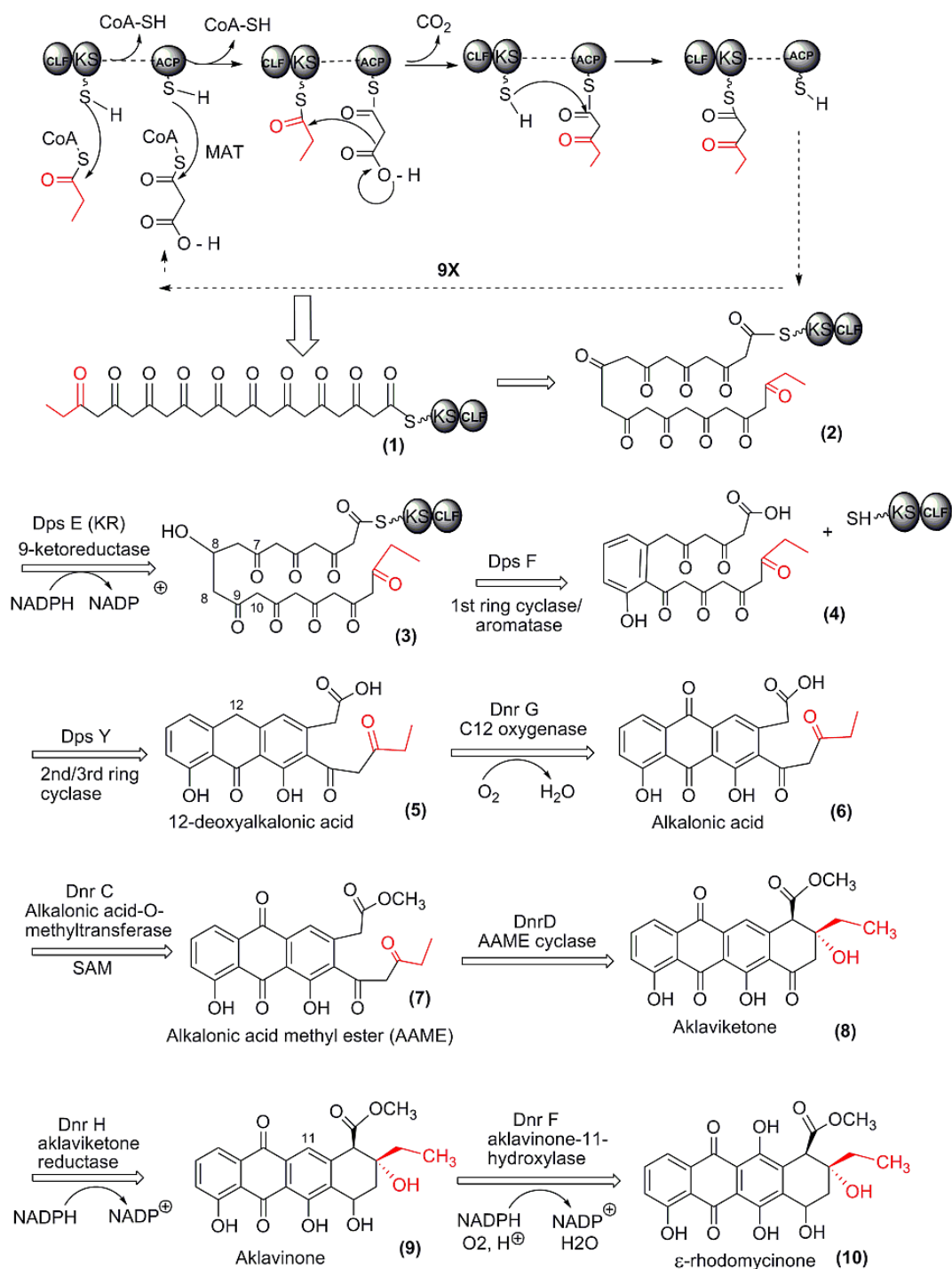
Figure 1.16: Synthèse d'une epsilon-rhodomycinone. Comme pour les NRPS, les PKS sont constitués de modules fonctionnels. Sur cet exemple, on peut voir que certains modules sont utilisés itérativement. La longue chaîne carbonée de la première étape est créée par une utilisation, répétée 9 fois, du même module. Tout comme les NRP, les PK peuvent être modifiés après libération par le PKS (étapes 5 à 10 ici). Source de l'image : en.wikipedia.org/wiki/Polyketide_synthase
