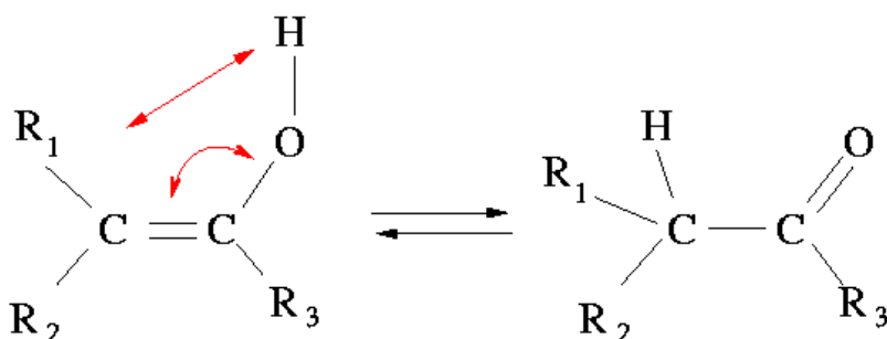
Figure 2.31: Tautomérie d'une molécule
