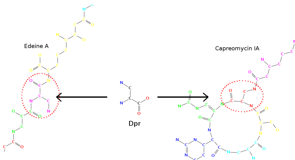
Figure 1.4: Deux exemples d'inclusion du monomère Dpr : Au sein de l'Edeine A, seules deux liaisons classiques du squelette peptidique sont effectuées entre le Dpr (en rose) et les autres monomères. Au sein de la Capreomycin IA, une troisième liaison est effectuée par le Dpr (en rouge) depuis son groupement amine ( NH_2 ) de la chaîne latérale.
