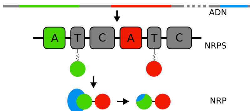
Figure 3.9: Modification post-synthèse du NRP par une action enzymatique. Les gènes NRPS contenant l’encodage des domaines A “vert” et “rouge” sont transcrits puis traduits depuis l’ADN afin de former les NRPS contenant les domaines de même couleur. La NRPS assemble ensuite le peptide. C’est enfin une enzyme ajoutée au cluster de gènes (ici en bleu), qui vient modifier l’un des monomères du NRP.
