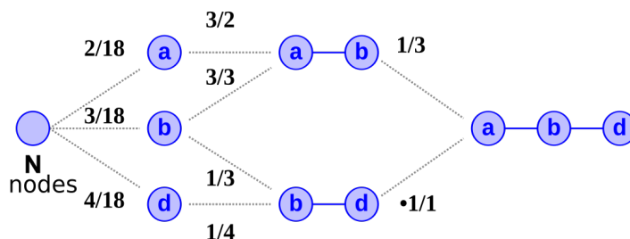
Figure 2.20: Reprise de la base d'apprentissage présentée en figure 2.18 pour définir le filtrage. Les comptages initiaux des fréquences de chacun des nœuds ont été étendus aux comptages de l'ensemble des sous-motifs possibles. Le taux de filtrage d'un ajout de nœud dans un motif est alors défini comme le nombre de détections dans la base du motif étendu divisé par le nombre de détections du motif initial. Ainsi, pour passer d'un motif a à un motif a-b, le taux de filtrage est de 3/2.
