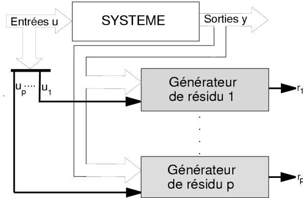
FIG. 4.2: Schéma DRGS relativement aux actionneurs
