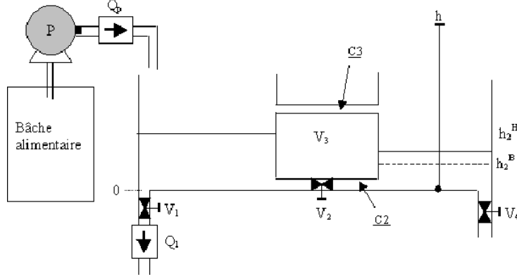
FIG. 6.1: Description du système hydraulique
