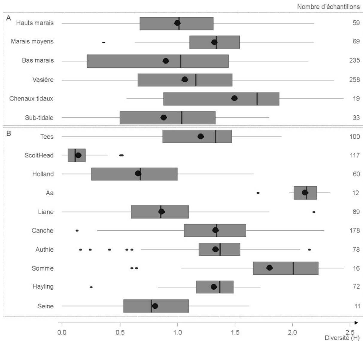
Figure 6 : Boîtes à moustaches montrant la diversité (H' de Shannon) calculé en groupant les échantillons par origine (A) ainsi que les aires d'études estuariennes (B). La ligne noire est la médiane et le cercle noir est la moyenne.
