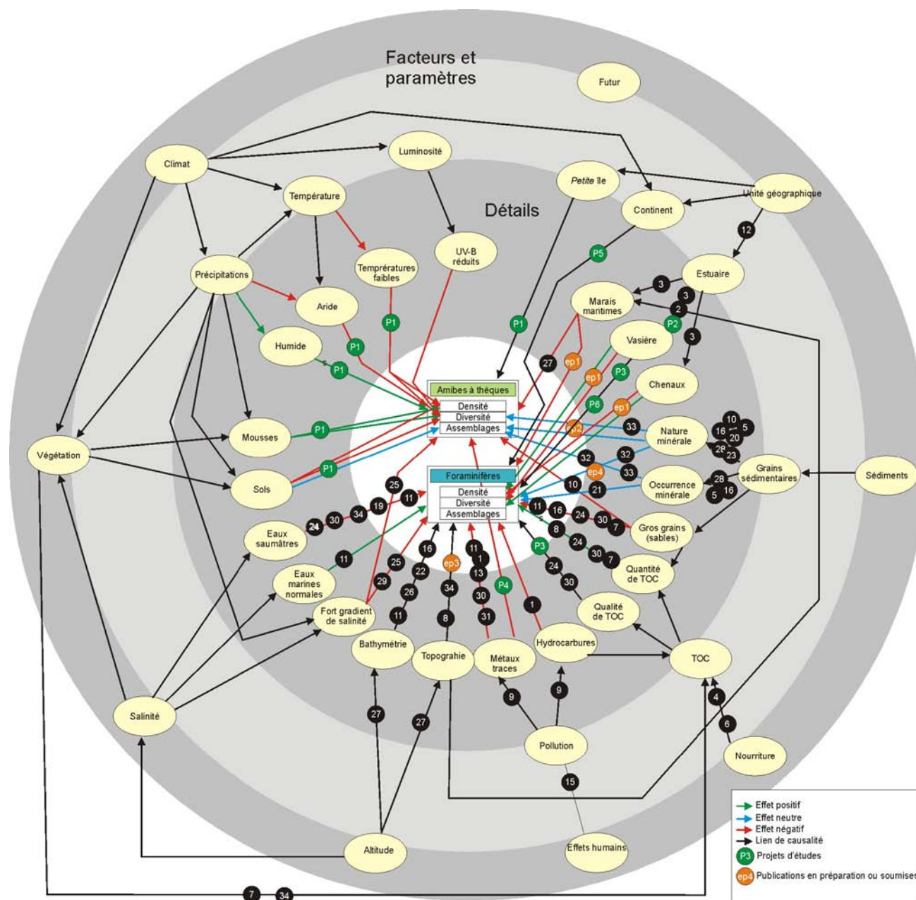
Figure 63 : Nonogramme des pressions des paramètres de l'environnement sur la densité, la diversité et la composition des assemblages de foraminifères benthiques et de thécamoebiens. Les numéros des différents articles étudiant les liens de causalités (cercles noirs) font référence au tableau 1. Les cercles jaunes font référence aux articles en préparation ou soumis, les cercles verts font référence aux projets d'études.
