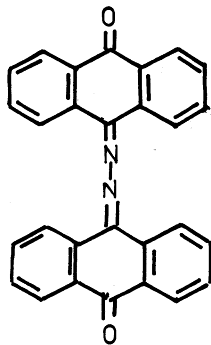
AZINE de l'ANTHRAQUINONE IV
