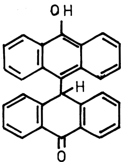
DERIVE DE L'ANTHRANOL
