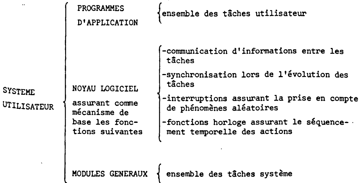
FIG.1 SYSTEME UTILISATEUR
