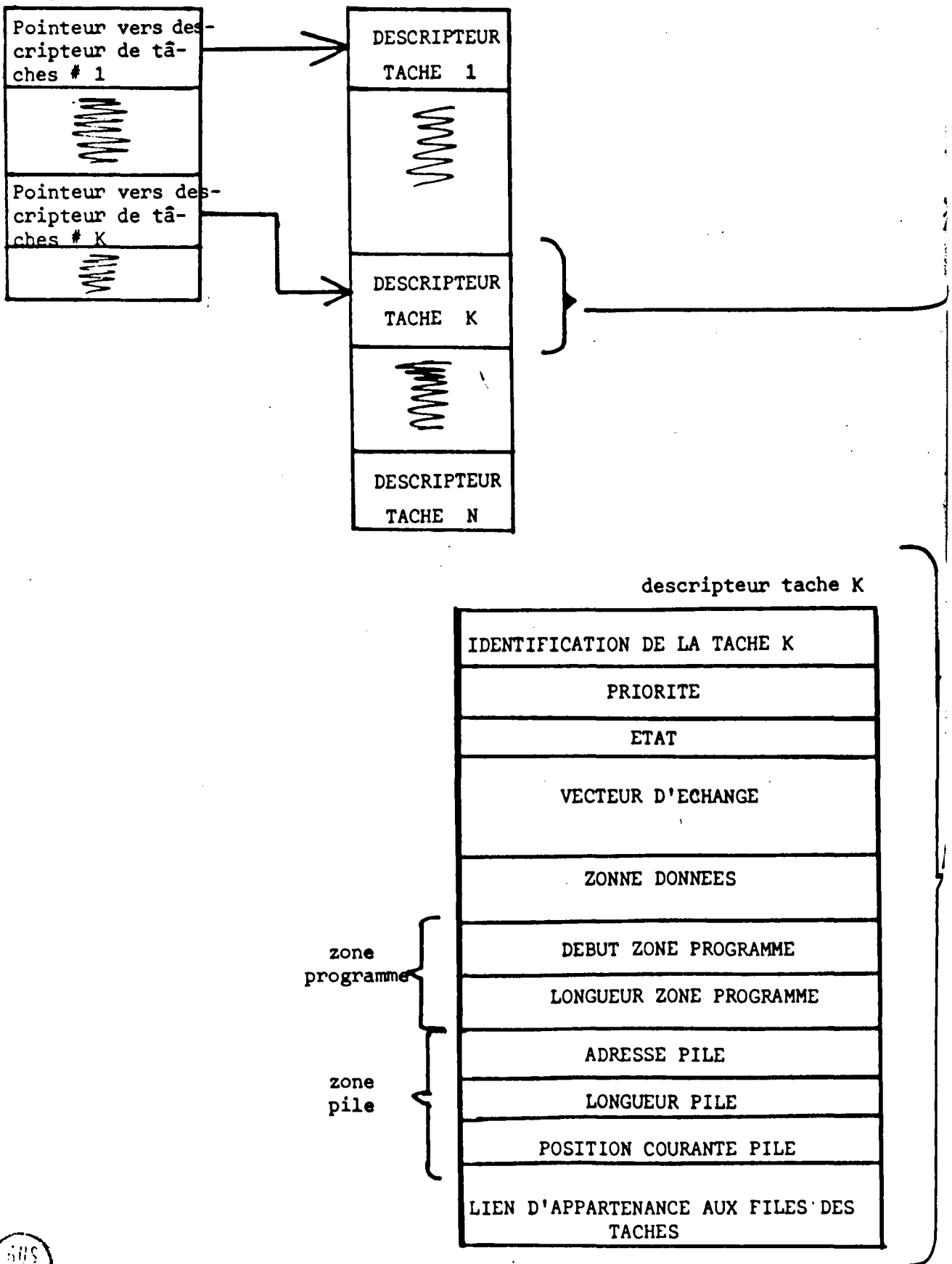
FIG. 7 : DESCRIPTEUR DE TACHES
