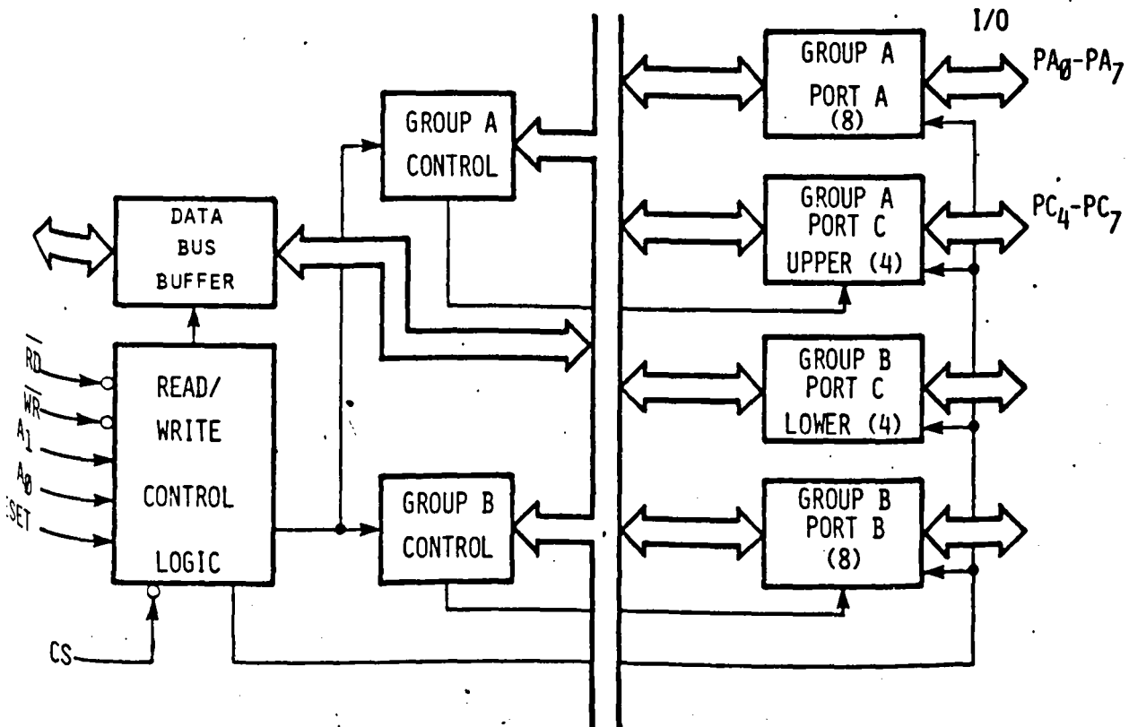
Fig. 2 : Brochage et organisation du coupleur parallèle (PPI) : 8255.
