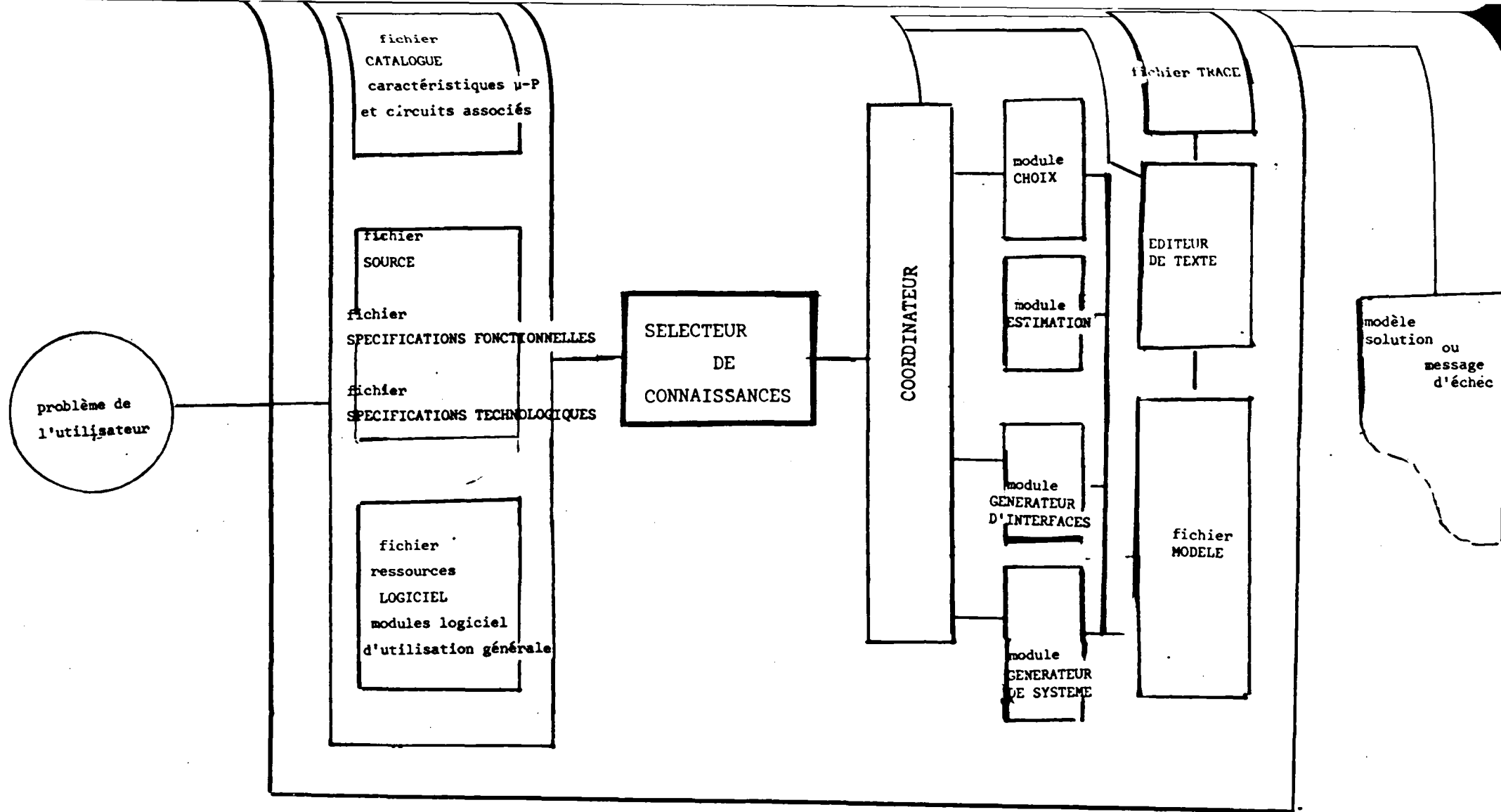
SCHEMA SYNOPTIQUE DE COSMIC.
