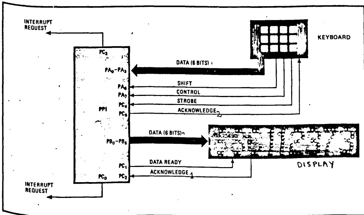
Fig. 3 : Keyboard and display. Exemple de caractérisation des lignes périphériques.
