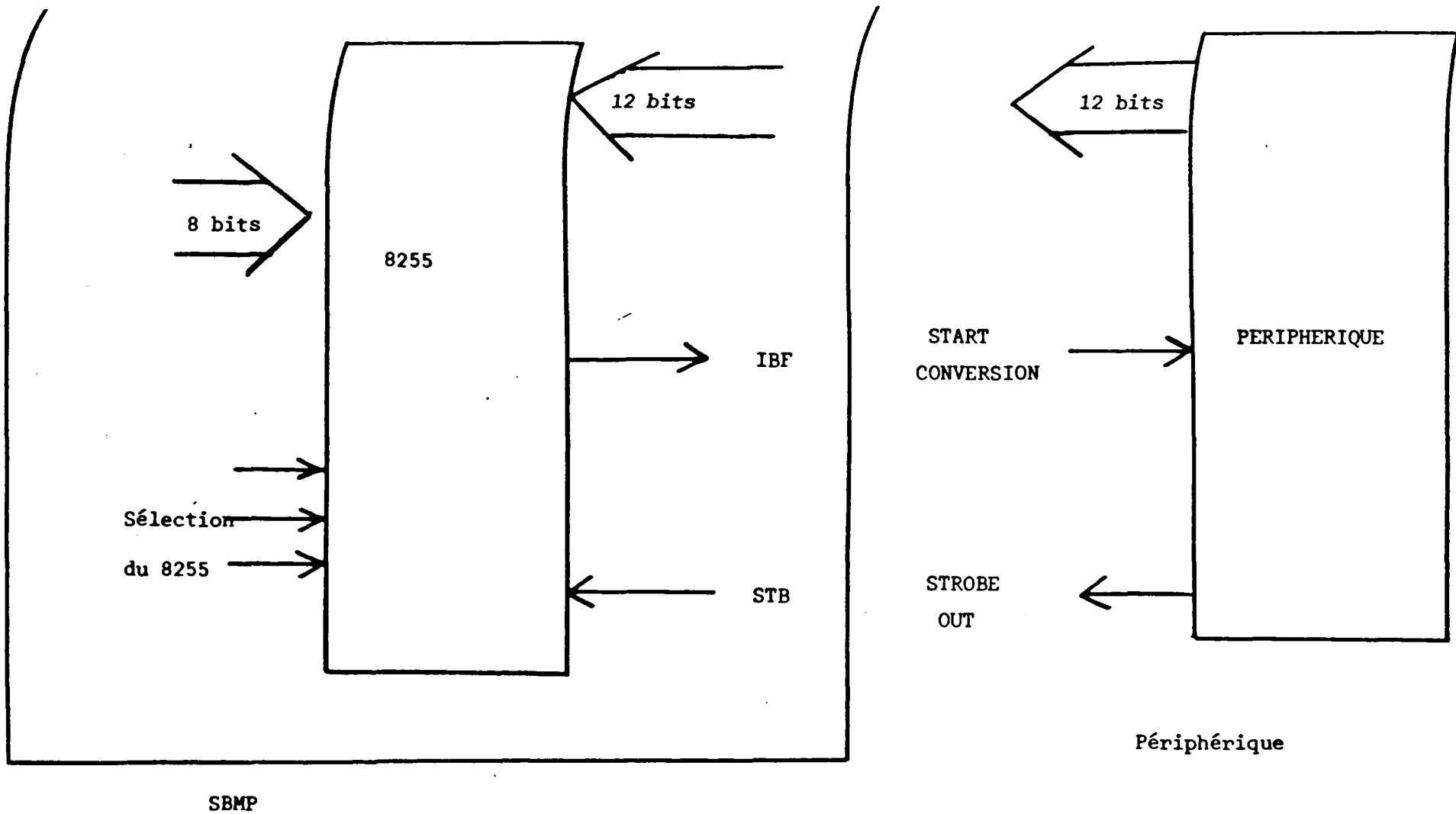
Fig. 7 : Correspondance des lignes d'E/S entre le périphérique et le dispositif d'E/S.
