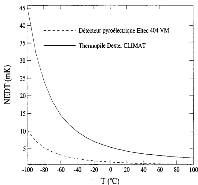
Figure B.1: Comparaison du NEDT de la thermopile du radiomètre CLIMAT et d'un pyroélectrique fabriqué par la société ELTEC, pour un intervalle spectral de 1 \mu\text{m} de largeur centré sur 10 \mu\text{m} , dans lequel l'optique a une transmittance égale à 1 et, pour un champ de 1 millistéradian.
