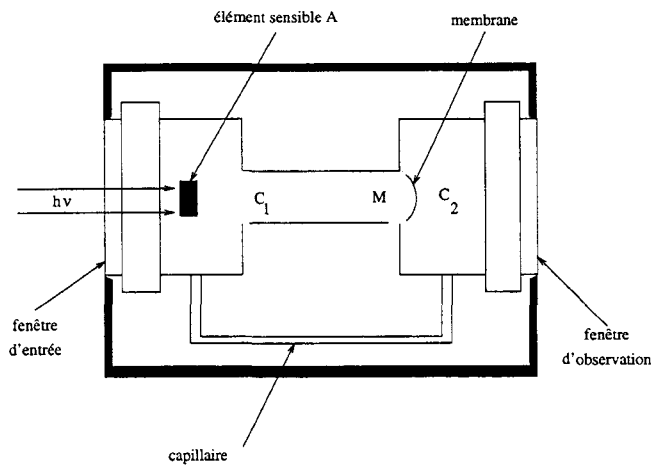
Figure II.8: Principe du détecteur pneumatique [Gaussorgues, 1989].
