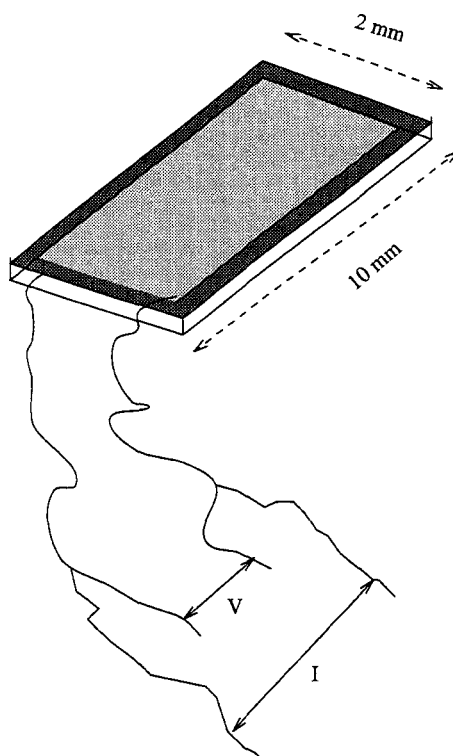
Figure D.1: Schéma d'une sonde en platine.
