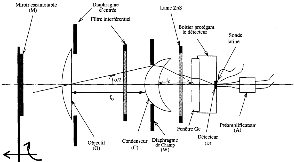
Figure II.16: Schéma synoptique de l'instrument
