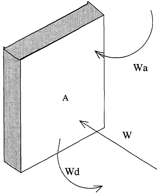
Figure II.2: Représentation des échanges énergétiques sur la surface sensible d'un détecteur thermique [Gaussorgues, 1989]
