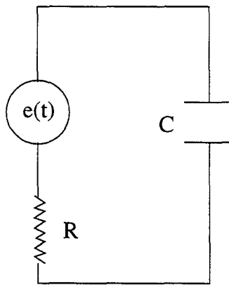
Figure II.5: Circuit équivalent au générateur de bruit Johnson [Lenoble , 1993]
