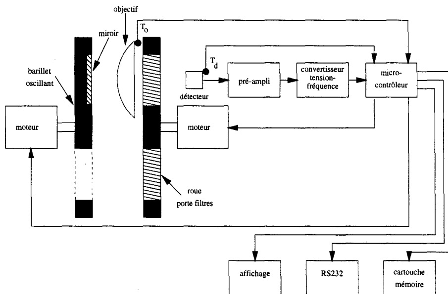
Figure II.17: Schéma de l'électronique montée sur l'instrument.
