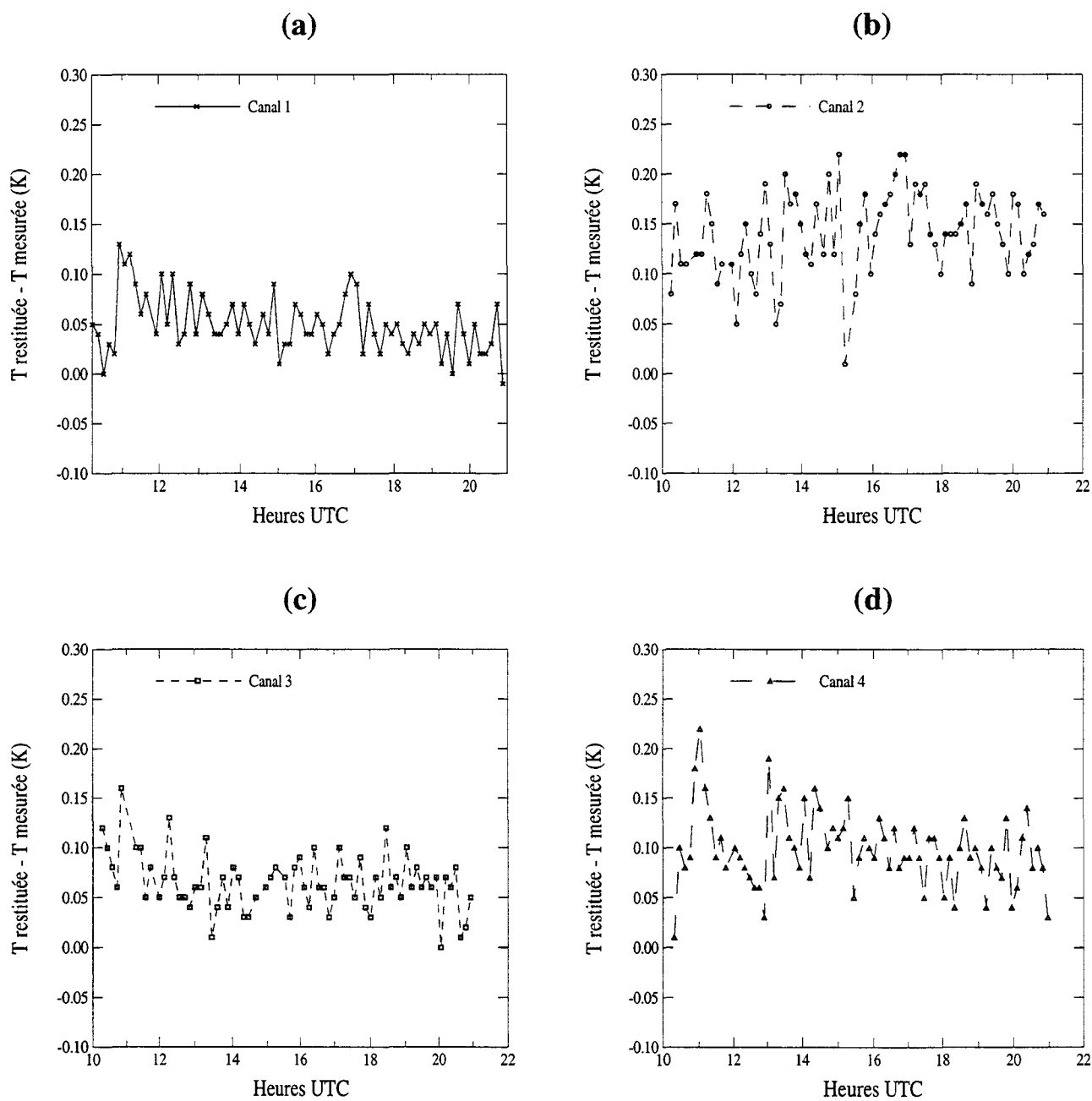
Figure III.12: Différences entre la température du corps noir restituée et mesurée dans les quatre canaux. (a): [8,14\mu\text{m}] , (b): [11.5,12.5\mu\text{m}] , (c): [10.5,11.5\mu\text{m}] , (d): [8.2,9.2\mu\text{m}] .
