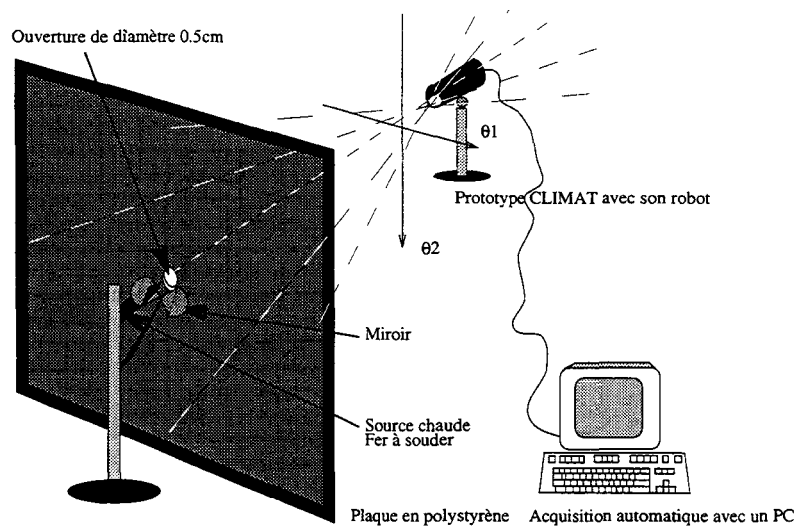
Figure III.1: Dispositif expérimental dédié à la mesure du champ de visée du prototype CLIMAT. Pour chaque visée repérée par (\theta_1, \theta_2) , le radiomètre mesure dans le canal large la luminance émise par une source chaude. La contribution de la plaque est éliminée en effectuant une mesure lorsque l'ouverture est occultée par le miroir.
