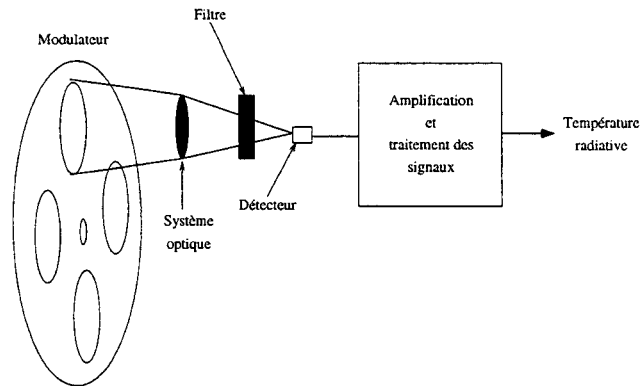
Figure I.2: Schéma synoptique d'un radiothermomètre ou d'un radiomètre à modulation.
