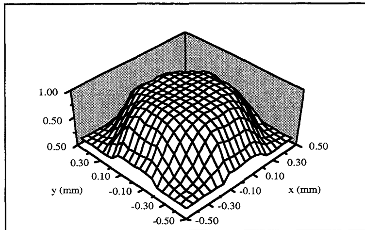
Figure II.15: Simulation de Monte Carlo sur le prototype du radiomètre CLIMAT d'après M.Haeffelin: densité d'énergie normalisée incidente sur le détecteur centré sur l'axe optique du système
