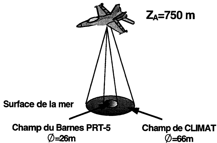
Figure IV.9: Configuration en vol des radiomètres CLIMAT et Barnes
