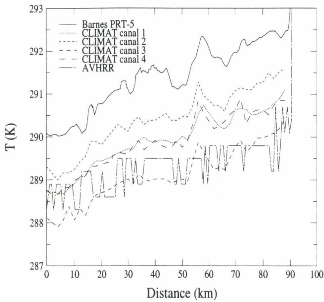
Figure IV.12: Températures de brillance de la mer le long de l'axe Calais–Dieppe mesurées par les radiomètres Barnes et CLIMAT comparées à la température de la mer restituée par l'algorithme "split–window" appliqué aux données du capteur satellitaire AVHRR.
