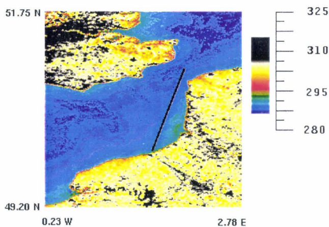
Figure IV.11: Températures de la mer obtenues à partir des mesures dans les canaux 4 et 5 du capteur AVHRR par application de l'algorithme "split-window". Les données ont été fournies par P. Leborgne du Centre de Météorologie Spatiale de Lannion
