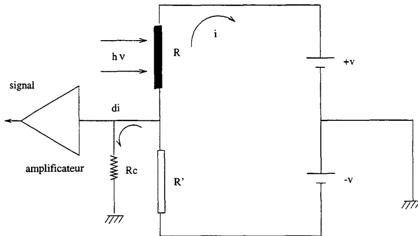
Figure II.7: Principe du bolomètre [Gaussorgues, 1989].
