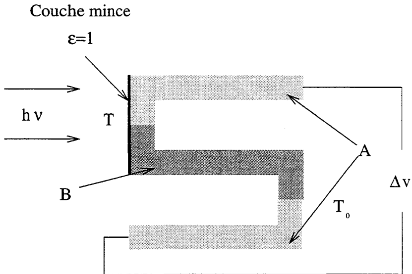
Figure II.10: Principe du détecteur à thermocouple [Lenoble , 1993].
