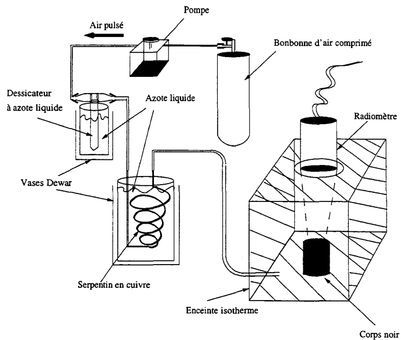
Figure III.8: Dispositif expérimental utilisé pour l'étalonnage du radiomètre.
