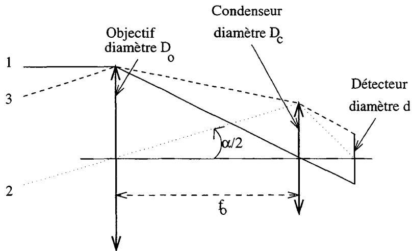
Figure II.11: Dispositif de Köhler pour un champ de demi-ouverture \alpha/2
