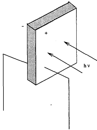
Figure II.9: Principe du détecteur pyroélectrique [Gaussorgues, 1989].
