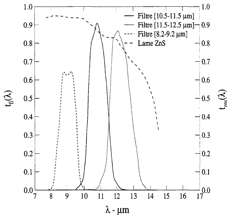
Figure III.4: Transmittances spectrales moyennées du jeu de de la même série que celui qui équipe le prototype: a: [11.5,12.5μm], b: [10.5,11.5μm], c: [8.2,9.2μm], d: lame ZnS.
