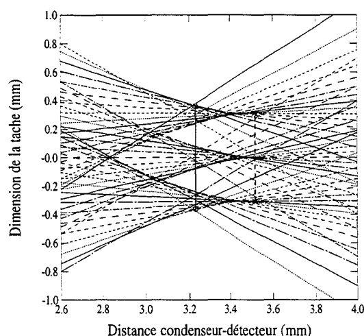
Figure II.12: Résultat du tracé de rayons pour l'option 3: Les rayons proviennent de des deux extrémités et du centre de l'objectif, pour lesquels nous avons fait varier l'angle de lancer. Le trait pointillé vertical définit la dimension de l'image paraxiale dans les conditions de Gauss et, le trait plein définit la dimension de la tache de moindre diffusion, hors conditions de Gauss
