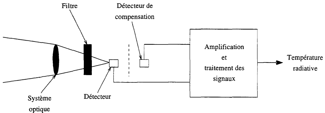
Figure I.1: Schéma synoptique d'un radiomètre statique.
