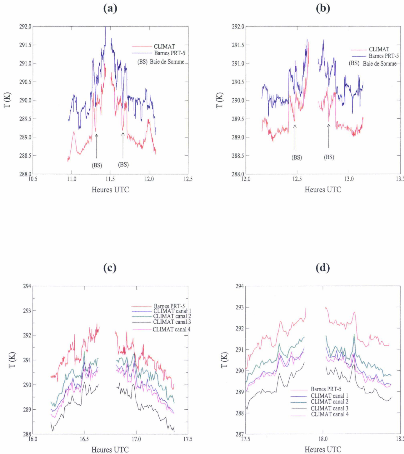
Figure IV.10: Résultats de la campagne de mesures aéroportées. Températures de brillance de la mer mesurées avec les radiomètres Barnes et CLIMAT. Chaque graphe correspond à un aller retour entre Calais et Dieppe, à une altitude donnée: (a): Canal large, Z_A = 750m , (b): Canal large, Z_A = 600m , (c): 4 canaux, Z_A = 750m , (d): 4 canaux, Z_A = 600m .
