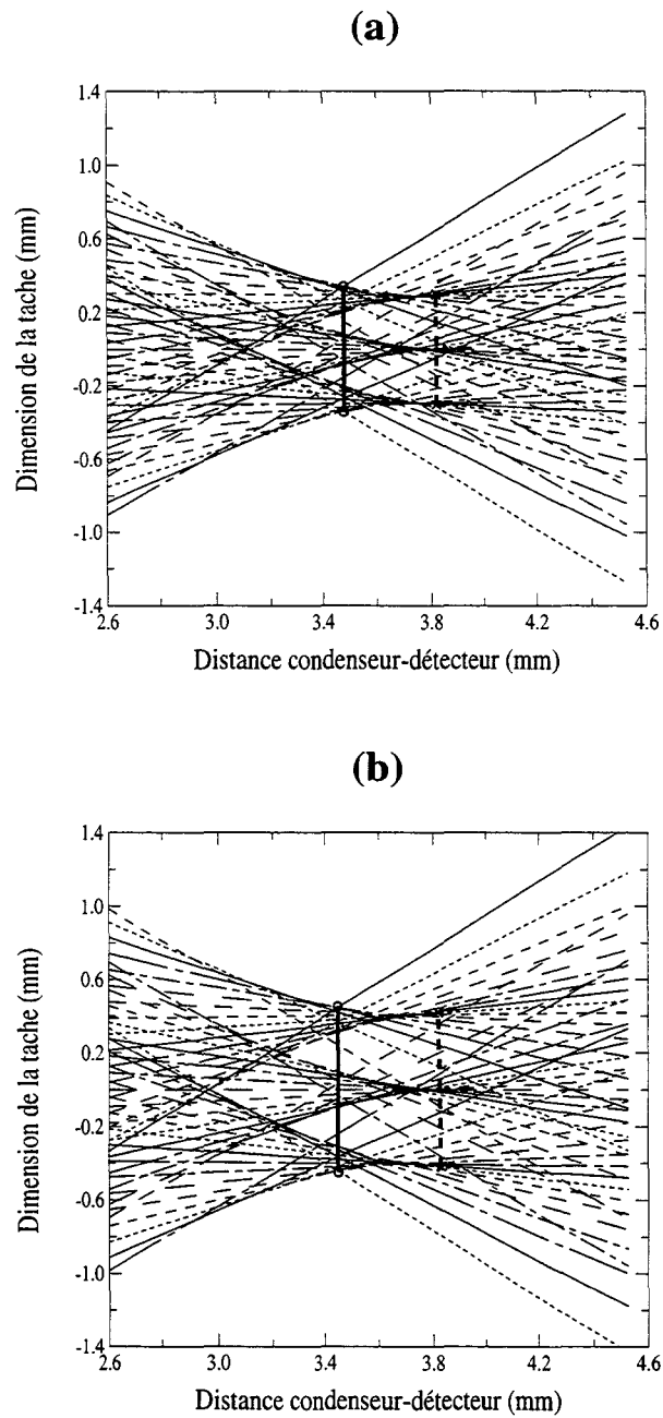
Figure II.13: Résultat du tracé de rayons pour le prototype du radiomètre CLIMAT: la figure (a) correspond à un diamètre utile de l'objectif de 4mm et la figure (b) correspond à un diamètre utile de 5.6 mm
