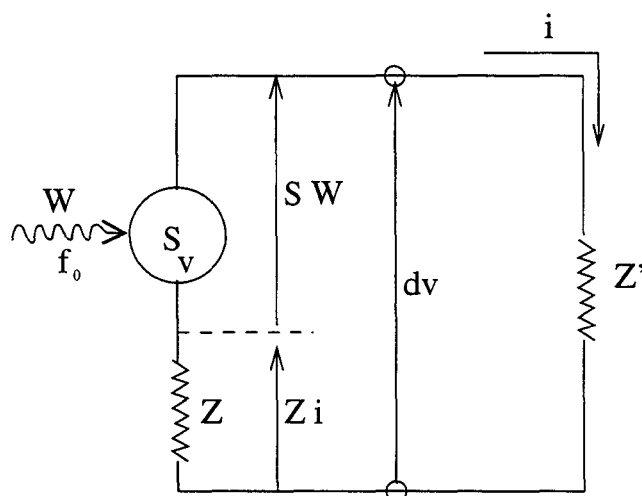
Figure II.3: Circuit équivalent impédance du détecteur [Gaussorgues, 1989]
