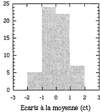
Figure III.14: : Mesure du bruit expérimental du prototype CLIMAT: Ecart à la moyenne du signal mesuré par CLIMAT, placé devant un corps noir, dans une enceinte thermostatée à 20°C
