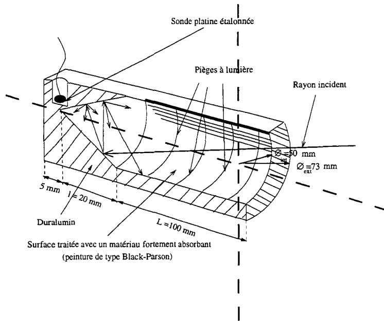
Figure III.7: Vue en coupe du corps noir utilisé pour l'étalonnage.
