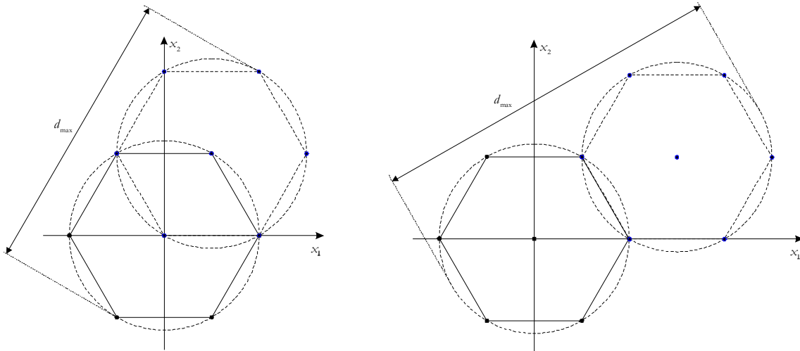
Figure 15 - Dimensions maximales de cellules suivant les 2 modes considérés pour les plans de Doehlert de type D-1 Mode 1 ( gauche ) – Mode 2 ( droite )
