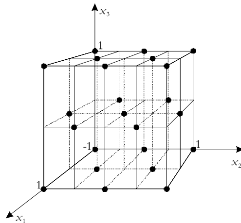
Plan treillis ( k=3 ) avec N_{n_1}=3, N_{n_2}=5, N_{n_3}=3 générateurs utilisés : I=-abc - (N=23)
