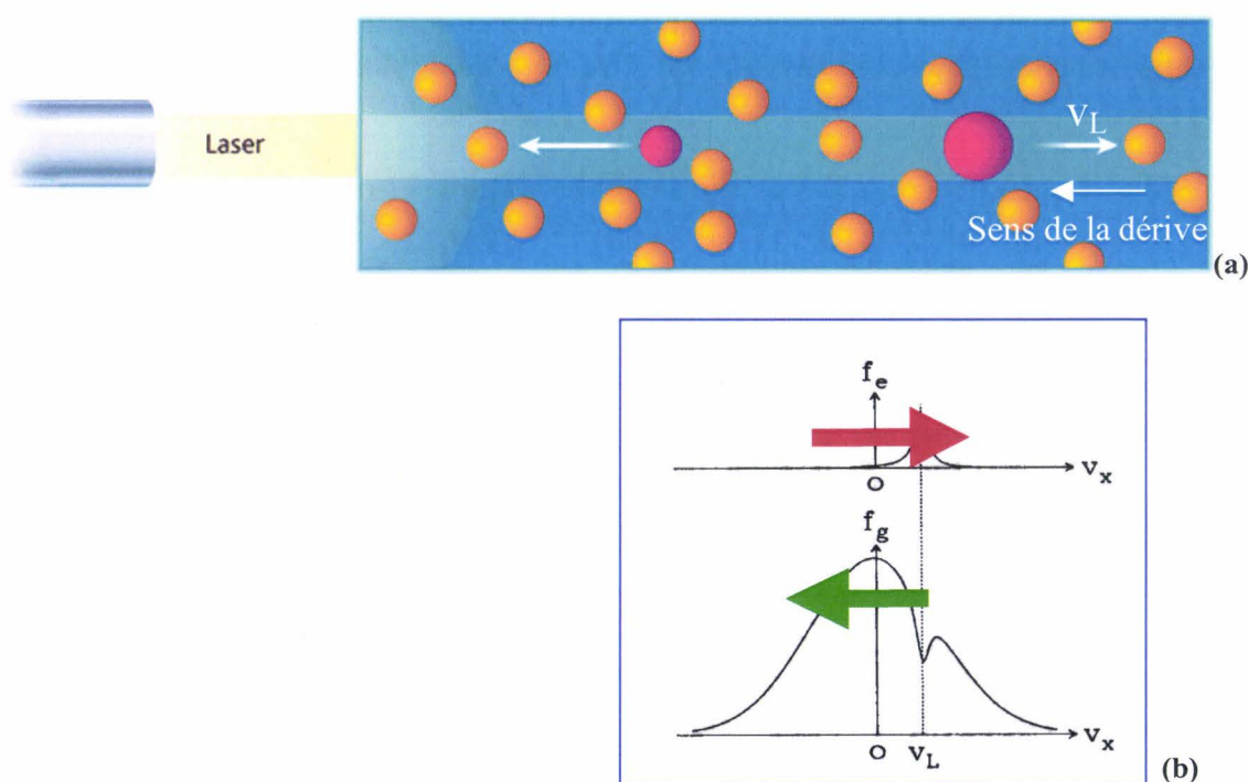
Figure III. 3. (a) Dérive induite par laser [Hou,2005] ; (b) Classes de vitesse
