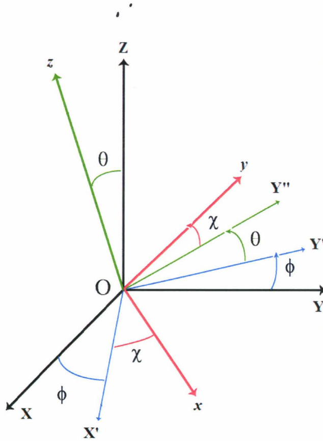
Figure I. 4. Les angles d'Euler
