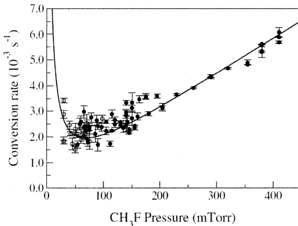
Figure IV. 11. Taux de conversion en fonction de la pression pour les cellules en verre
