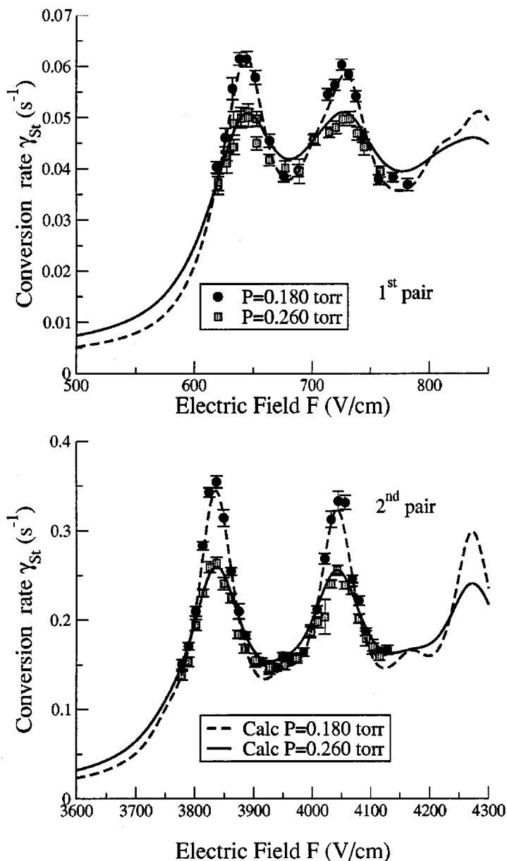
Figure II. 11. «Spectre de conversion» pour les deux premiers croisements pour deux valeurs de pression: 180 mTorr et 260 mTorr.
