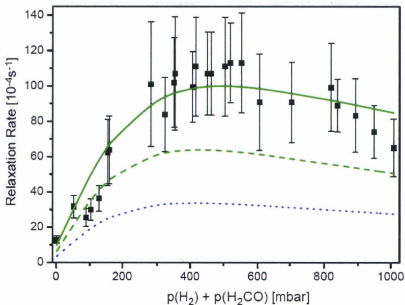
Figure II. 4. Taux de conversion en fonction de la pression pour \text{H}_2\text{CO} en présence de \text{H}_2 [Bec] Courbe en trait plein: calcul avec les paramètres de Curl et al. [Cur] Courbe en pointillée: calcul avec les paramètres de Chapovsky [Cha, 2001]
