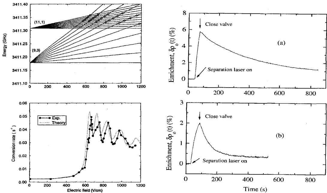
Figure II. 8. Mesures du taux de conversion en champ électrique de ^{13}\text{CH}_3\text{F}
