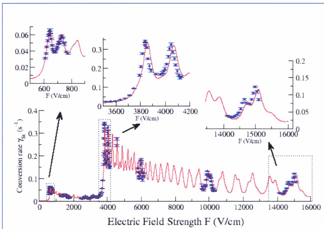
Figure II. 12. «Spectre de conversion»
