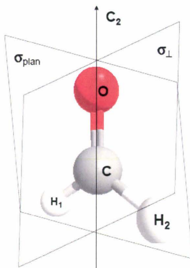
Figure I. 3. Le groupe ponctuel de H 2 CO
