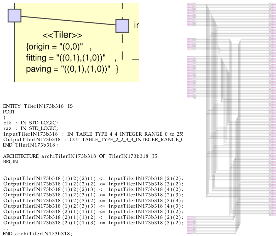
FIG. 5.11: La partie en haut à gauche représente l'expression des dépendances de données exprimées en ARRAY-OL, la partie en bas à gauche représente le code VHDL généré du comptant tiler et la droite de la figure le résultat de synthèse sous Quartus de ce composant. Les connecteurs sont bien visibles.
