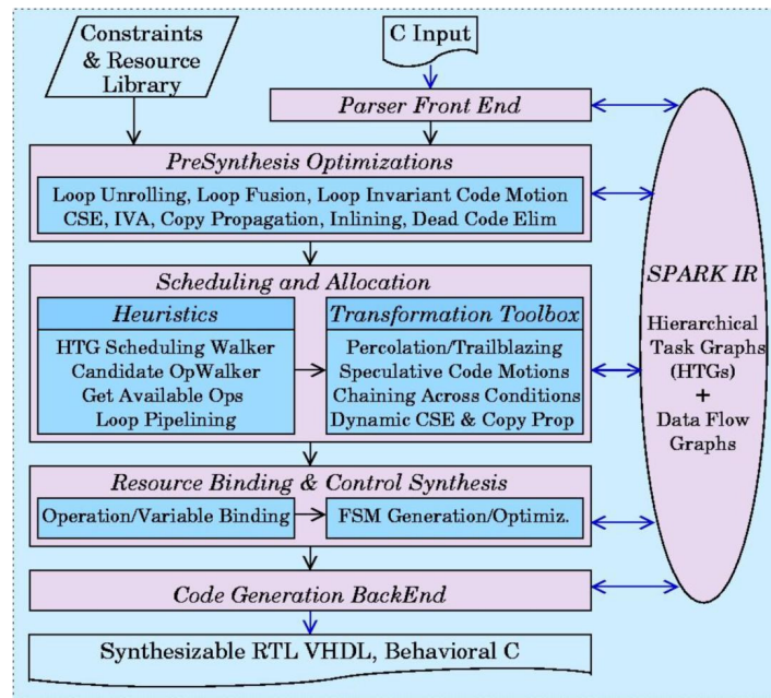
FIG. 1.7: Le flot de conception dans SPARK [122].
