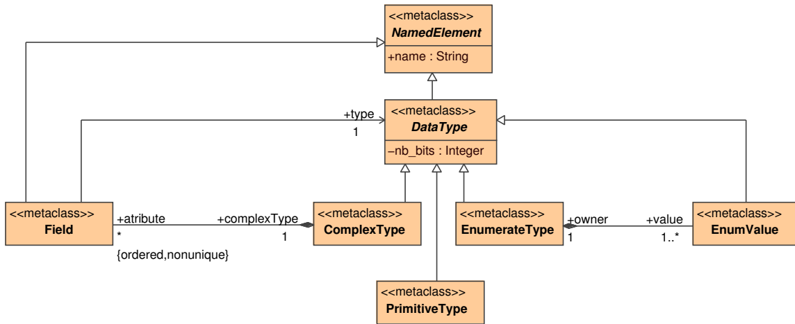
FIG. 3.14: Métamodélisation des types de données utilisée dans les différents métamodèle de l’environnement Gaspard et par conséquent pour les types de données du métamodèle RTL.
