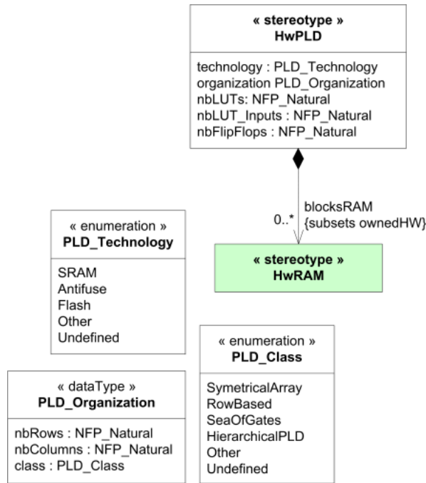
FIG. 1.17: Partie du profil MARTE [101] représentant la modélisation des FPGAs.
